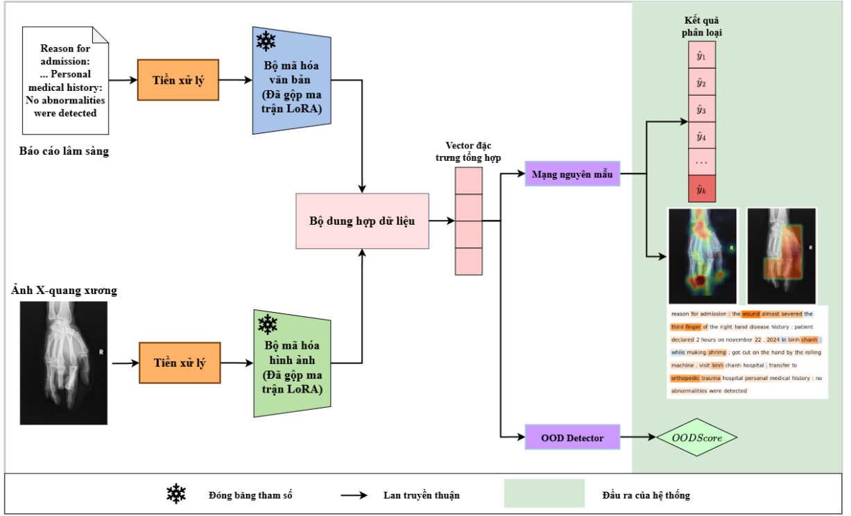
Hình 3.7: Quy trình suy luận trực tuyến và phát hiện mẫu ngoại phân phối
