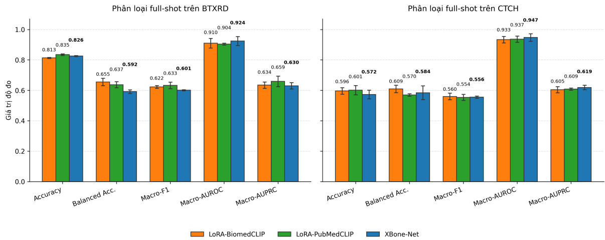
Hình 4.2: Đối sánh năm độ đo full-shot giữa XBone-Net và hai mô hình cơ sở chỉnh hiệu quả tham số gần nhất
