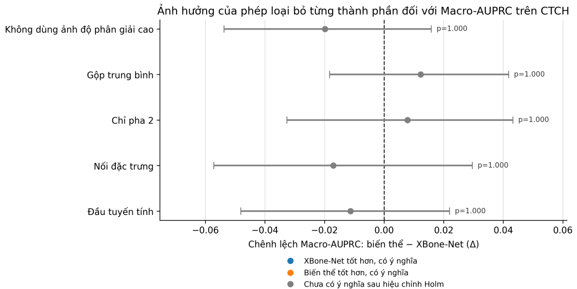
Hình B.6: Khoảng tin cậy 95% của chênh lệch Macro-AP giữa từng biến thể loại bỏ thành phần và XBone-Net trên CTCH
