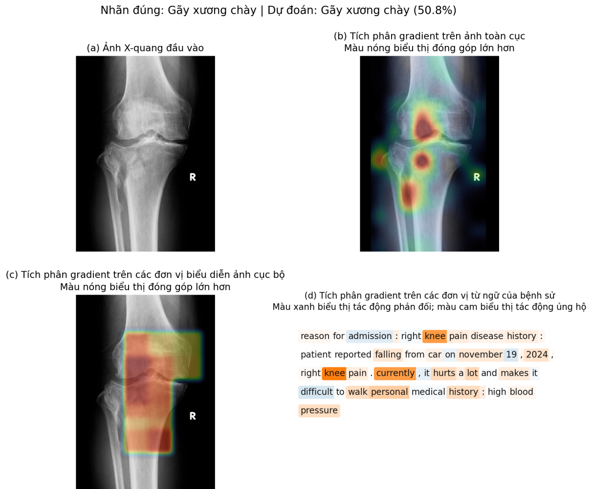
Hình 4.13: Phân tích tích phân gradient của một trường hợp dự đoán đúng gãy xương chày trên CTCH
