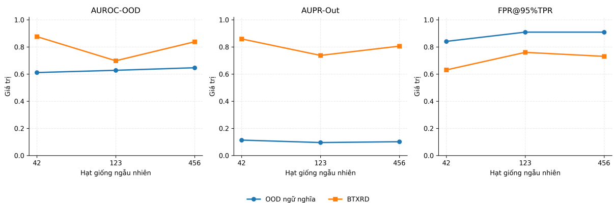
Hình B.7: Các độ đo OOD của phương pháp Mahalanobis theo tâm lớp tại từng hạt giống trên kịch bản OOD ngữ nghĩa và BTXRD
