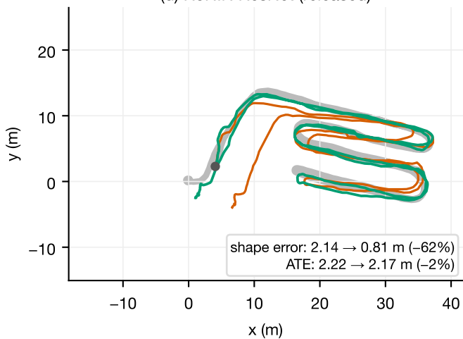
(d) RoNIN ResNet (released)
