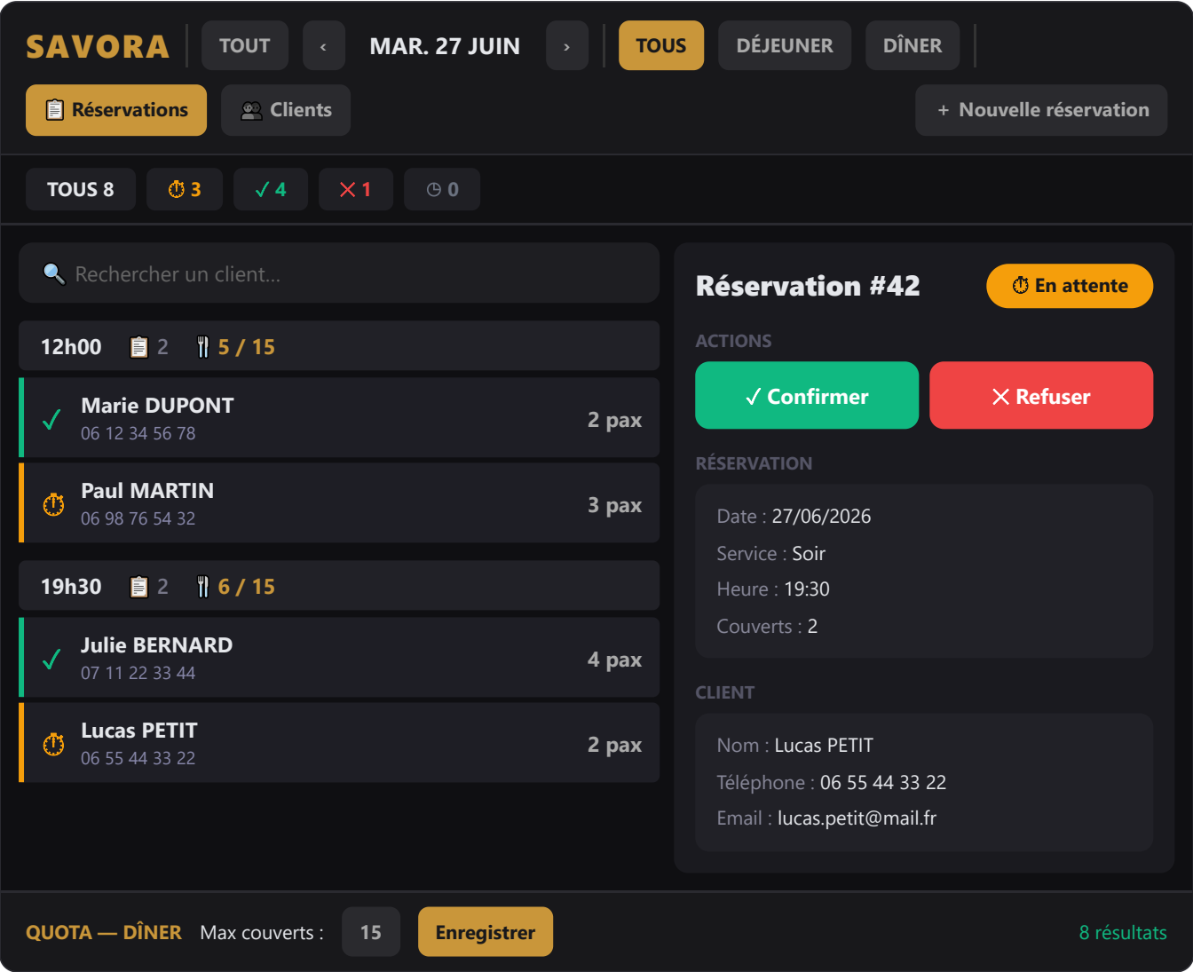
Figure 1 — Écran principal : navigation par date, filtres par service et statut, planning groupé par créneau, panneau de détail avec actions, barre de quota.
