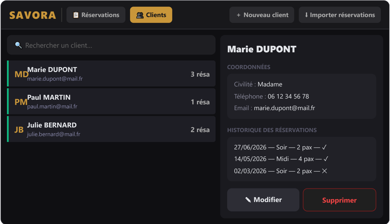
Figure 2 — Gestion des clients : liste avec recherche et compteur de réservations, fiche détaillée éditable, historique, actions CRUD.
