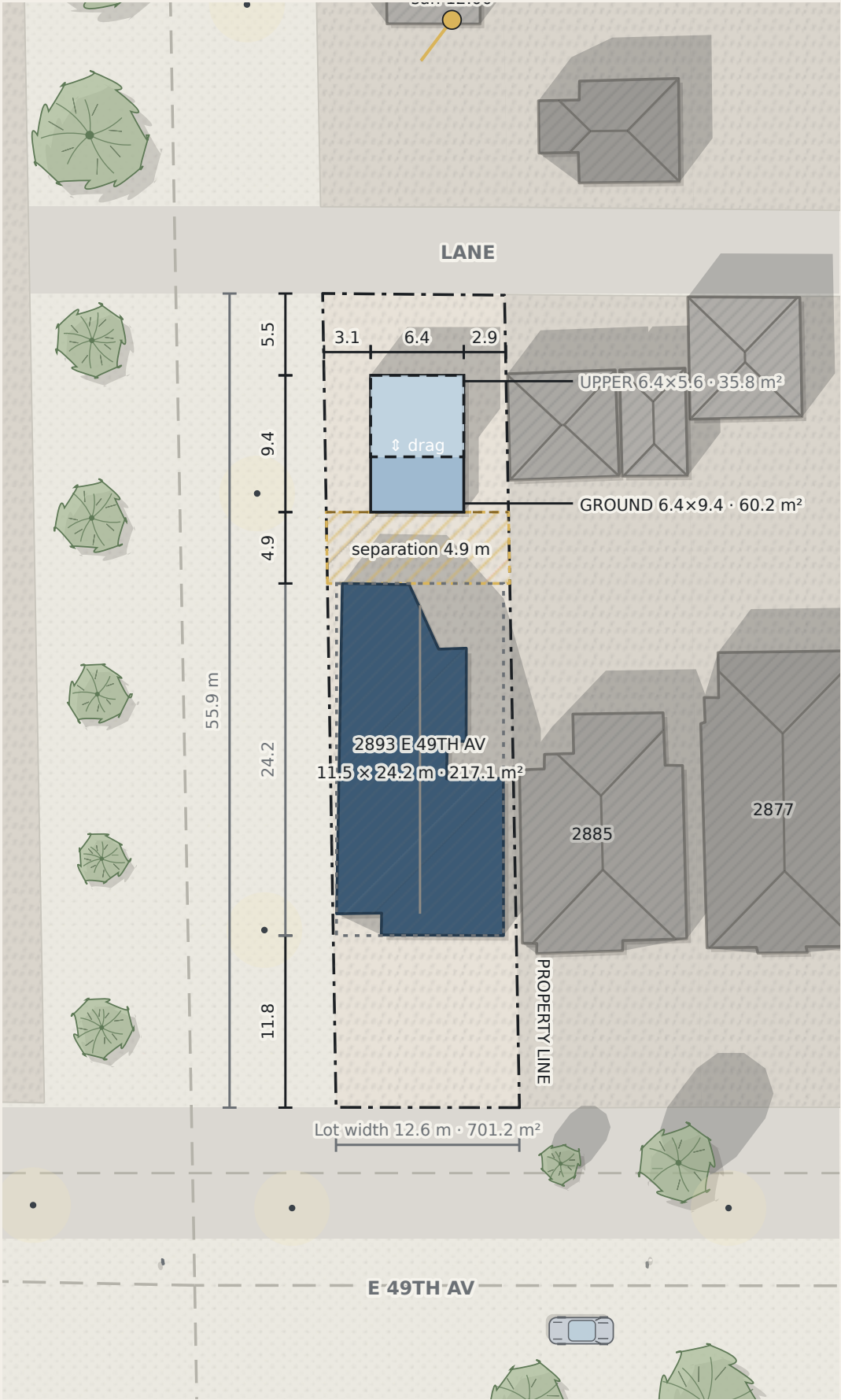
Site plan 2893 E 49TH AV · laneway house · setbacks in m 0 5 m N
