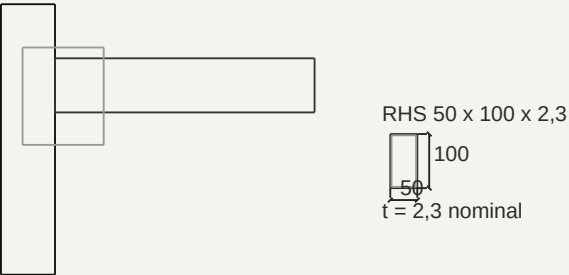
D1 / BALOK-KOLOM
