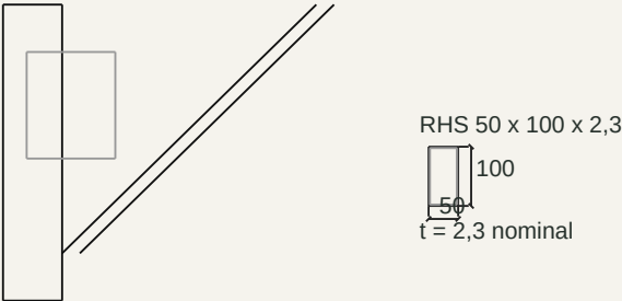
D2 / X-KOLOM
