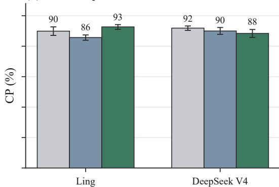
(b) Ordered-path CP
