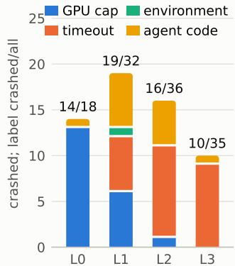
(d) Crashes
