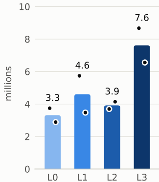
(b) Tokens/run, L3/L0 2.30×
