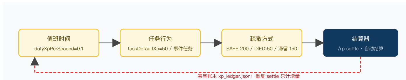
图 3 · 经验三来源 → 增量结算 → 等级 (LevelCurve: xpForLevel(n)=base \cdot n^{pow} , 默认 base=100, pow=2 )
