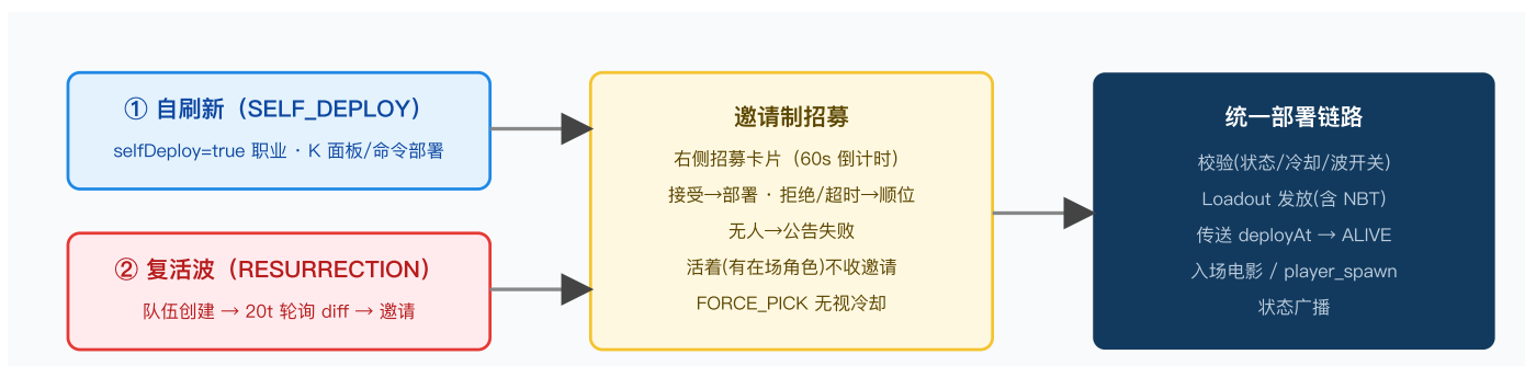
图 4 · 三条刷新通道汇入统一部署链路
