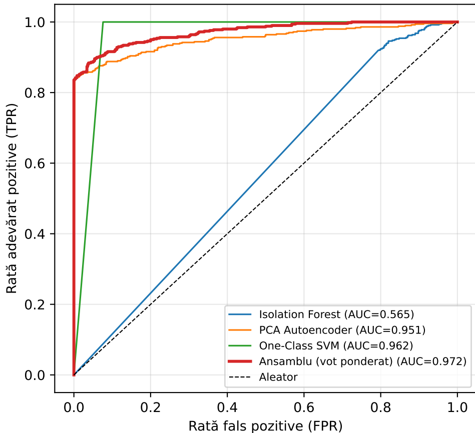
Curbe ROC — modele individuale vs. ansamblu
