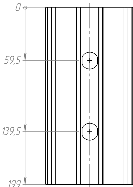
Рис. 6 195.003-04 (1600A) остальное см. рис. 1
