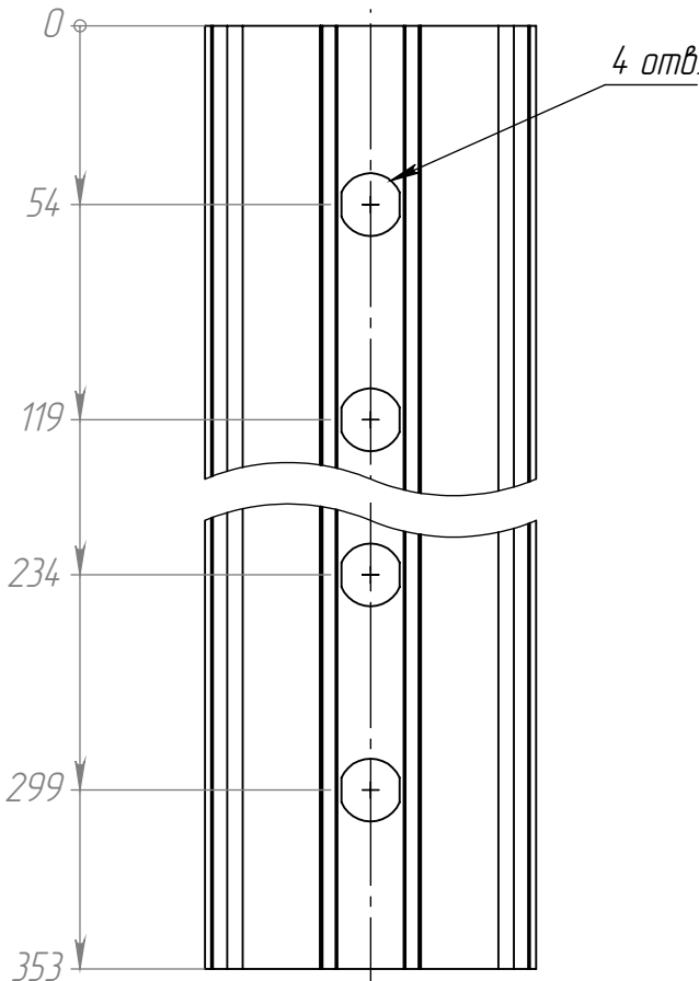
Рис. 8 195.003-06 (2500A) остальное см. рис. 1
