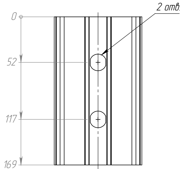
Рис. 5 195.003-03 (1250A) остальное см. рис. 1
