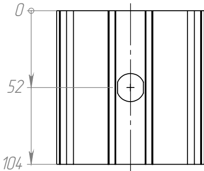
Рис. 3 195.003-01 (800A) остальное см. рис. 1
