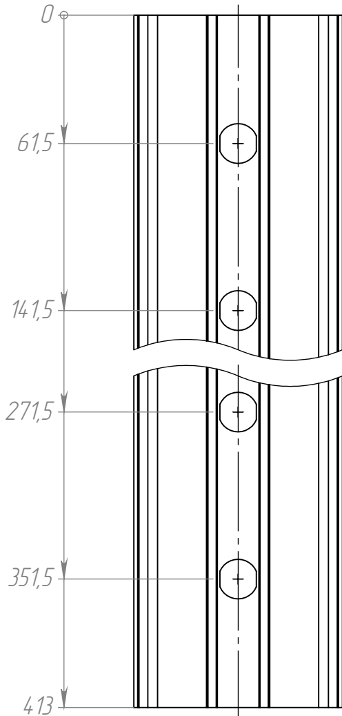
Рис. 9 195.003-07 (3200A) остальное см. рис. 1
