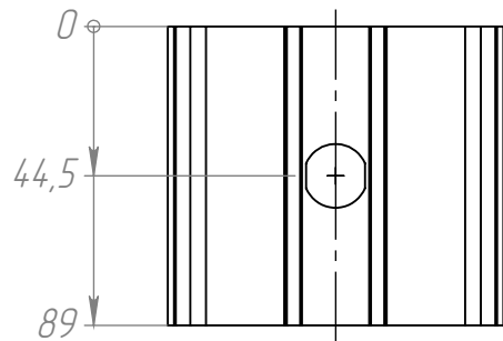
Рис. 2 195.003 (630A) остальное см. рис. 1
