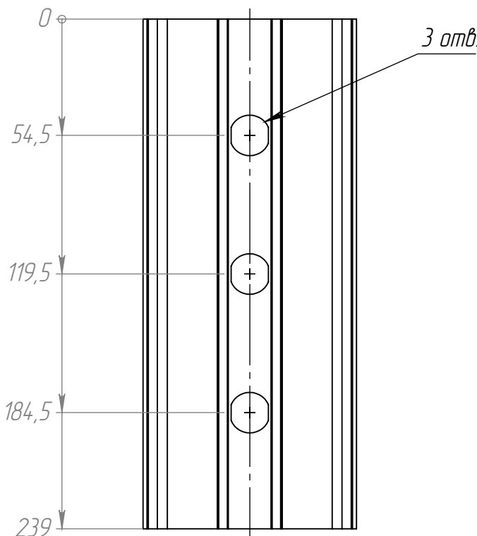
Рис. 7 195.003-05 (2000A) остальное см. рис. 1
