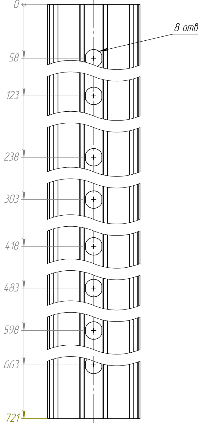
Рис. 11 195.003-09 (5000A) остальное см. рис. 1
