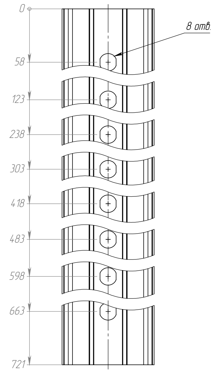
Рис.11 195.004-09 (5000A) остальное см. рис. 1
