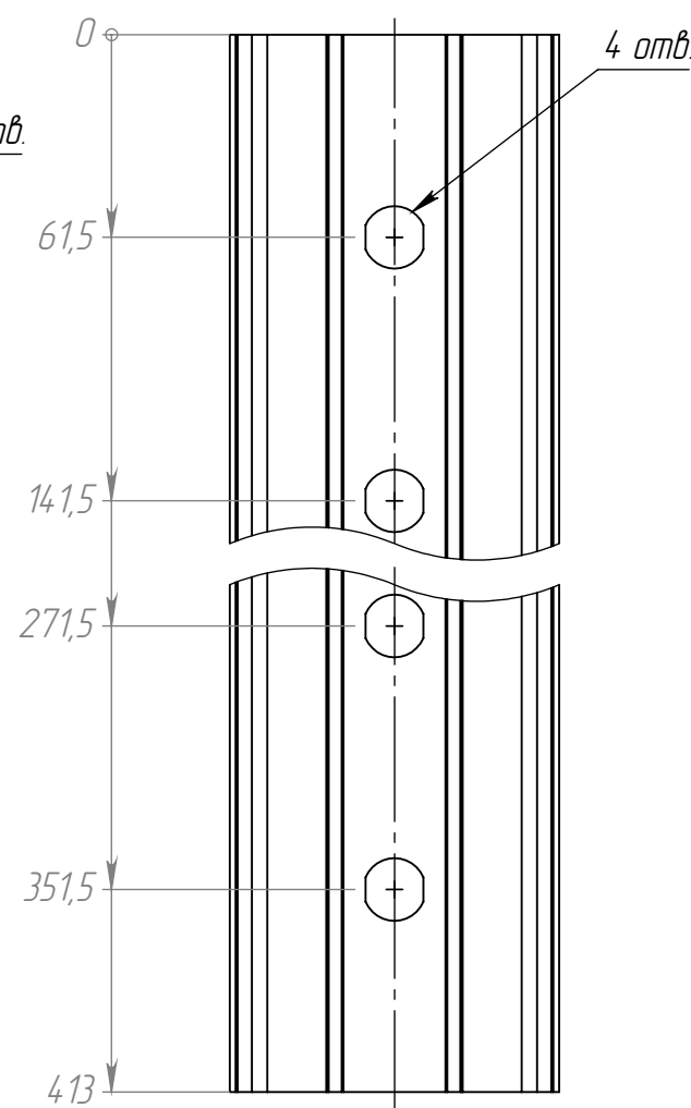
Рис.9 195.004-07 (3200A) остальное см.рис. 1
