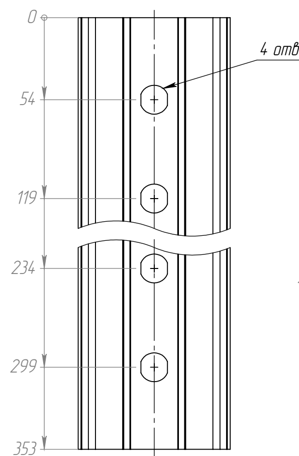
Рис.8: 195.004-06 (2500A) остальное см.рис. 1
