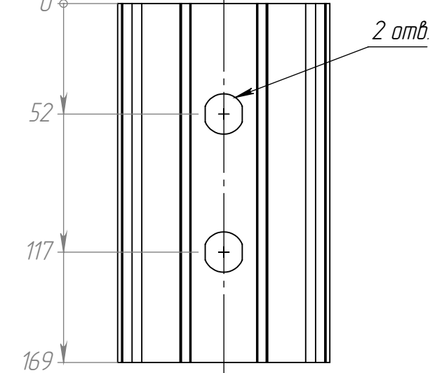
Рис.5 195.004-03 (1250A) остальное см. рис. 1
