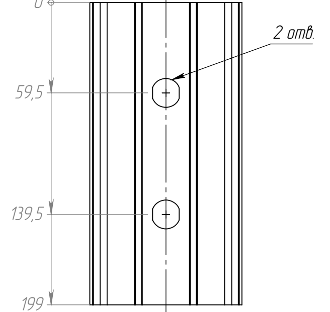
Рис.6: 195.004-04 (1600A) остальное см. рис. 1
