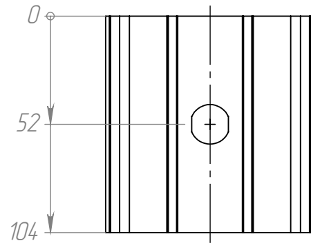
Рис.3 195.004-01 (800A) остальное см. рис. 1
