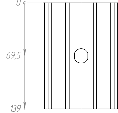
Рис.4 195.004-02 (1000A) остальное см. рис. 1
