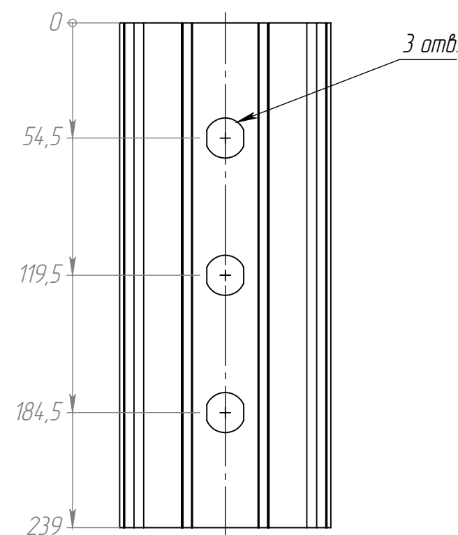
Рис.7: 195.004-05 (2000A) остальное см.рис. 1
