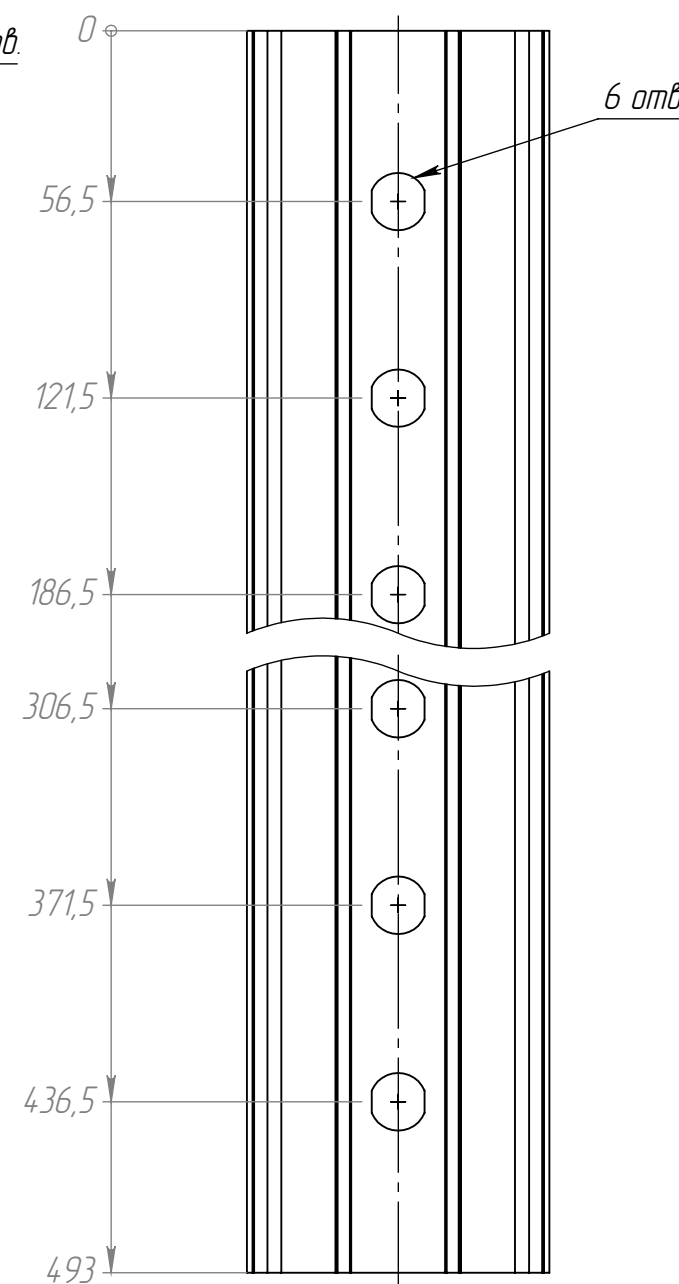
Рис.10 195.004-08 (4000A) остальное см.рис. 1
