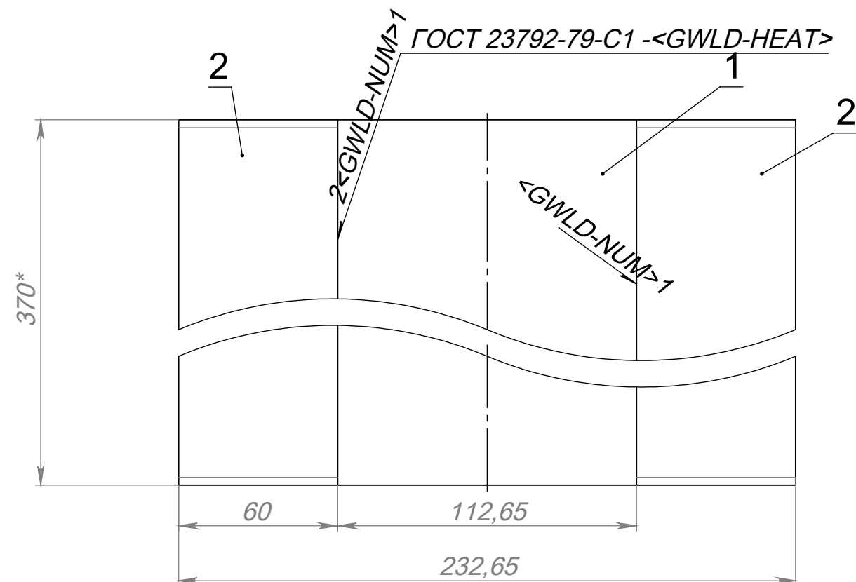
дет. поз. 1 и поз.2
