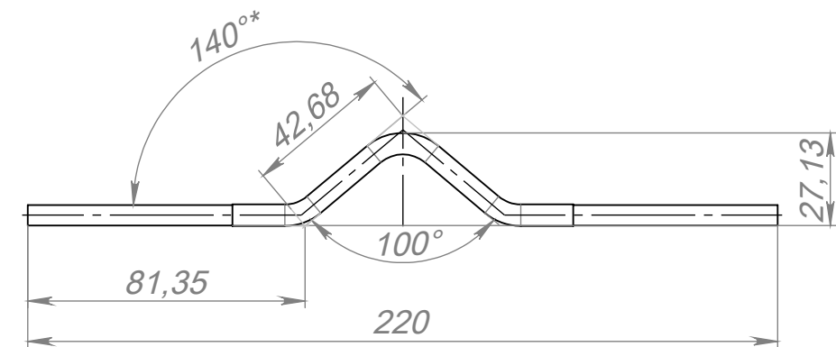
Рис. 1 Гибы пакета шин Дет. поз.3 не показана
