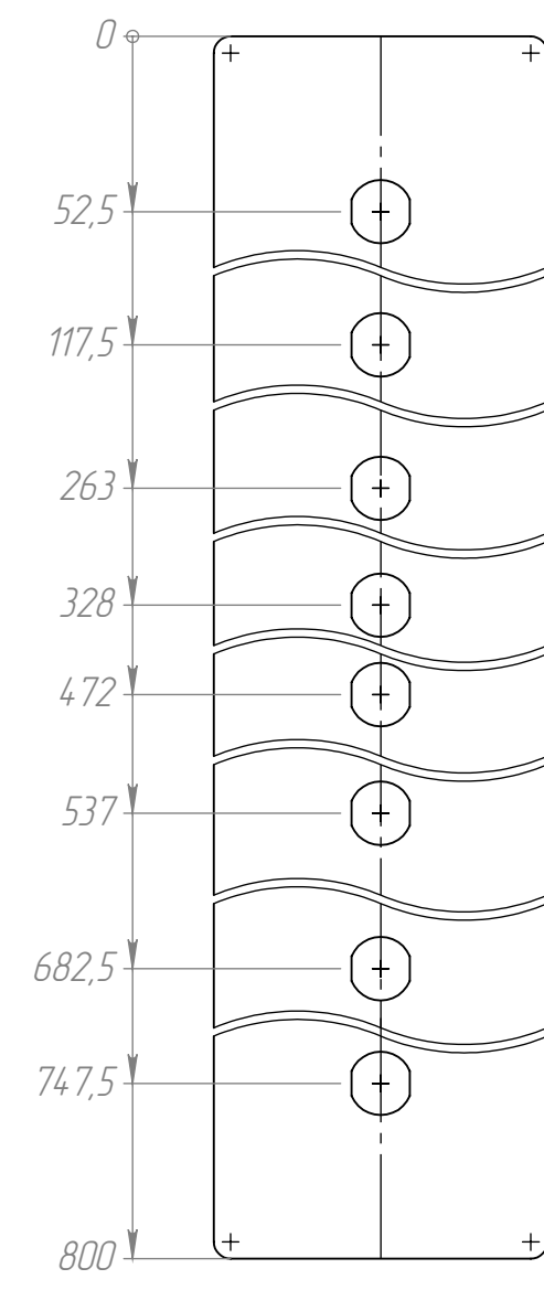
Рис. 3 781.005-02 (6300A) остальное см. рис. 1
