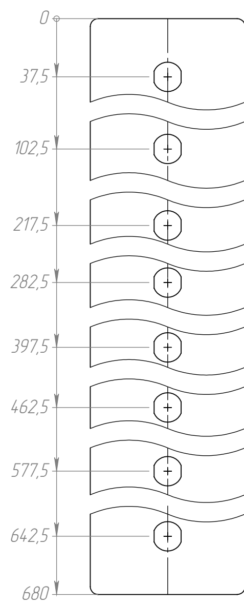
Рис. 2 781.005-01 (5000A) остальное см. рис. 1
