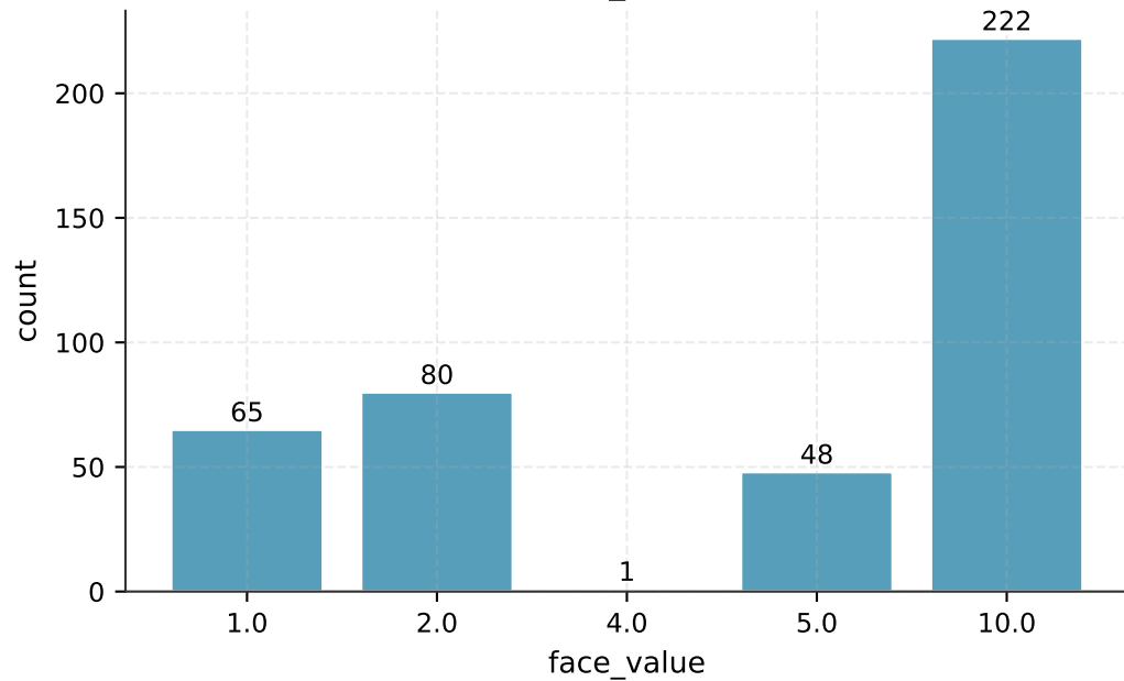
face_value
