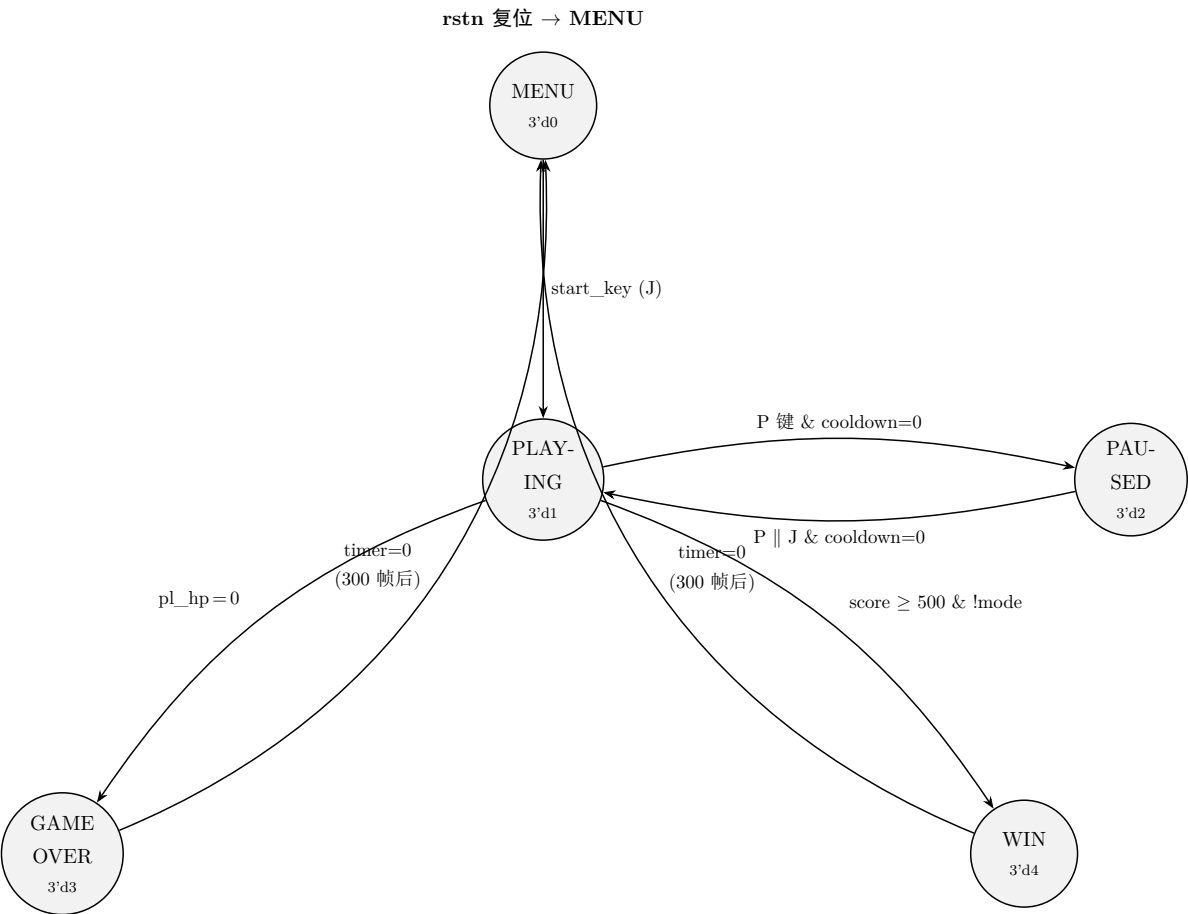
图 5: 游戏状态机状态转换图（Moore 型 FSM）
