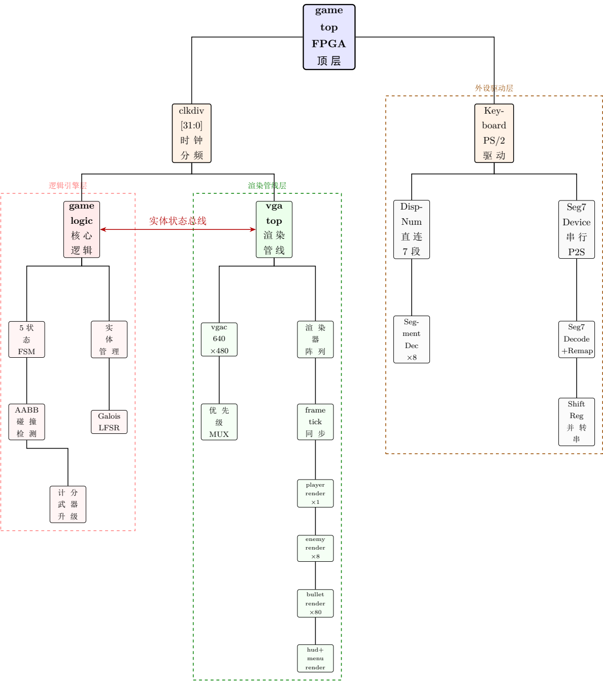
图 2: 模块关系结构图
