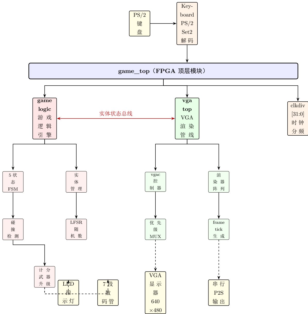
图 1: 系统总体架构框图
