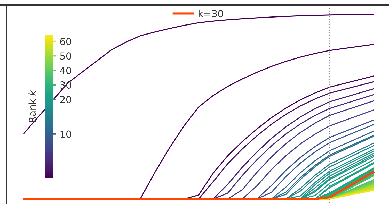
NNM / PGD+FW
