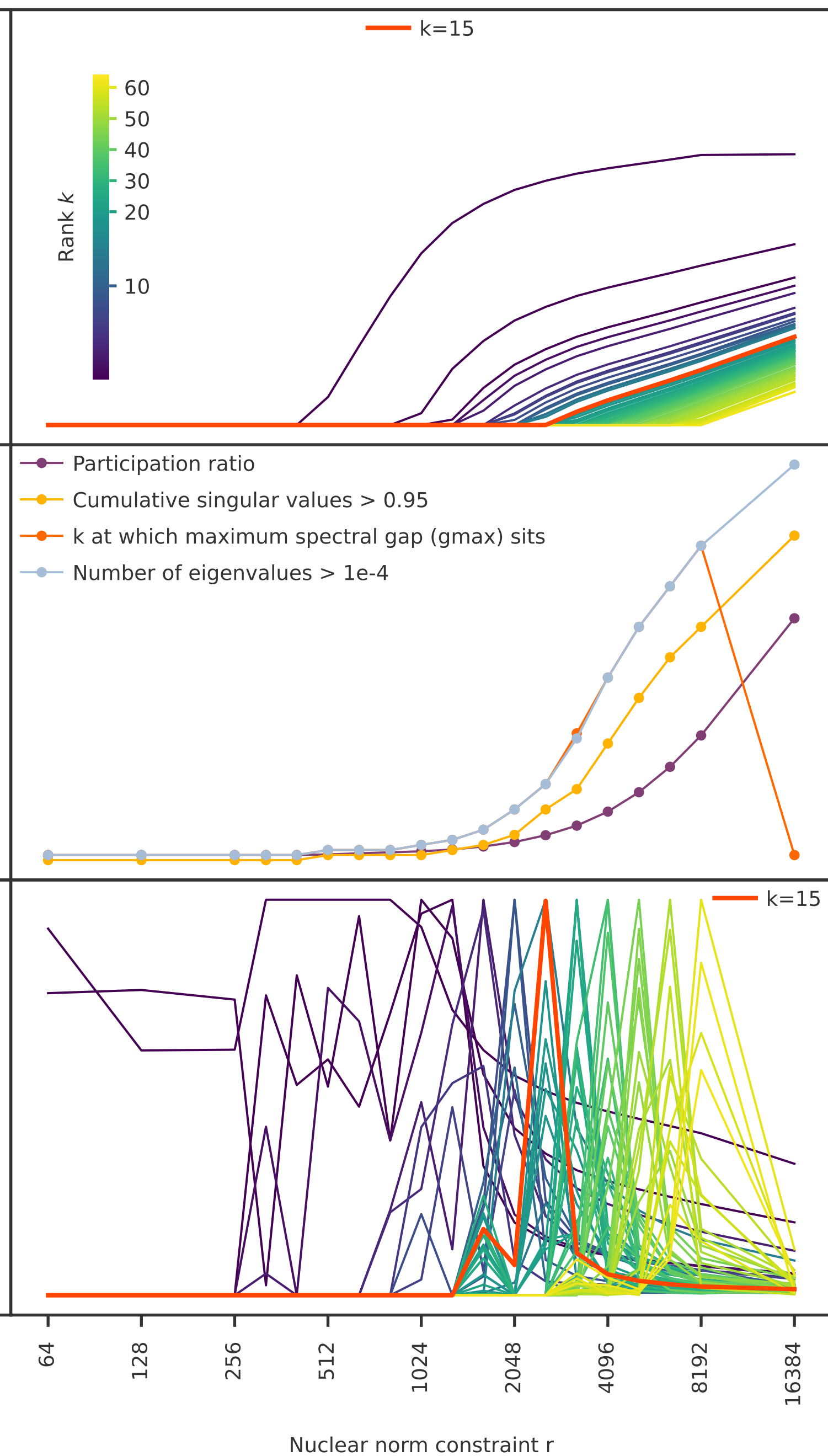
NNM / PGD+FW
