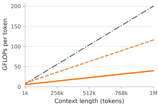
Prefill FLOPs
