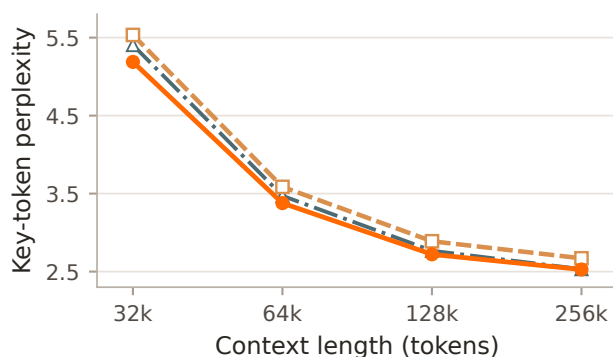
(d) LongPPL ↓
