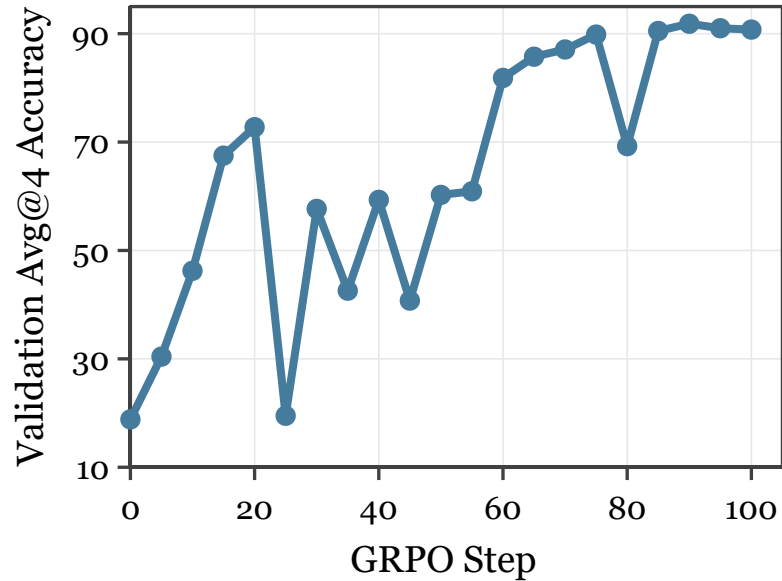
ALFWWorld
