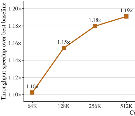
(a) NemotronDiffusion 14B
