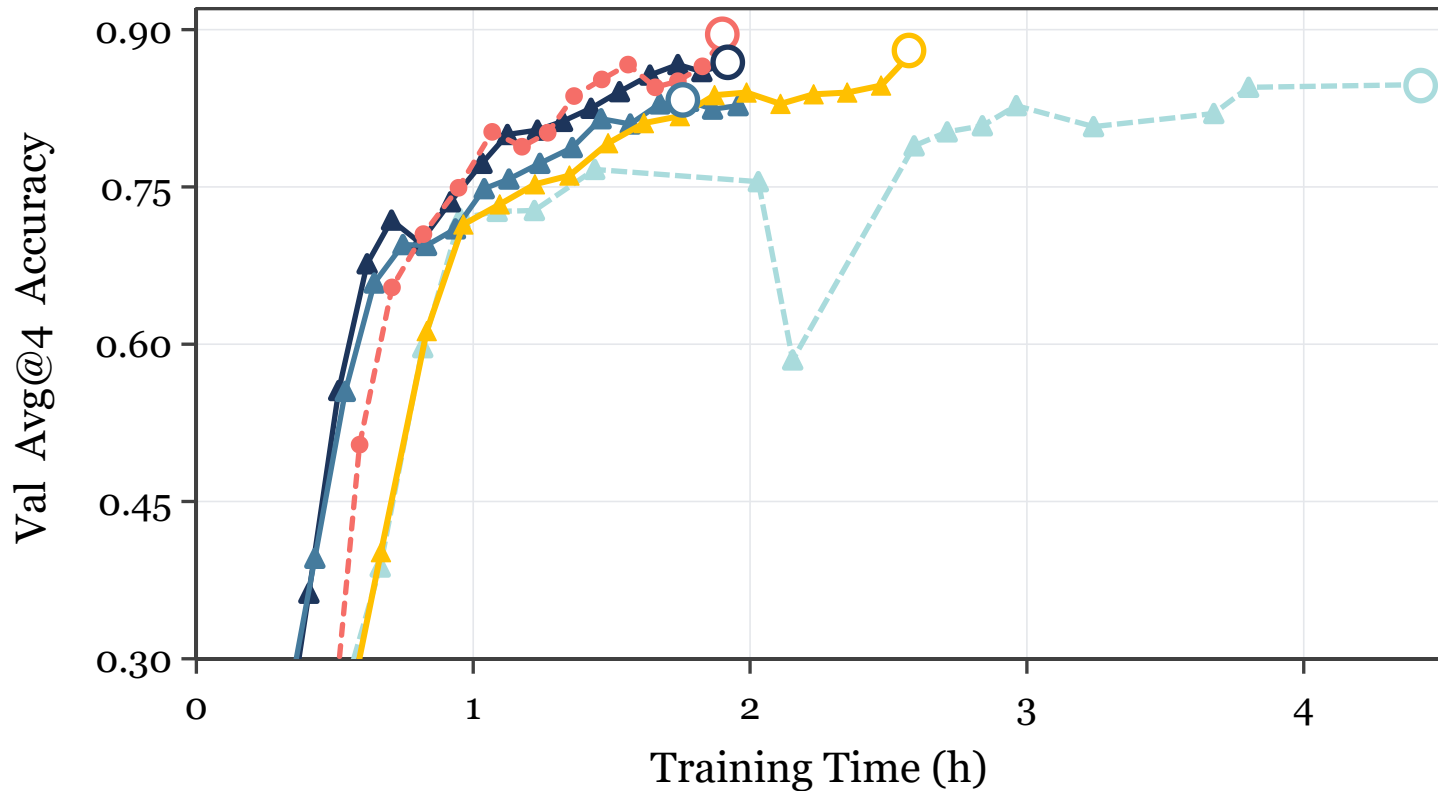
ALFWorld-1.7B
