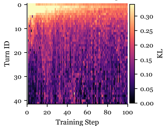
ALFWorld-4B Heatmap
