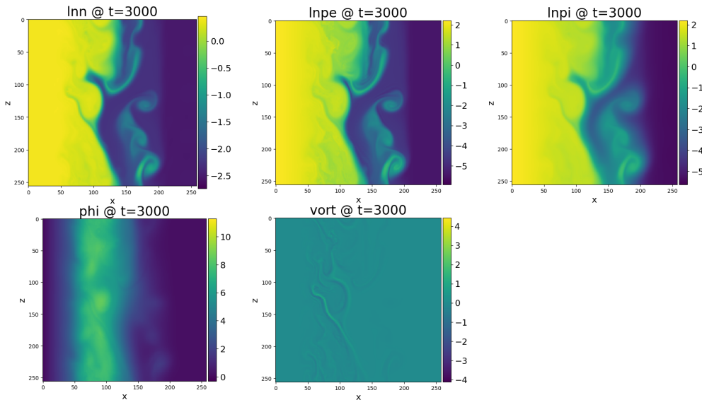
Figure 3: Standard simuleringen Alexander_pi til t = 3000 . Akserne er i numeriske grid enheder og ghost cells inkluderet. Fysiske enheder er z = 140/\rho_s , x = 140/\rho_s + \text{ghostcells}
