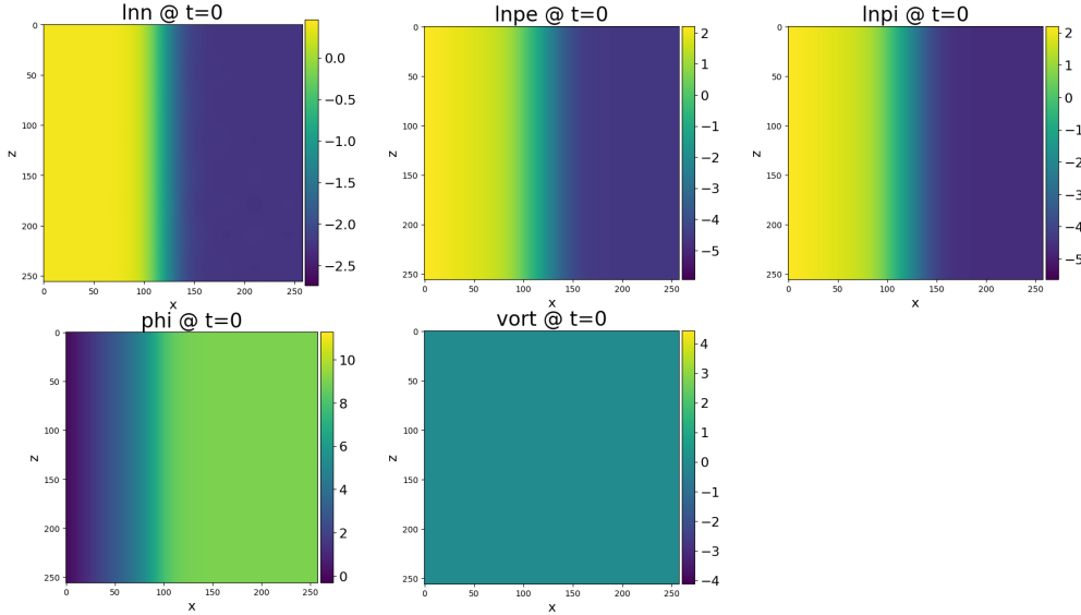
Figure 2: Standard simuleringen Alexander_pi til t = 0 . Akserne er i numeriske grid enheder og ghost cells inkluderet. Fysiske enheder er z = 140/\rho_s , x = 140/\rho_s + \text{ghostcells}
