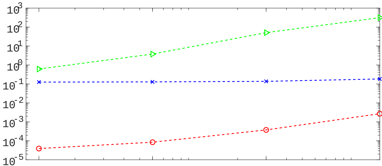
最优分解计算时间(秒)
