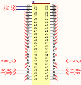
PC104
