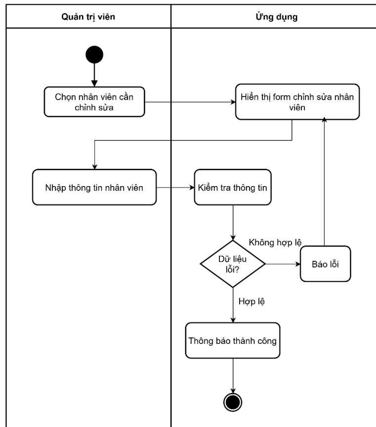
Hình 3-156: Sơ đồ hoạt động chỉnh sửa nhân viên
