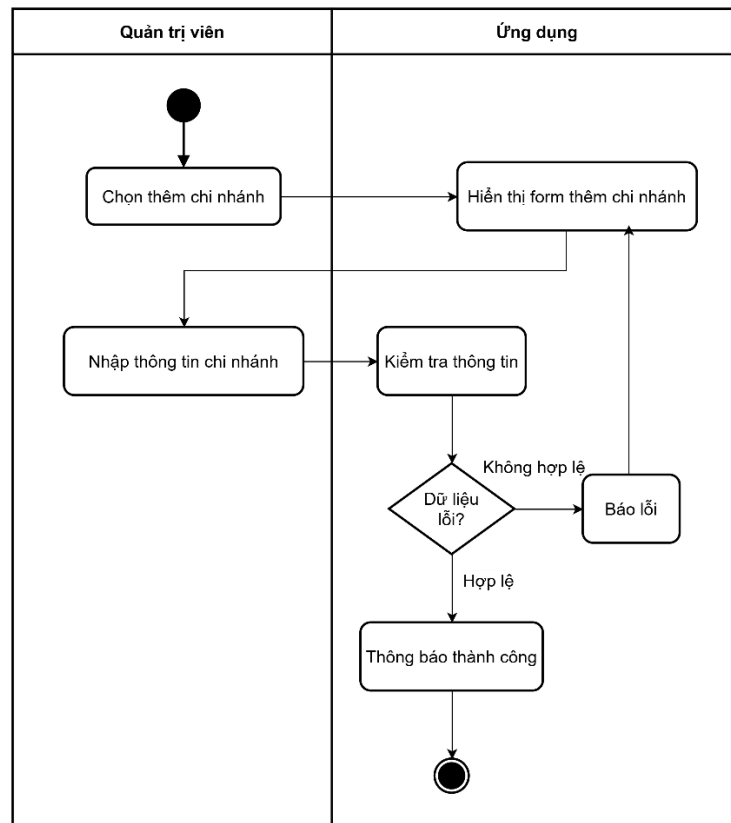
Hình 3-138: Sơ đồ hoạt động thêm chi nhánh
