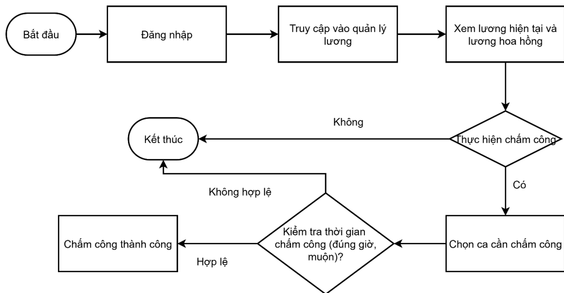
Hình 2-12: Sơ đồ quy trình quản lý lương của kỹ thuật viên
