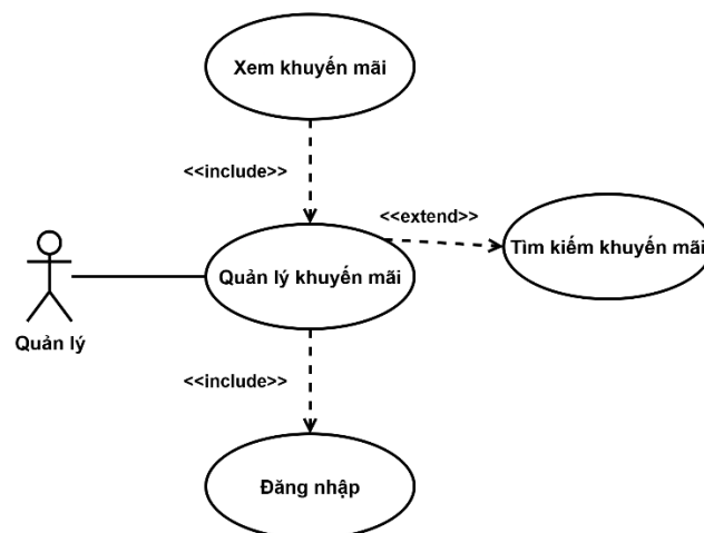
Hình 3-22: Sơ đồ use case quản lý khuyến mãi của quản lý
