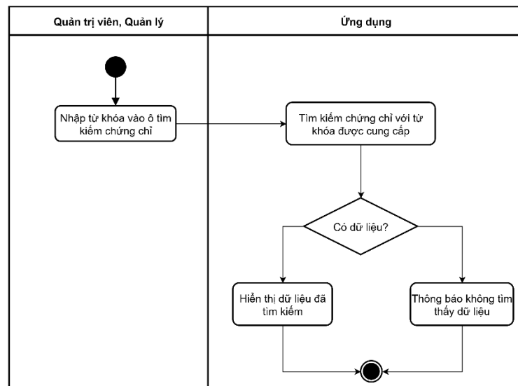
Hình 3-178: Sơ đồ hoạt động tìm kiếm chứng chỉ
