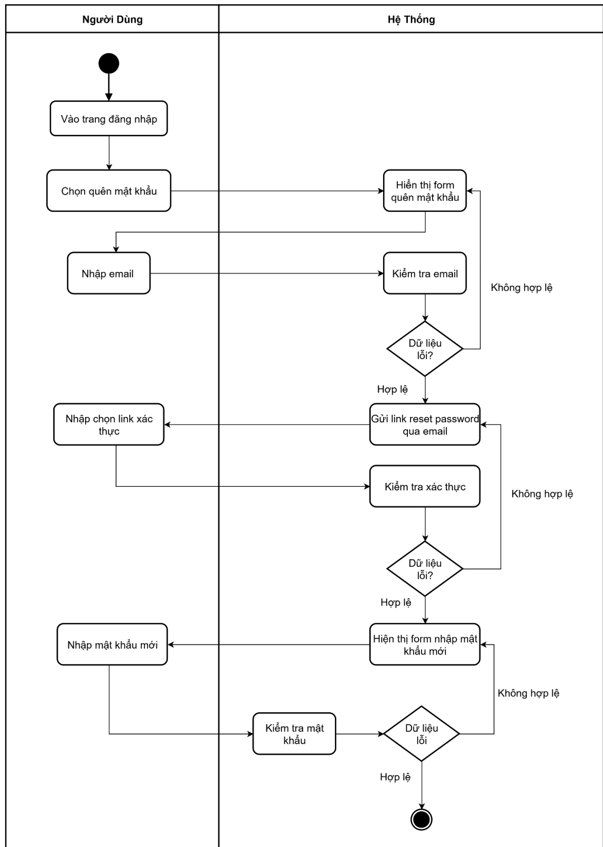
Hình 3-132: Sơ đồ hoạt động quên mật khẩu
