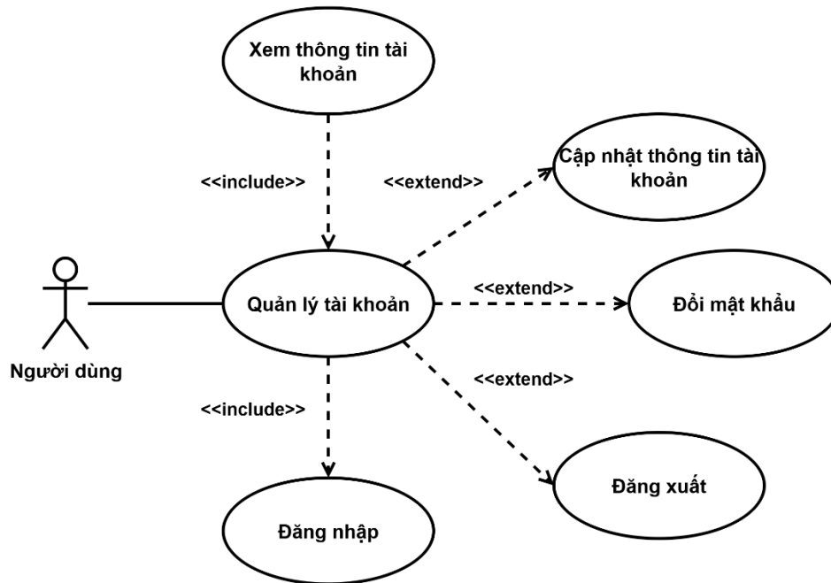
Hình 3-3: Sơ đồ use case quản lý tài khoản
