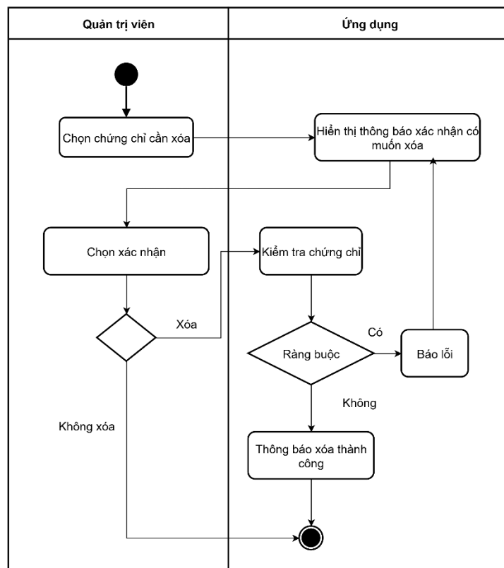
Hình 3-177: Sơ đồ hoạt động xóa chứng chỉ
