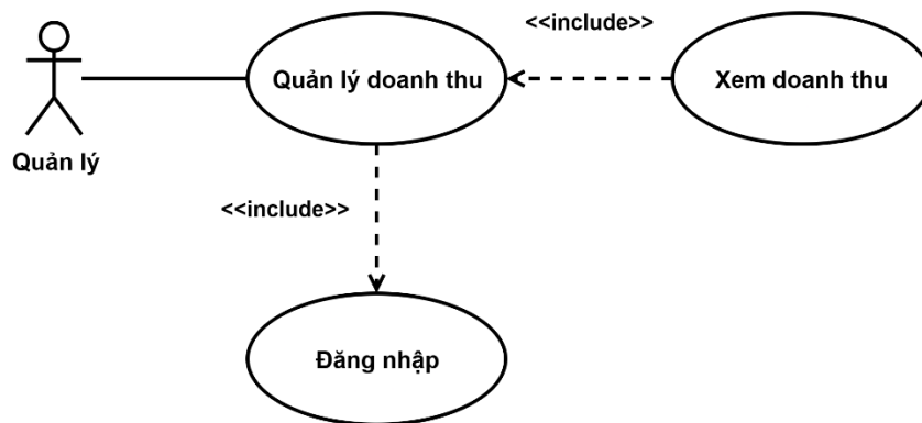
Hình 3-25: Sơ đồ use case quản lý doanh thu của quản lý
