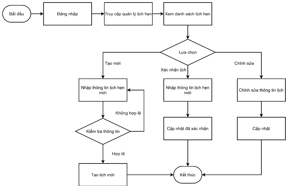
Hình 2-15: Sơ đồ quản lý lịch hẹn của lễ tân
