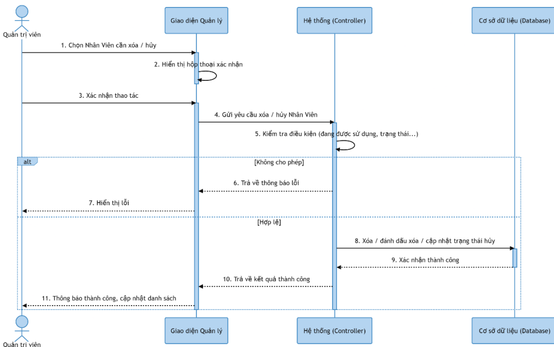
Hình 3-78: Sơ đồ tuần tự xóa nhân viên
