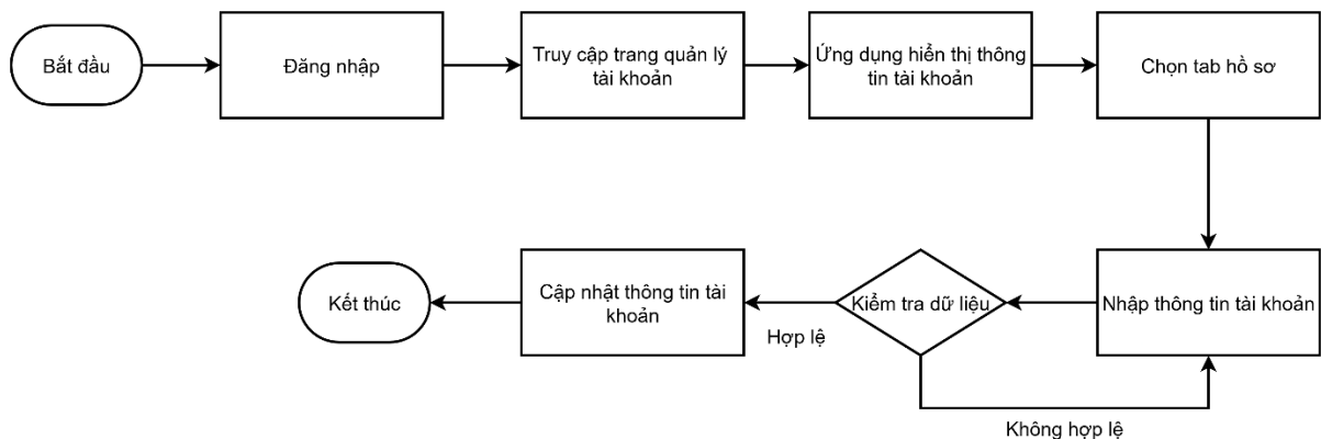
Hình 2-5: Sơ đồ quy trình quản lý tài khoản
