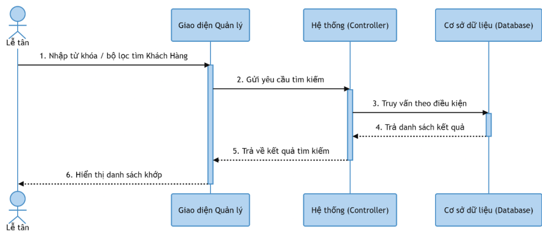
Hình 3-118: Sơ đồ tuần tự tìm kiếm khách hàng
