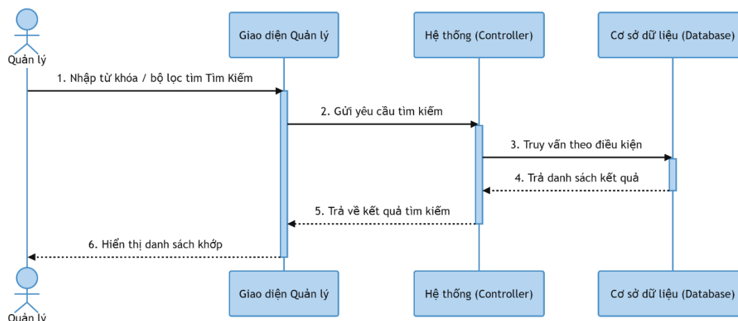
Hình 3-101: Sơ đồ tuần tự tìm kiếm dịch vụ của quản lý
