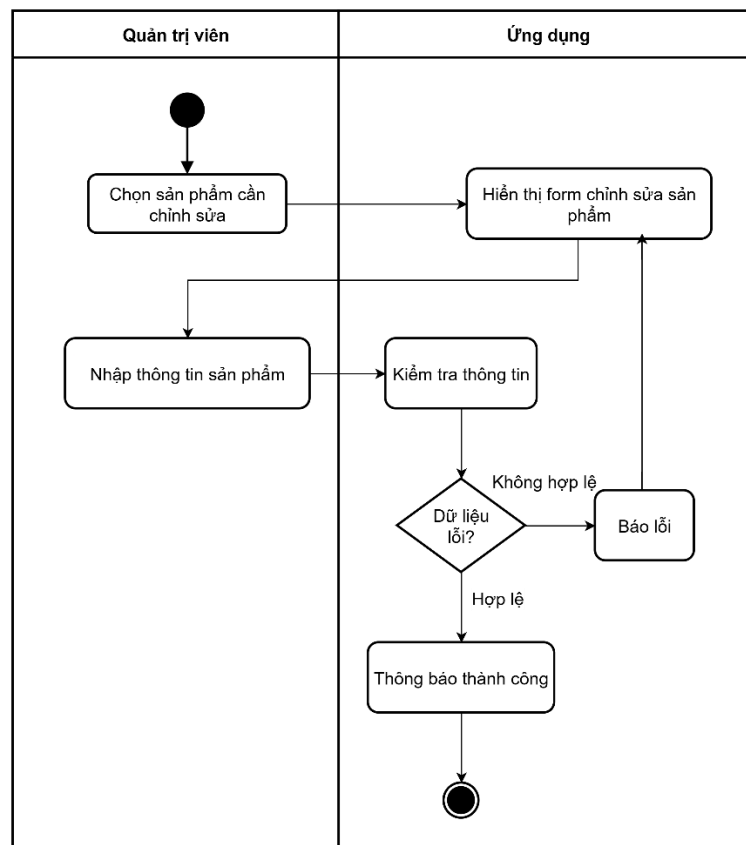
Hình 3-149: Sơ đồ hoạt động sửa sản phẩm
