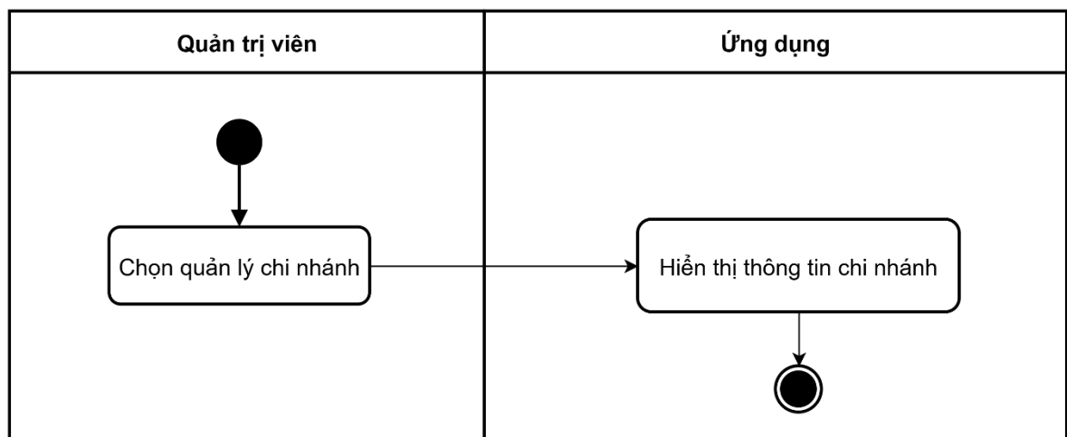
Hình 3-137: Sơ đồ hoạt động xem chi nhánh
