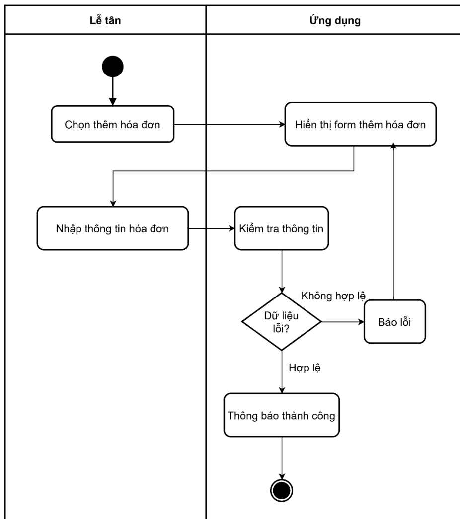
Hình 3-189: Sơ đồ hoạt động tạo hóa đơn
