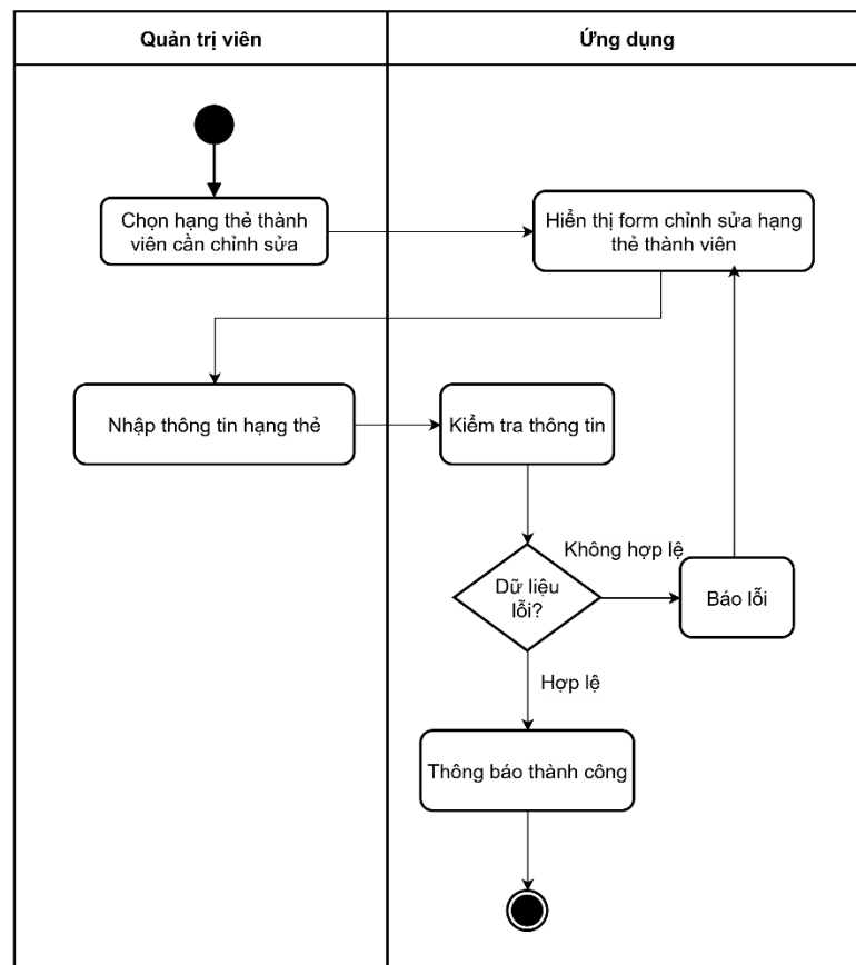
Hình 3-194: Sơ đồ hoạt động sửa hạng thẻ thành viên
