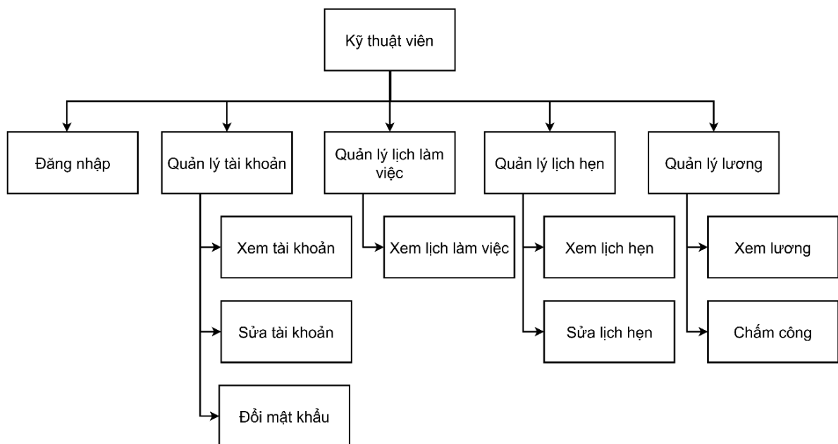
Hình 2-42: Sơ đồ chức năng của kỹ thuật viên
