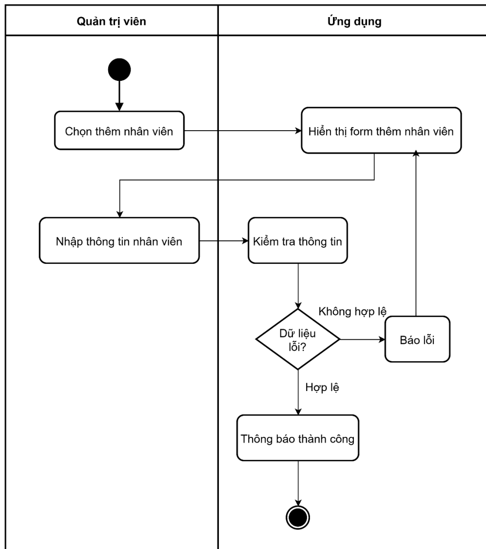
Hình 3-155: Sơ đồ hoạt động thêm nhân viên
