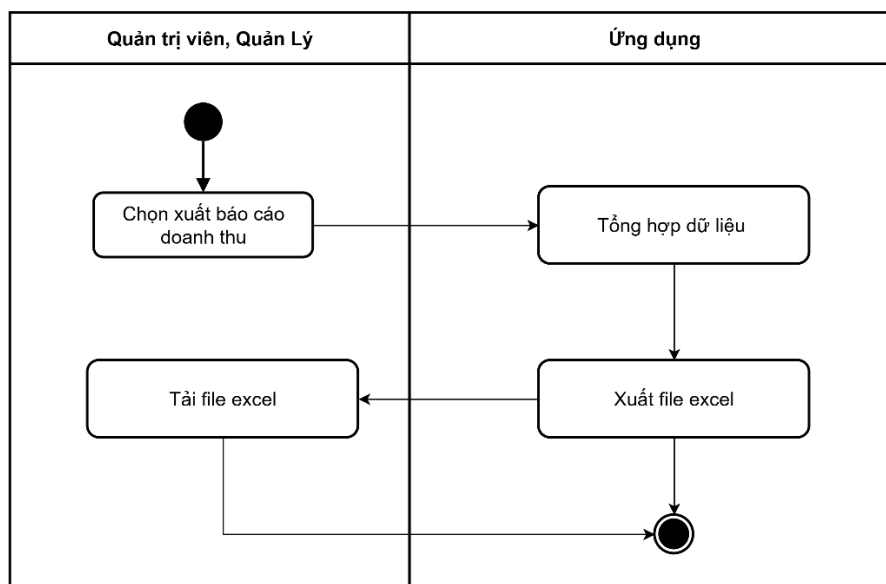
Hình 3-153: Sơ đồ hoạt động xuất doanh thu
