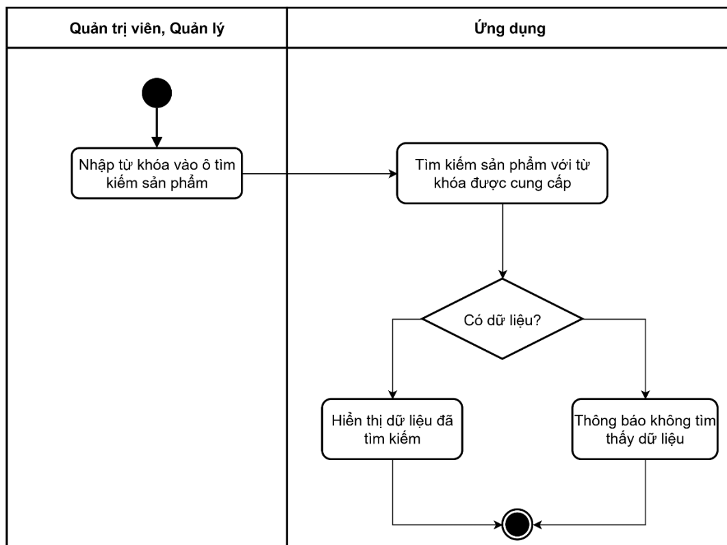
Hình 3-151: Sơ đồ hoạt động tìm kiếm sản phẩm
