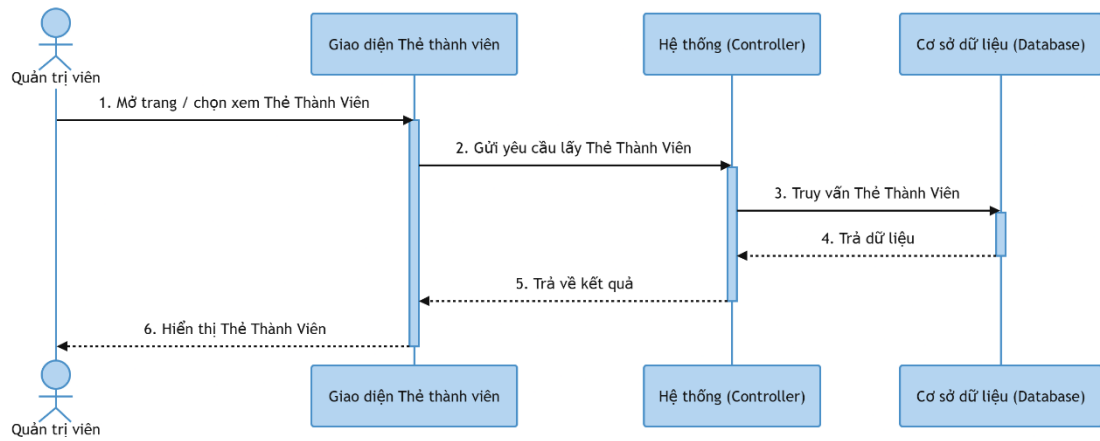
Hình 3-95: Sơ đồ tuần tự xem thẻ thành viên
