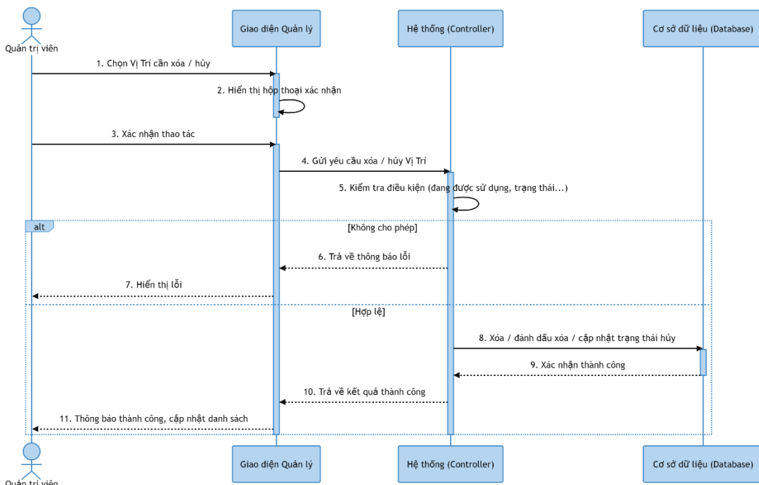
Hình 3-88: Sơ đồ tuần tự xóa vị trí
