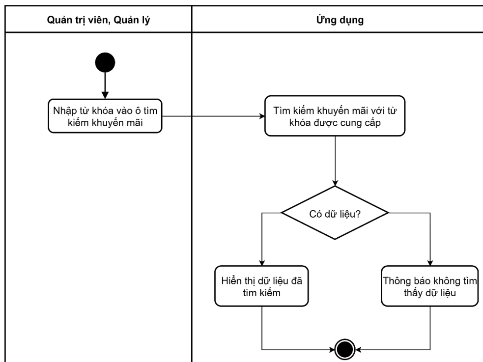
Hình 3-163: Sơ đồ hoạt động tìm kiếm khuyến mãi
