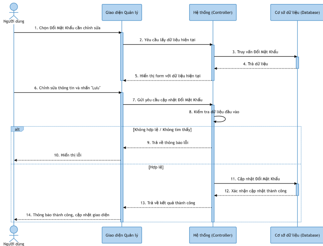
Hình 3-42: Sơ đồ tuần tự đổi mật khẩu
