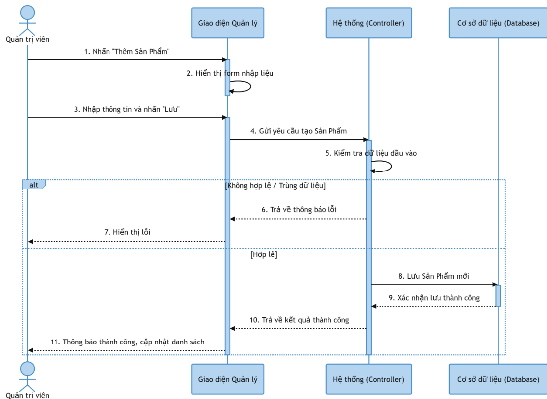
Hình 3-92: Sơ đồ tuần tự thêm sản phẩm
