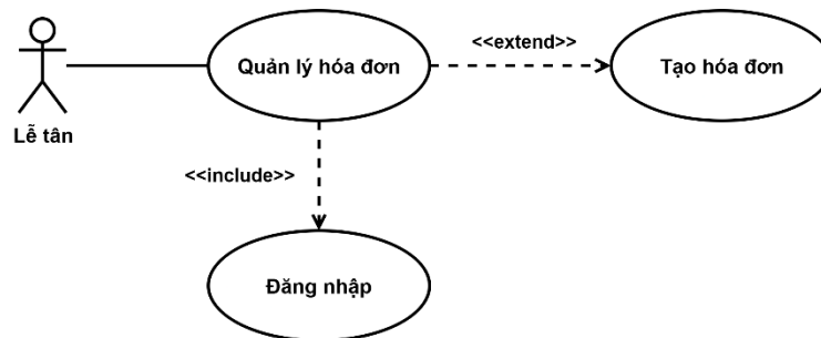
Hình 3-32: Sơ đồ use case chi tiết quản lý hóa đơn của lễ tân
