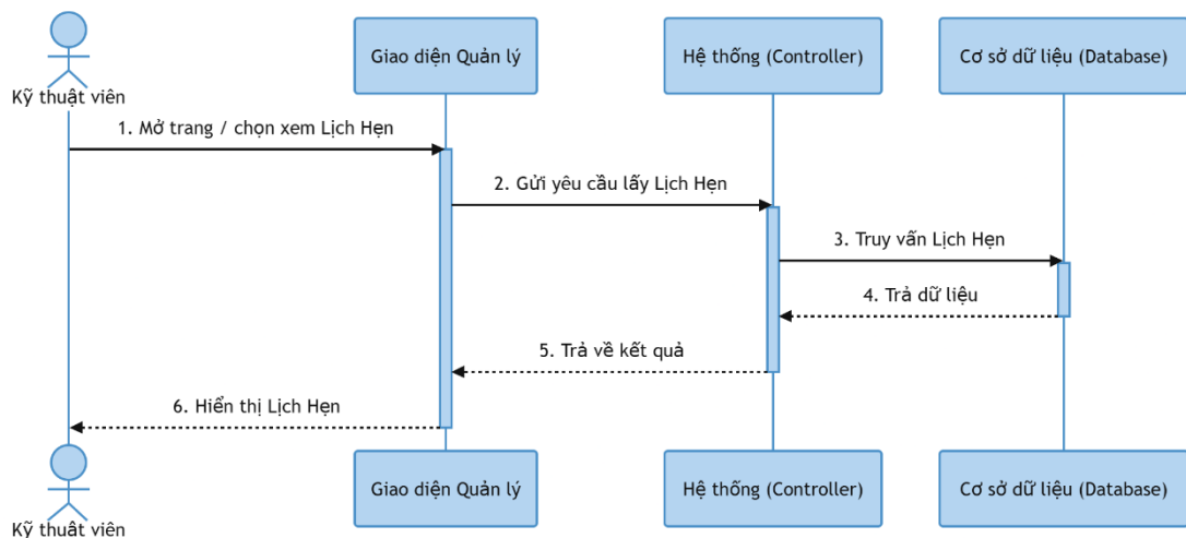
Hình 3-120: Sơ đồ tuần tự xem lịch hẹn
