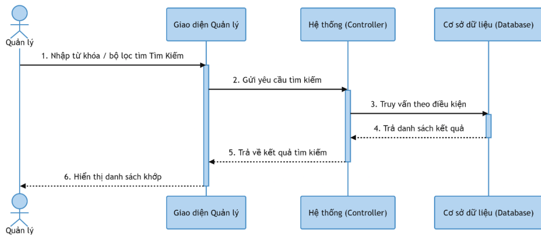
Hình 3-107: Sơ đồ tuần tự tìm kiếm khuyến mãi của quản lý
