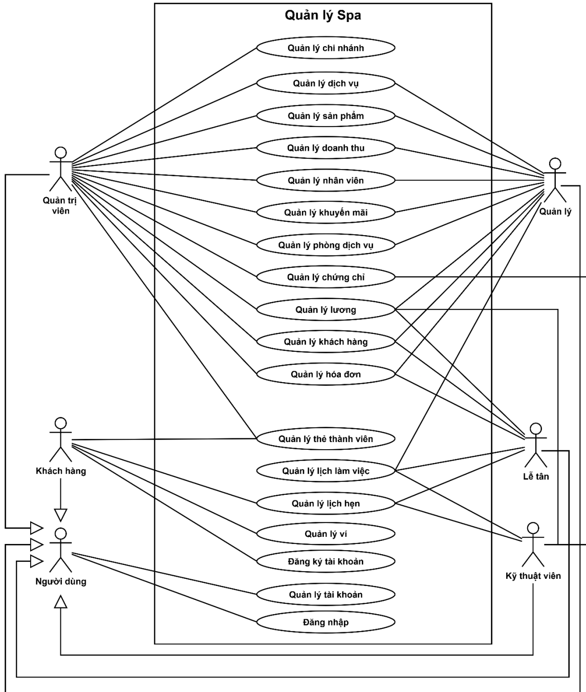
Hình 2-43: Sơ đồ use case tổng quát
