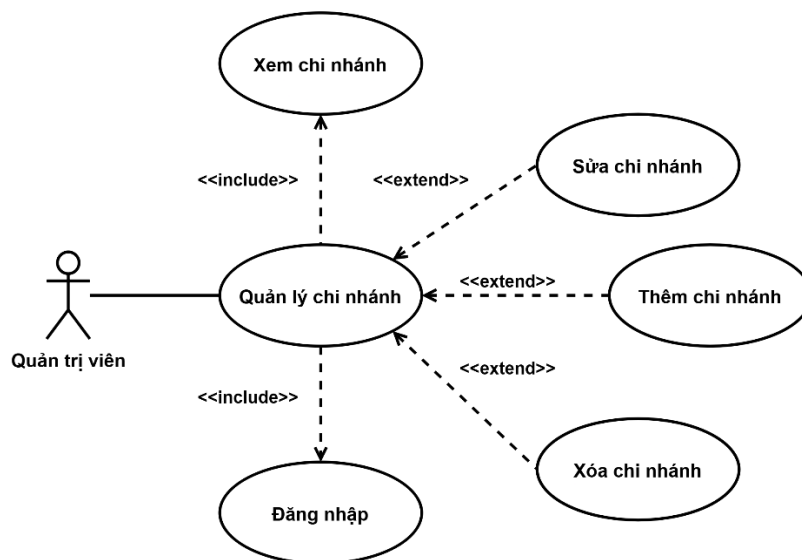
Hình 3-4: Use case quản lý chi nhánh của quản trị viên
