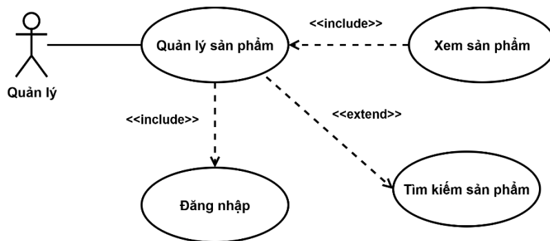
Hình 3-19: Sơ đồ use case chi tiết quản lý sản phẩm của quản lý
