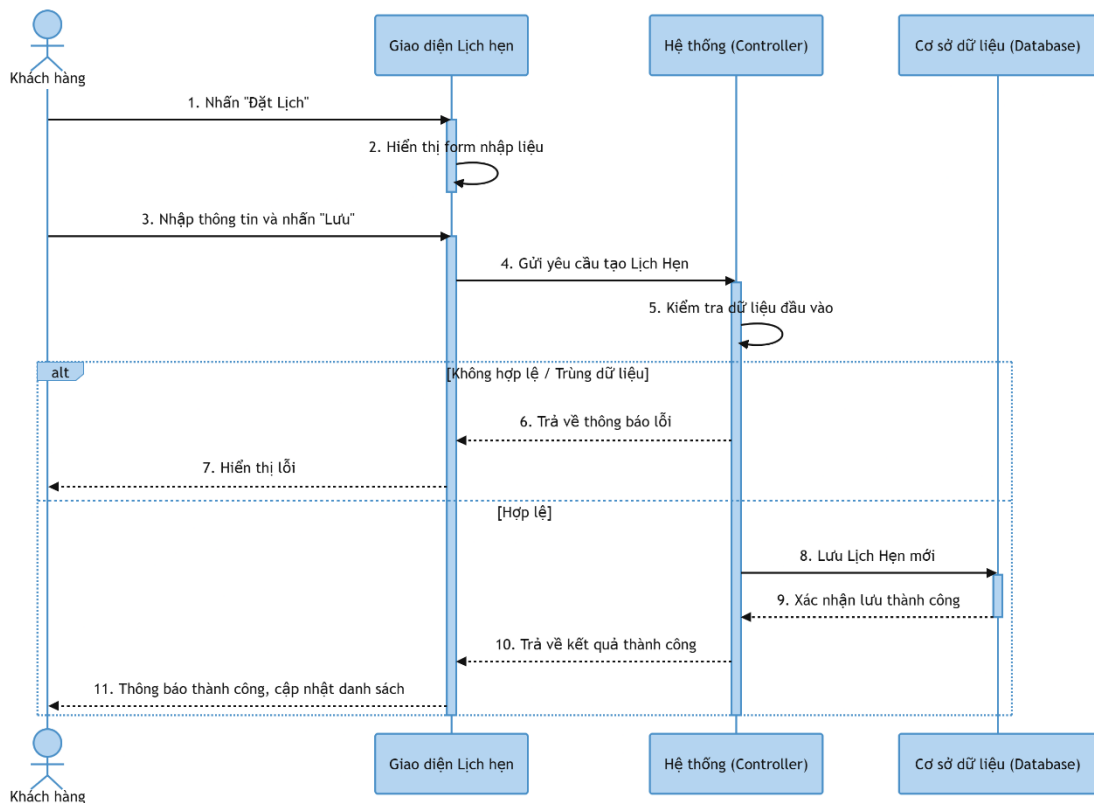
Hình 3-127: Sơ đồ tuần tự đặt lịch hẹn
