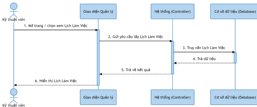
Hình 3-122: Sơ đồ tuần tự xem lịch làm việc
