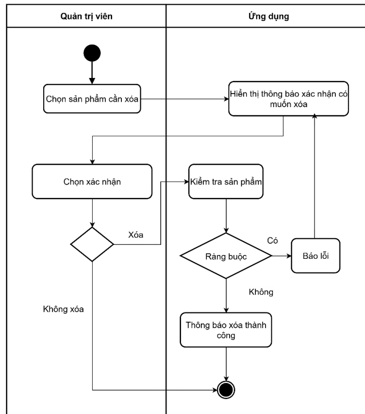
Hình 3-150: Sơ đồ hoạt động xóa sản phẩm
