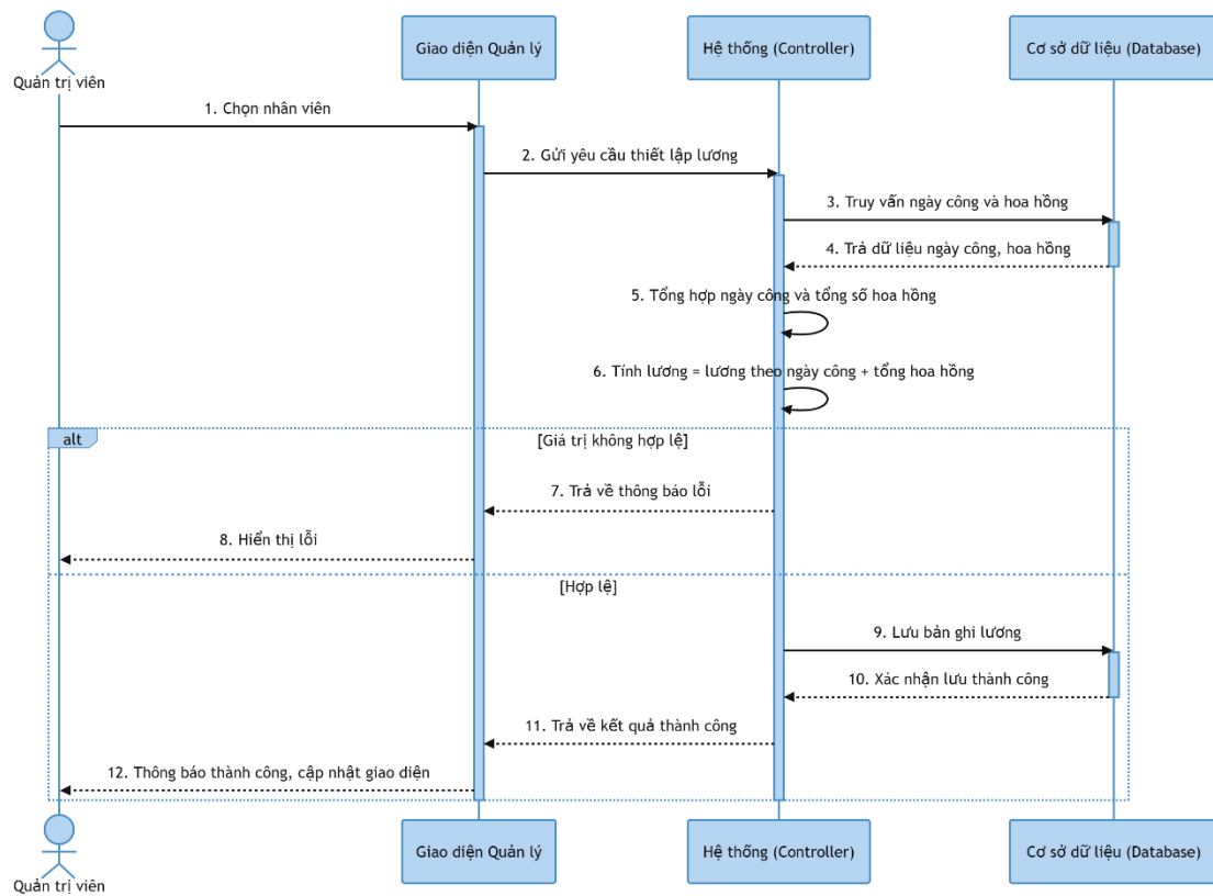
Hình 3-73: Sơ đồ tuần tự tính lương
