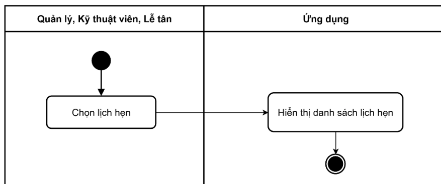
Hình 3-200: Sơ đồ hoạt động xem lịch hẹn
