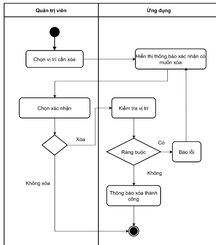
Hình 3-172: Sơ đồ hoạt động xóa vị trí
