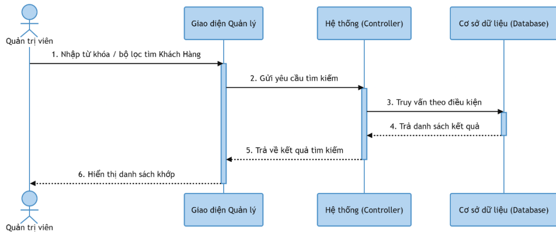
Hình 3-65: Sơ đồ tuần tự tìm kiếm khách hàng
