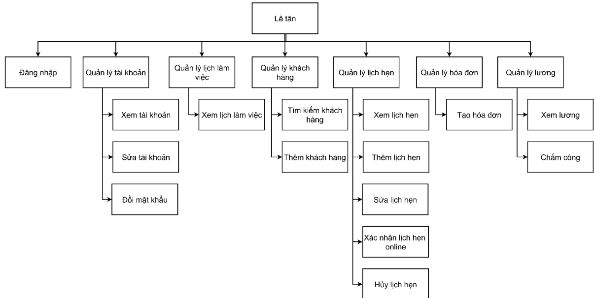
Hình 2-41: Sơ đồ chức năng của lễ tân
