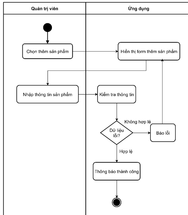
Hình 3-148: Sơ đồ hoạt động thêm sản phẩm
