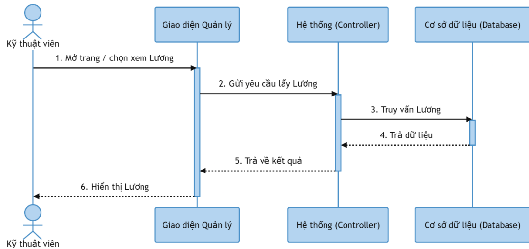
Hình 3-123: Sơ đồ tuần tự xem lương
