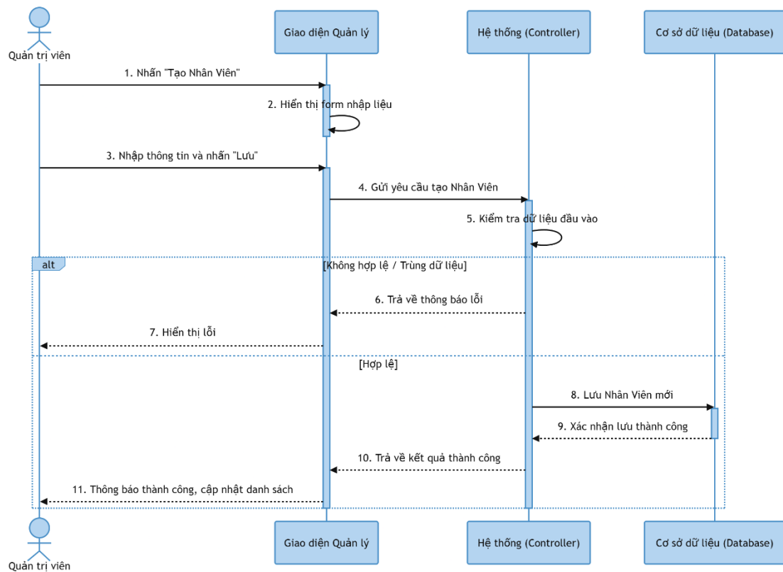
Hình 3-76: Sơ đồ tuần tự tạo nhân viên
