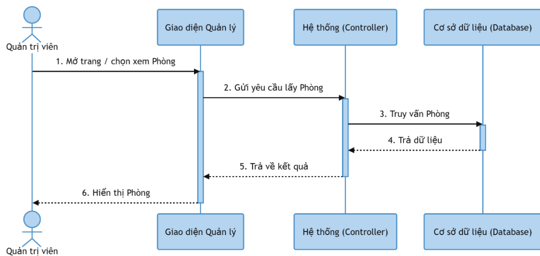
Hình 3-80: Sơ đồ tuần tự xem danh sách phòng
