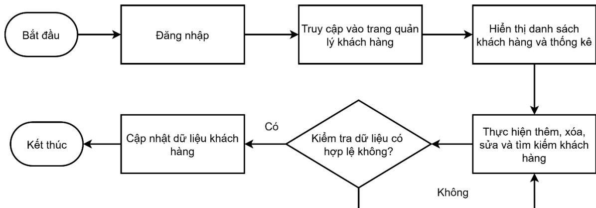
Hình 2-31: Sơ đồ quản lý khách hàng của quản trị viên
