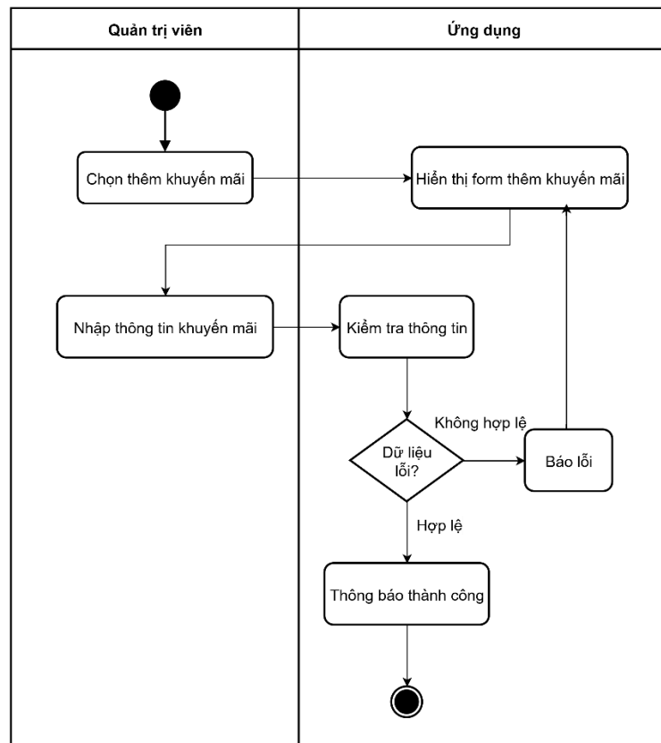
Hình 3-160: Sơ đồ hoạt động thêm khuyến mãi
