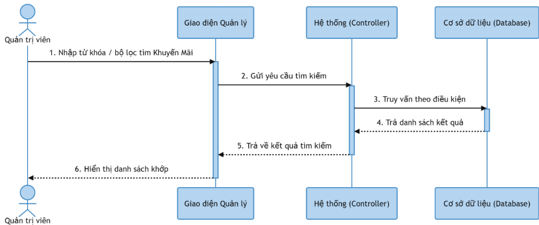
Hình 3-70: Sơ đồ tuần tự tìm kiếm khuyến mãi
