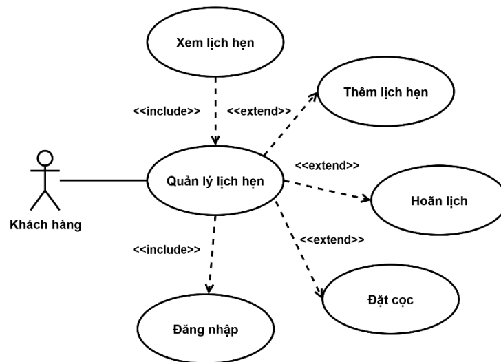
Hình 3-35: Sơ đồ use case quản lý lịch hẹn
