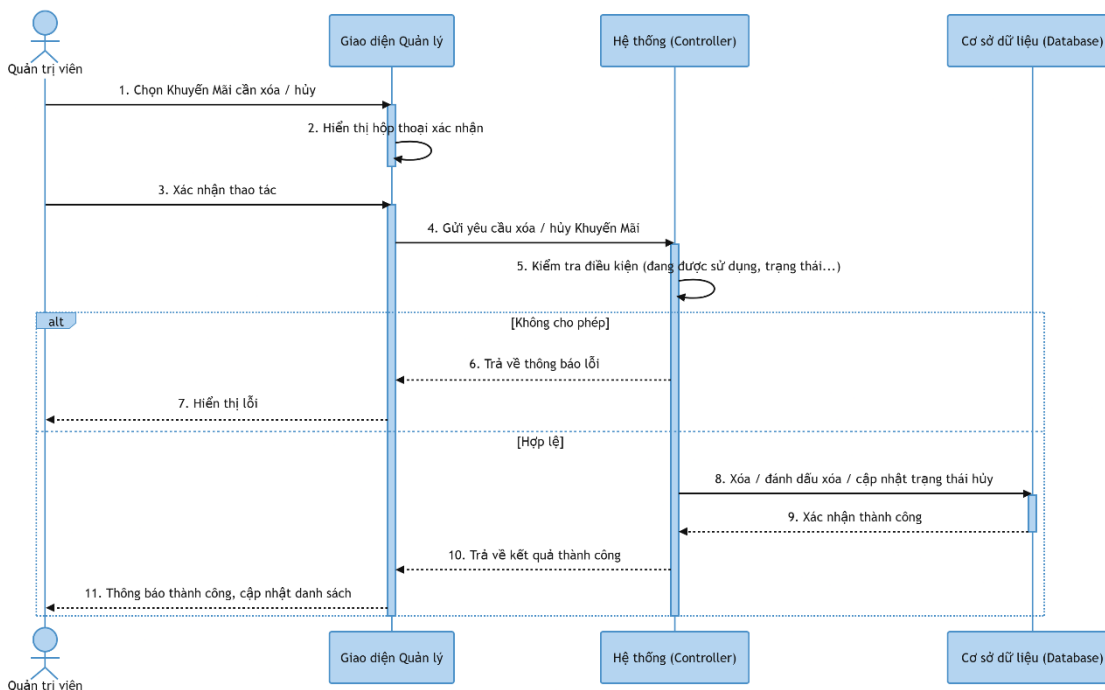
Hình 3-69: Sơ đồ tuần tự xóa khuyến mãi
