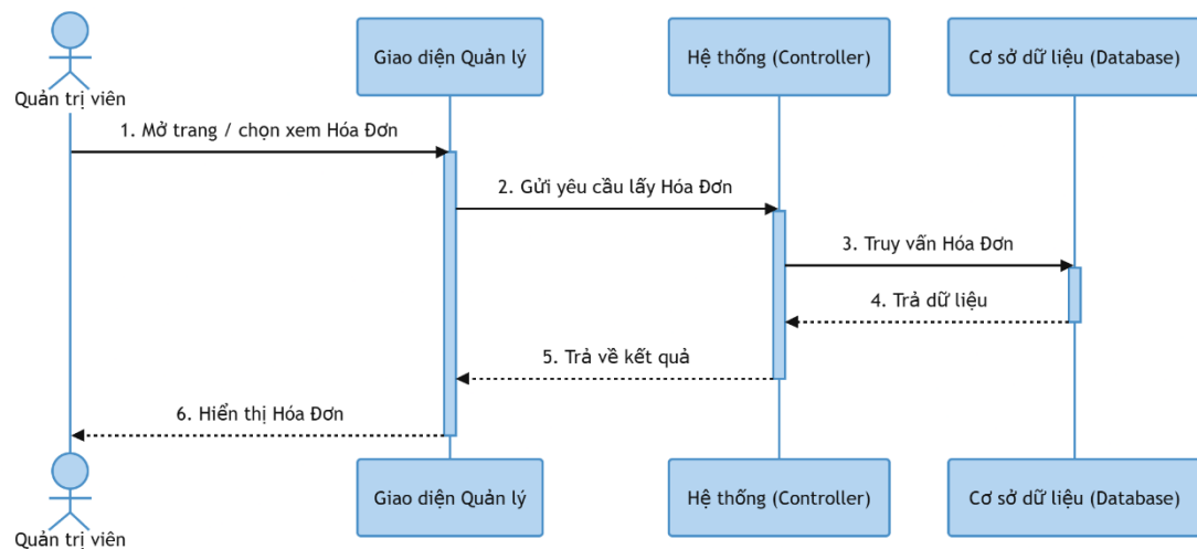
Hình 3-58: Sơ đồ tuần tự xem danh sách hóa đơn
