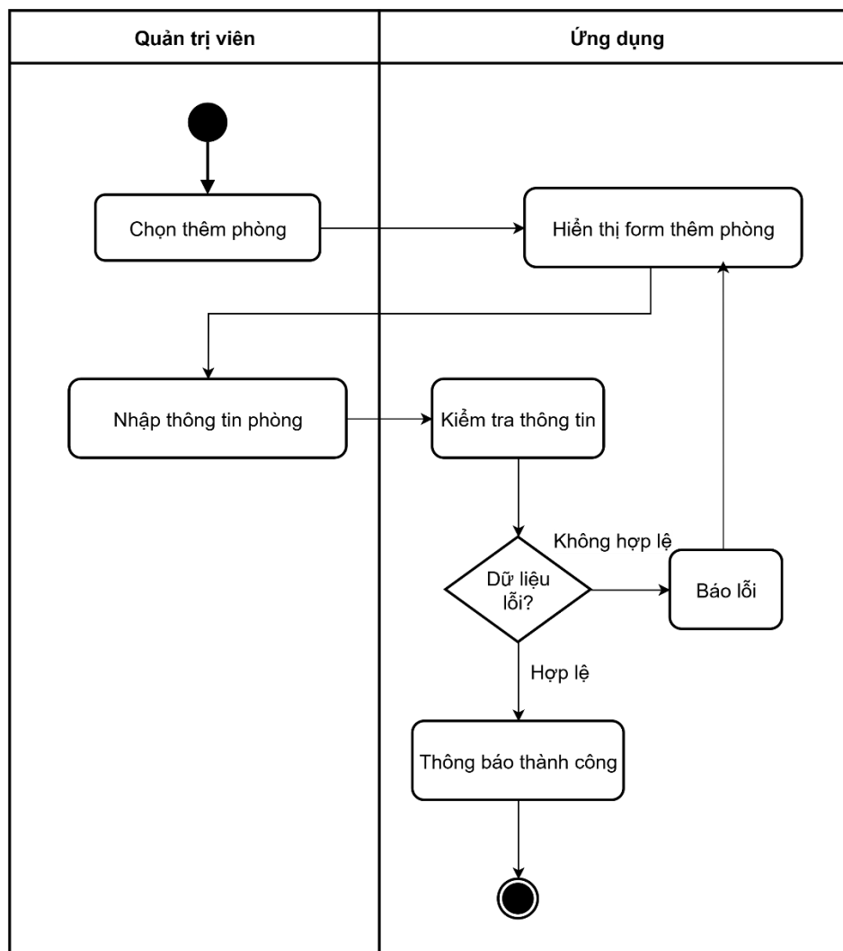
Hình 3-165: Sơ đồ hoạt động thêm phòng
