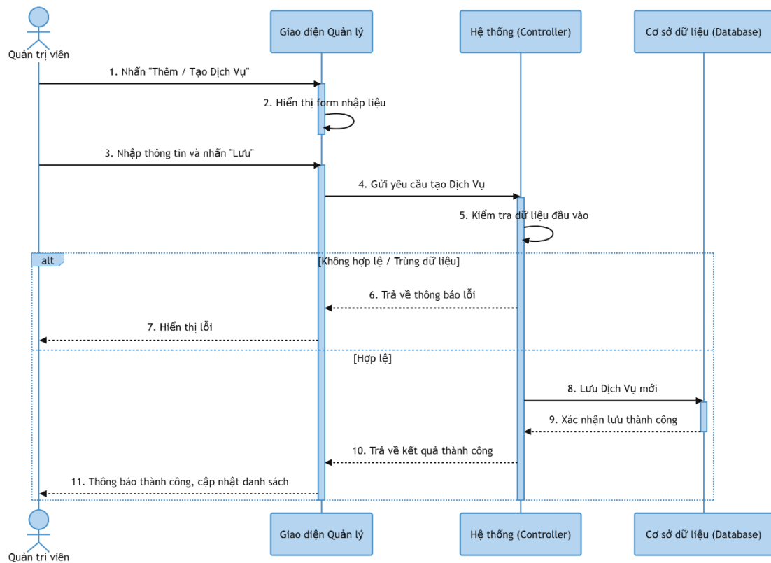
Hình 3-52: Sơ đồ tuần tự tạo dịch vụ
