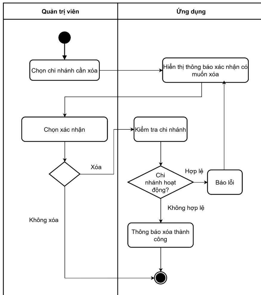
Hình 3-140: Sơ đồ hoạt động xóa chi nhánh
