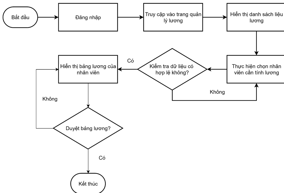
Hình 2-33: Sơ đồ chức năng quản lý lương của quản trị viên
