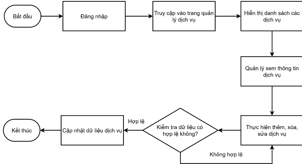
Hình 2-28: Sơ đồ quản lý dịch vụ của quản trị viên
