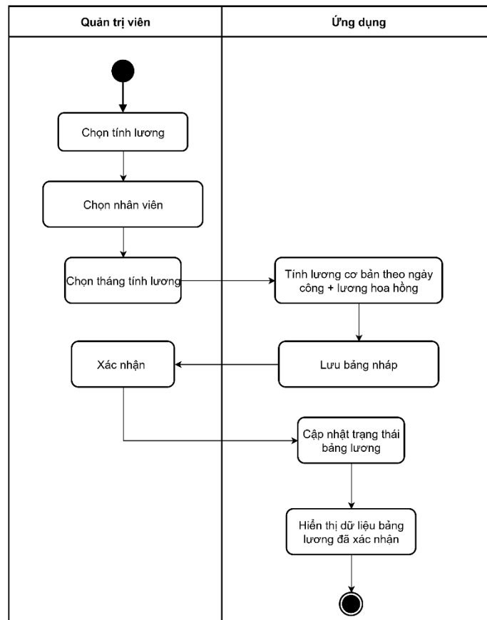
Hình 3-180: Sơ đồ hoạt động tính lương
