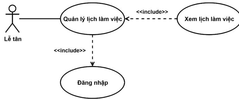
Hình 3-29: Sơ đồ use case chi tiết quản lý lịch làm việc của lễ tân
