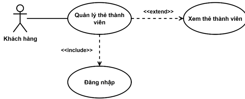
Hình 3-36: Sơ đồ use case chi tiết quản lý thẻ thành viên
