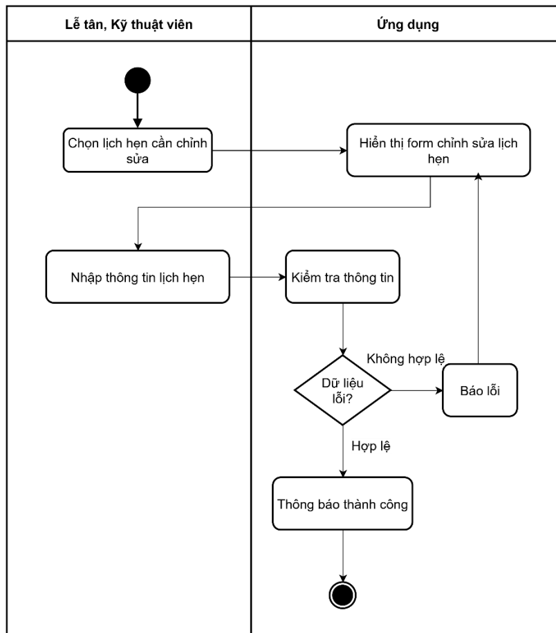
Hình 3-202: Sơ đồ hoạt động sửa lịch hẹn
