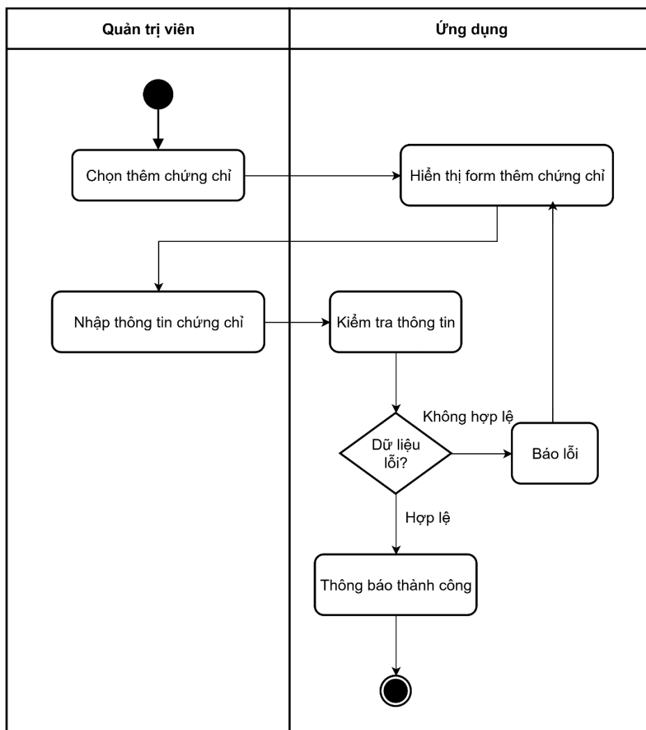
Hình 3-175: Sơ đồ hoạt động thêm chứng chỉ
