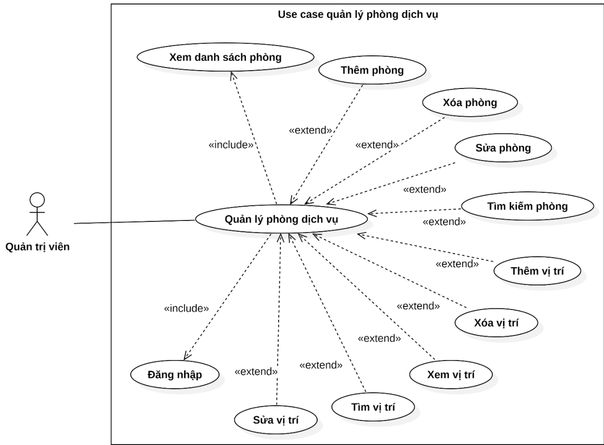
Hình 3-8: Sơ đồ use case chi tiết quản lý phòng dịch vụ của quản trị viên
