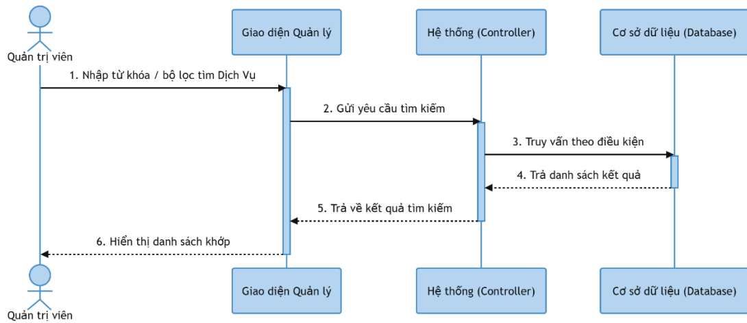
Hình 3-55: Sơ đồ tuần tự tìm kiếm dịch vụ
