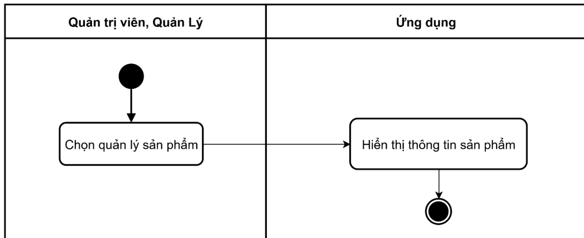
Hình 3-147: Sơ đồ hoạt động xem thông tin sản phẩm
