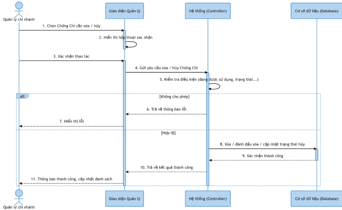
Hình 3-50: Sơ đồ tuần tự xóa chứng chỉ
