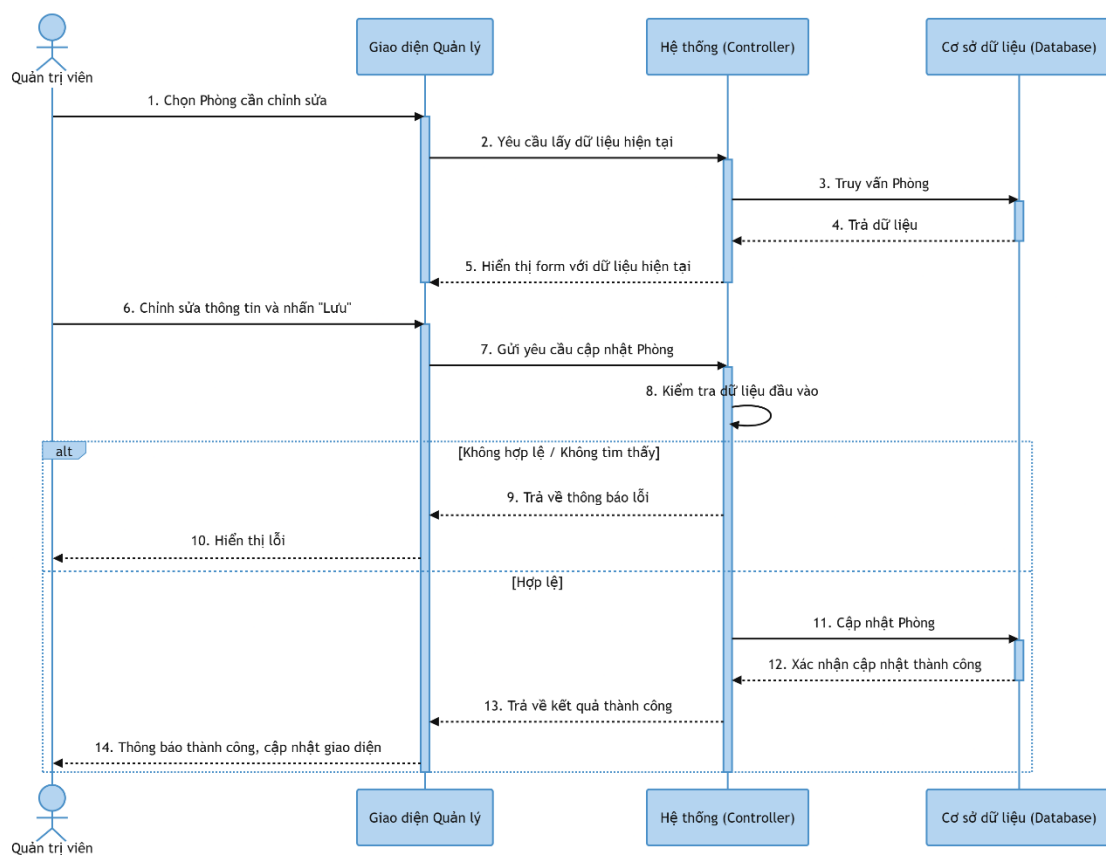
Hình 3-82: Sơ đồ tuần tự chỉnh sửa phòng
