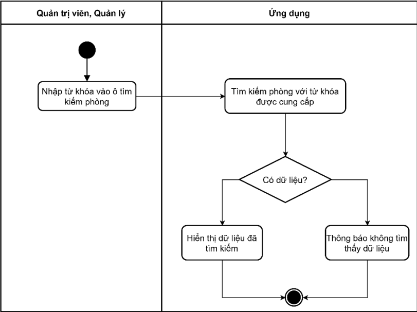
Hình 3-168: Sơ đồ hoạt động tìm kiếm phòng
