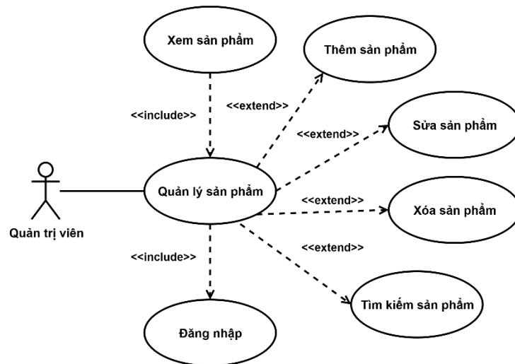
Hình 3-6: Sơ đồ use case quản lý sản phẩm của quản trị viên
