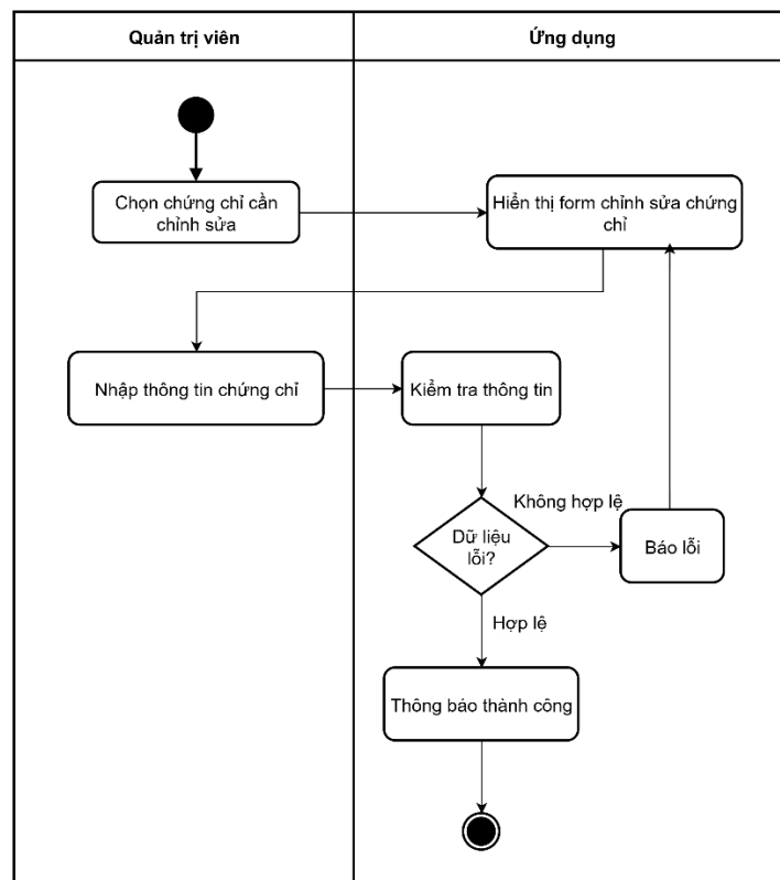
Hình 3-176: Sơ đồ hoạt động chỉnh sửa chứng chỉ
