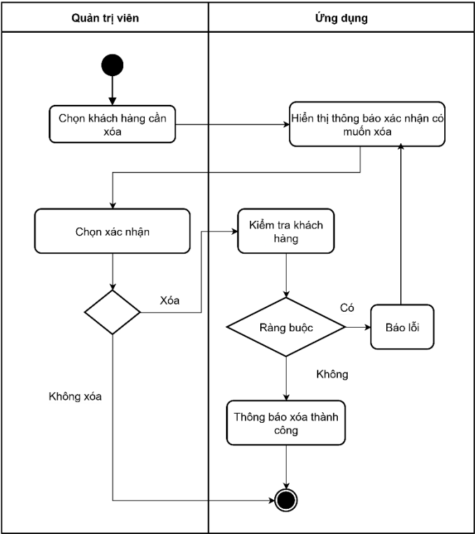
Hình 3-186: Sơ đồ hoạt động xóa khách hàng
