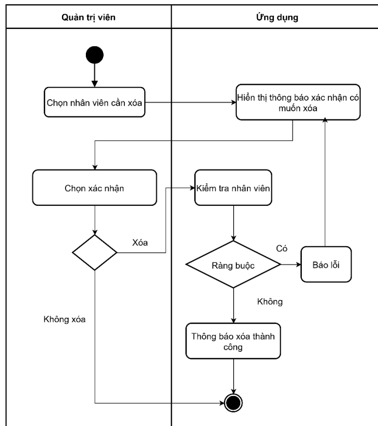
Hình 3-157: Sơ đồ hoạt động xóa nhân viên
