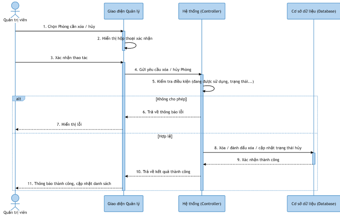
Hình 3-83: Sơ đồ tuần tự xóa phòng
