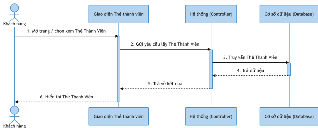
Hình 3-130: Sơ đồ tuần tự xem thẻ thành viên
