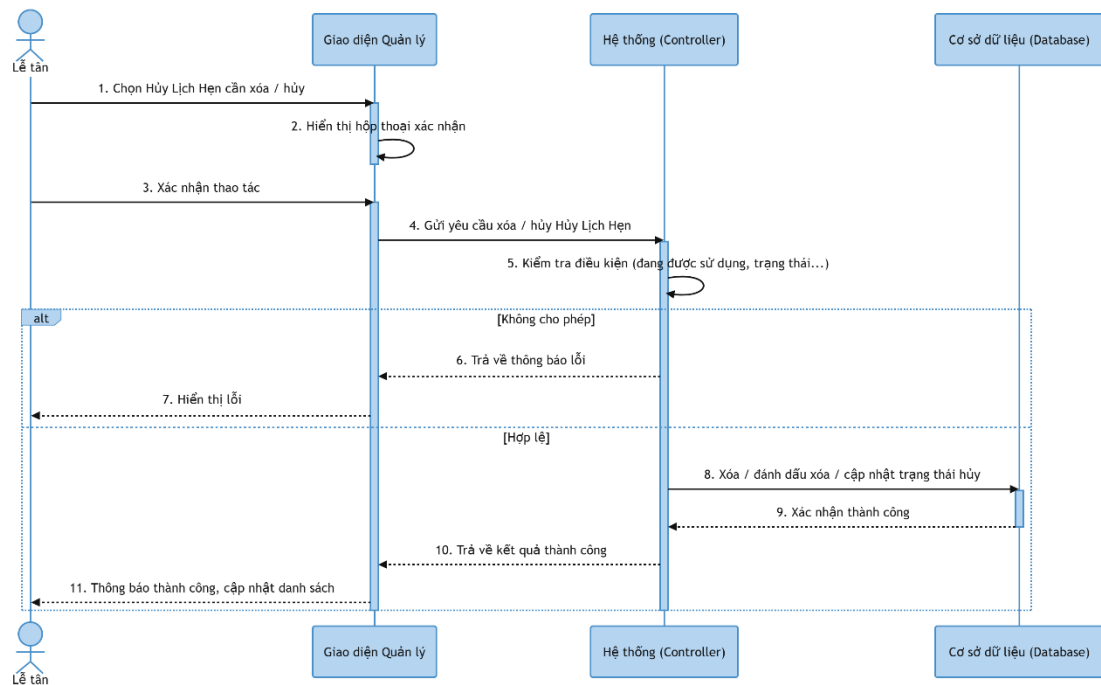
Hình 3-115: Sơ đồ tuần tự hủy lịch hẹn
