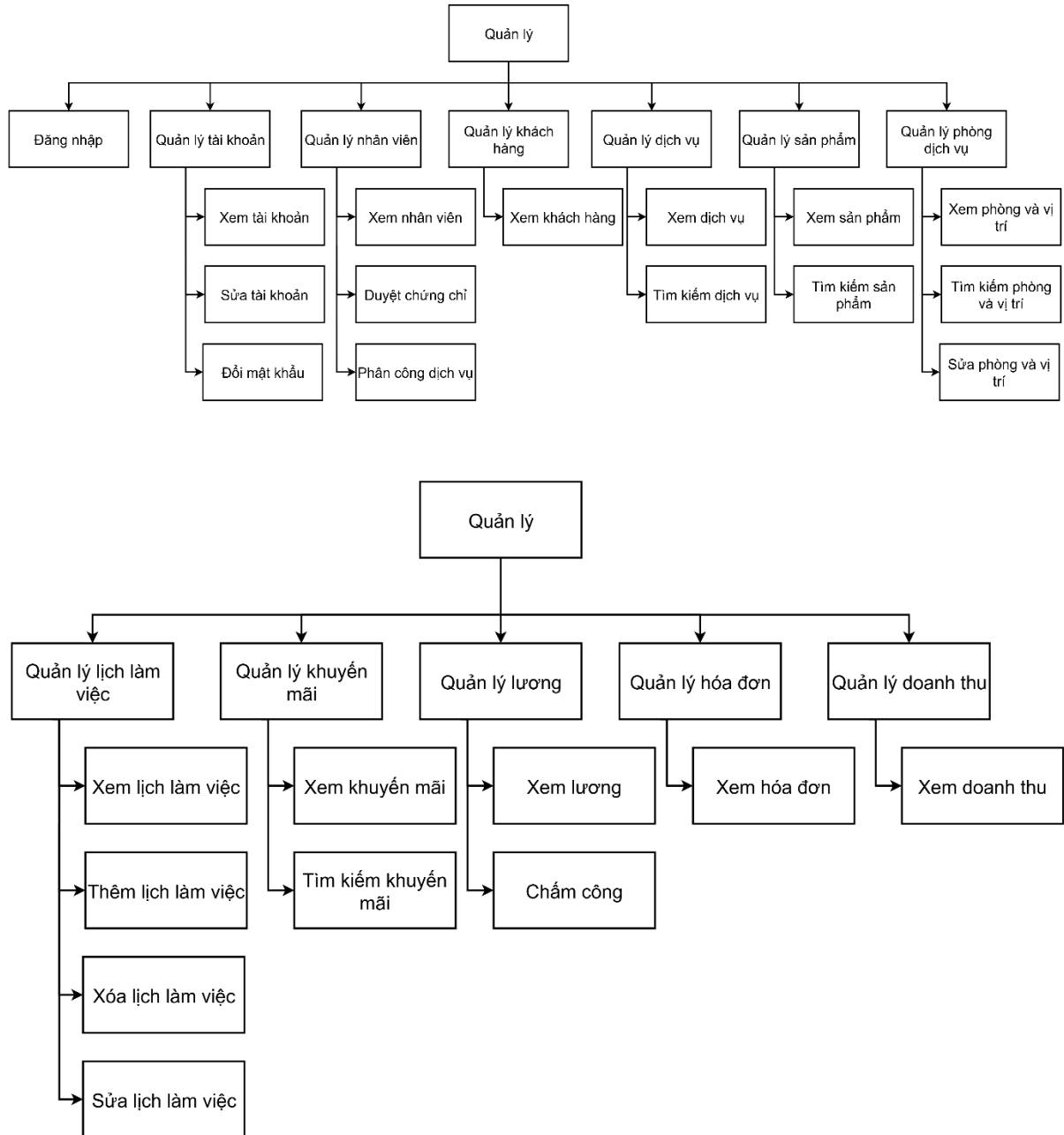
Hình 2-40: Sơ đồ chức năng của quản lý
