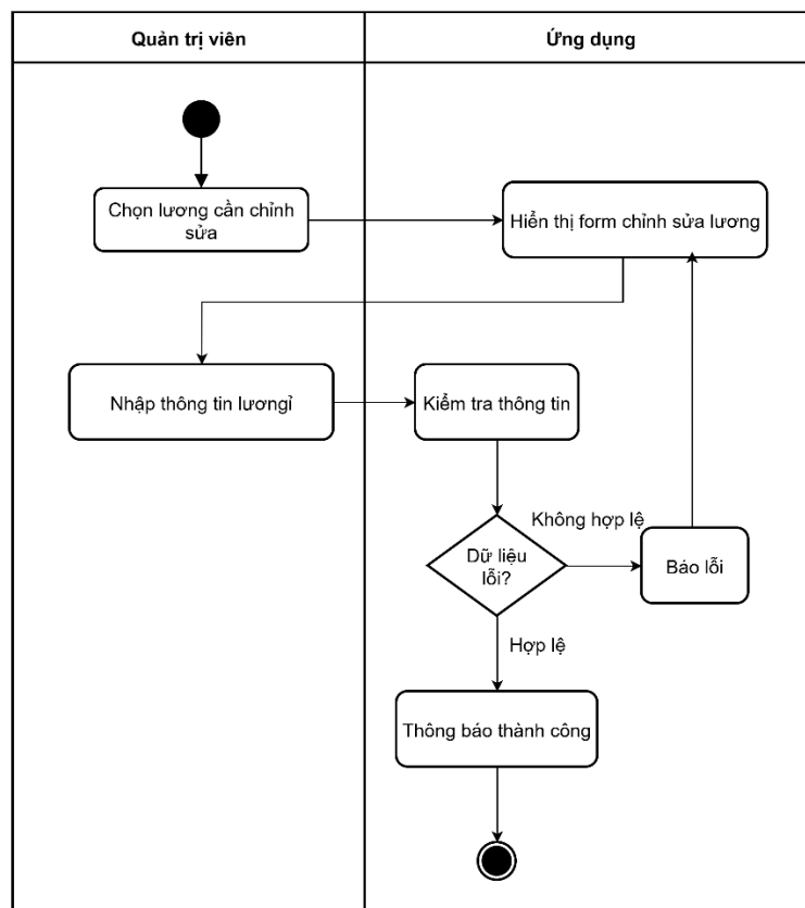
Hình 3-181: Sơ đồ hoạt động chỉnh sửa lương
