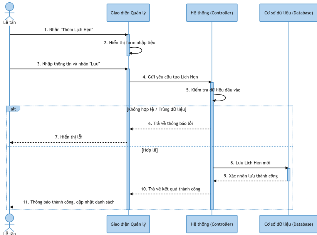
Hình 3-112: Sơ đồ tuần tự tạo lịch hẹn của lễ tân
