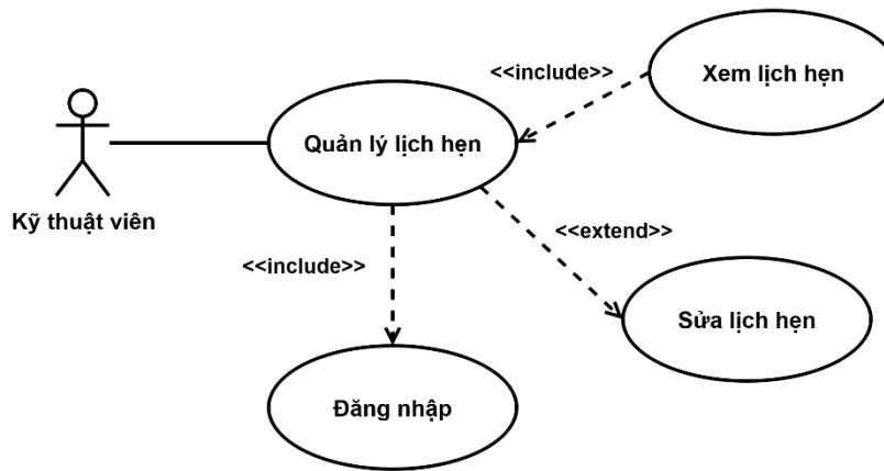
Hình 3-27: Sơ đồ use case quản lý lịch hẹn của kỹ thuật viên
