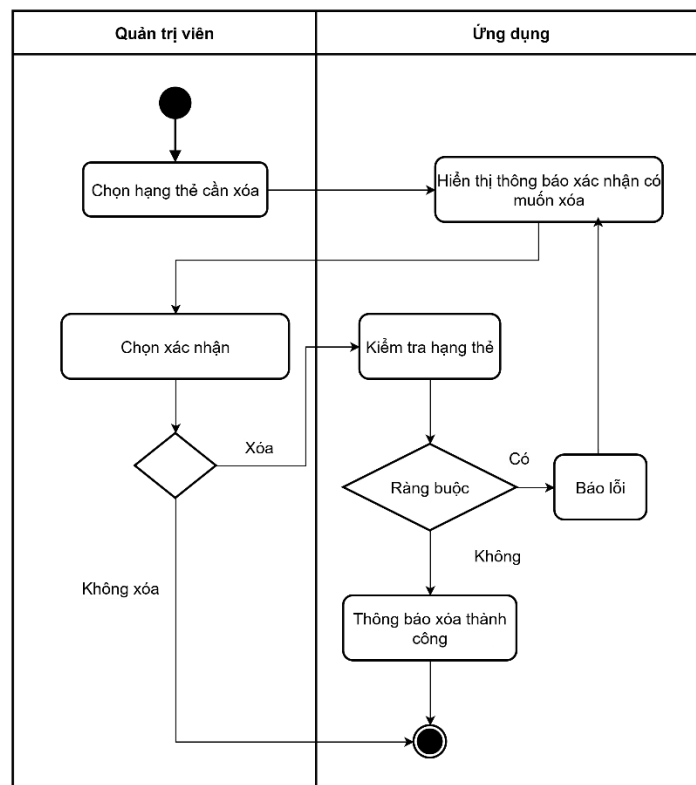
Hình 3-195: Sơ đồ hoạt động xóa hạng thẻ thành viên
