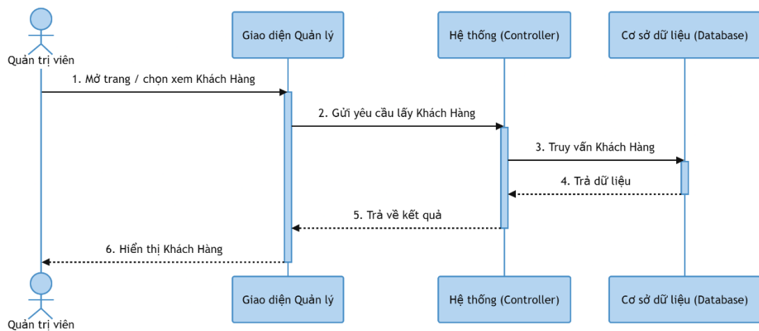
Hình 3-61: Sơ đồ tuần tự xem danh sách khách hàng
