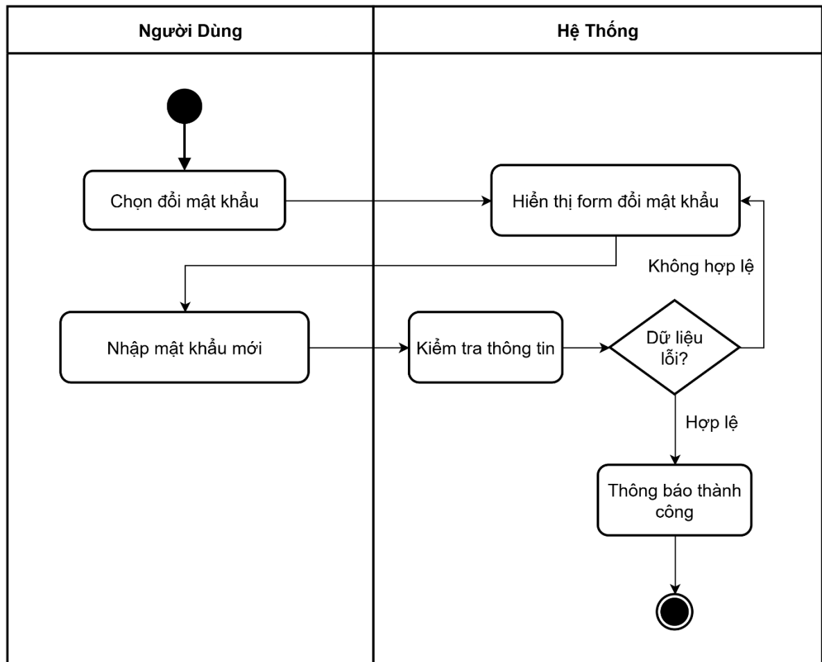
Hình 3-136: Sơ đồ hoạt động đổi mật khẩu
