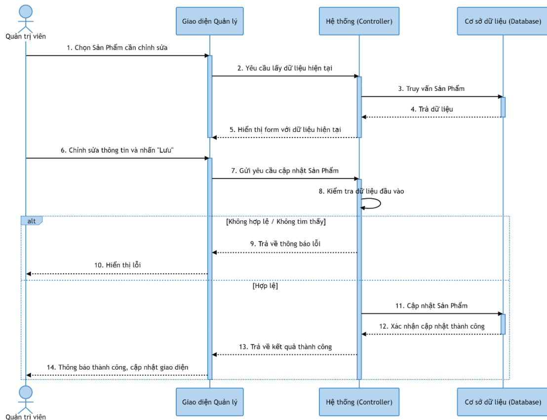
Hình 3-91: Sơ đồ tuần tự chỉnh sửa sản phẩm
