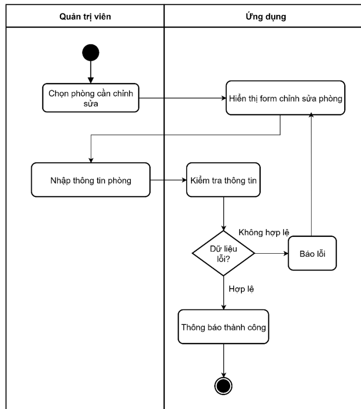
Hình 3-166: Sơ đồ hoạt động chỉnh sửa phòng
