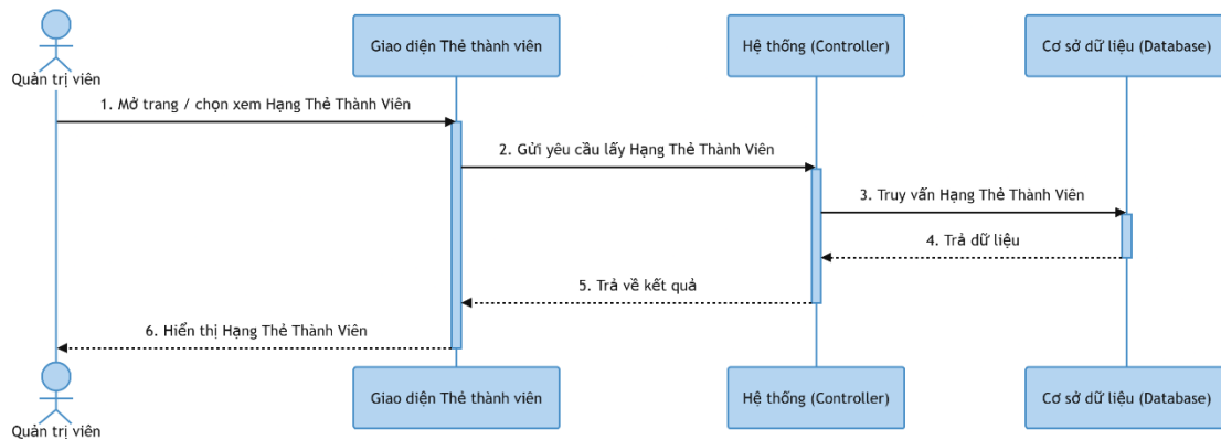
Hình 3-96: Sơ đồ tuần tự xem hạng thẻ thành viên
