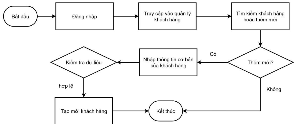
Hình 2-14: Sơ đồ quản lý khách hàng của lễ tân
