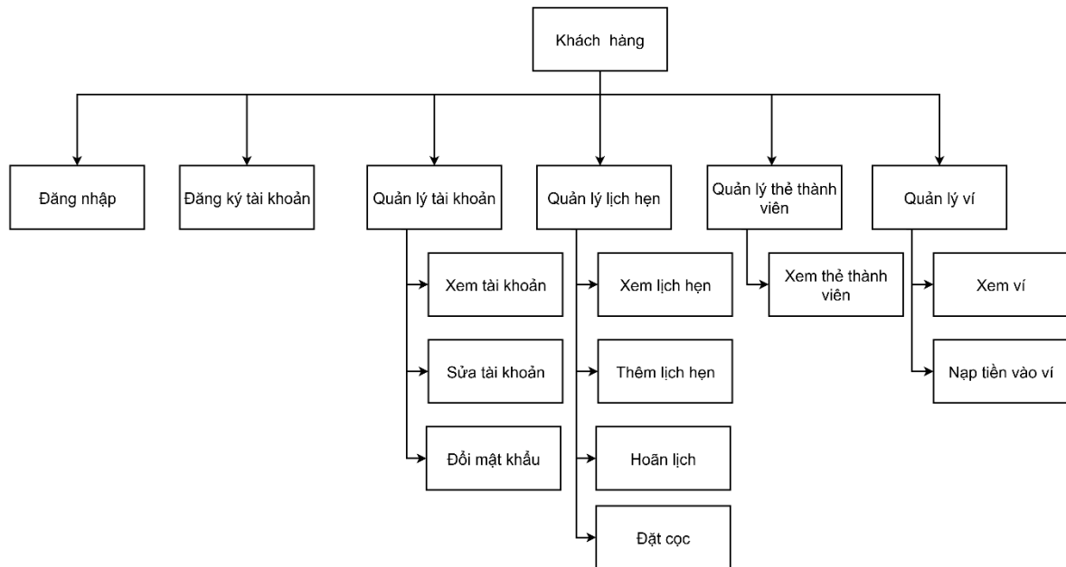
Hình 2-38: Sơ đồ chức năng của khách hàng
