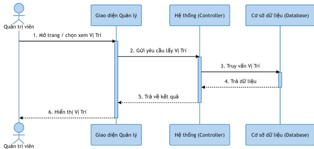
Hình 3-85: Sơ đồ tuần tự xem vị trí
