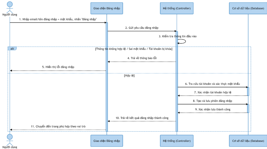
Hình 3-38: Sơ đồ tuần tự chức năng đăng nhập
