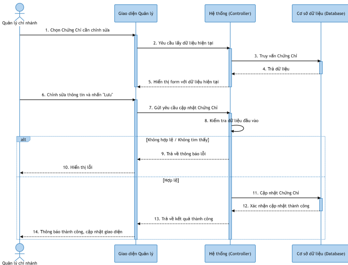
Hình 3-49: Sơ đồ tuần tự sửa chứng chỉ
