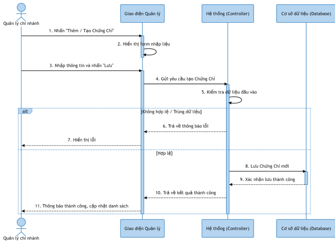
Hình 3-48: Sơ đồ tuần tự tạo chứng chỉ
