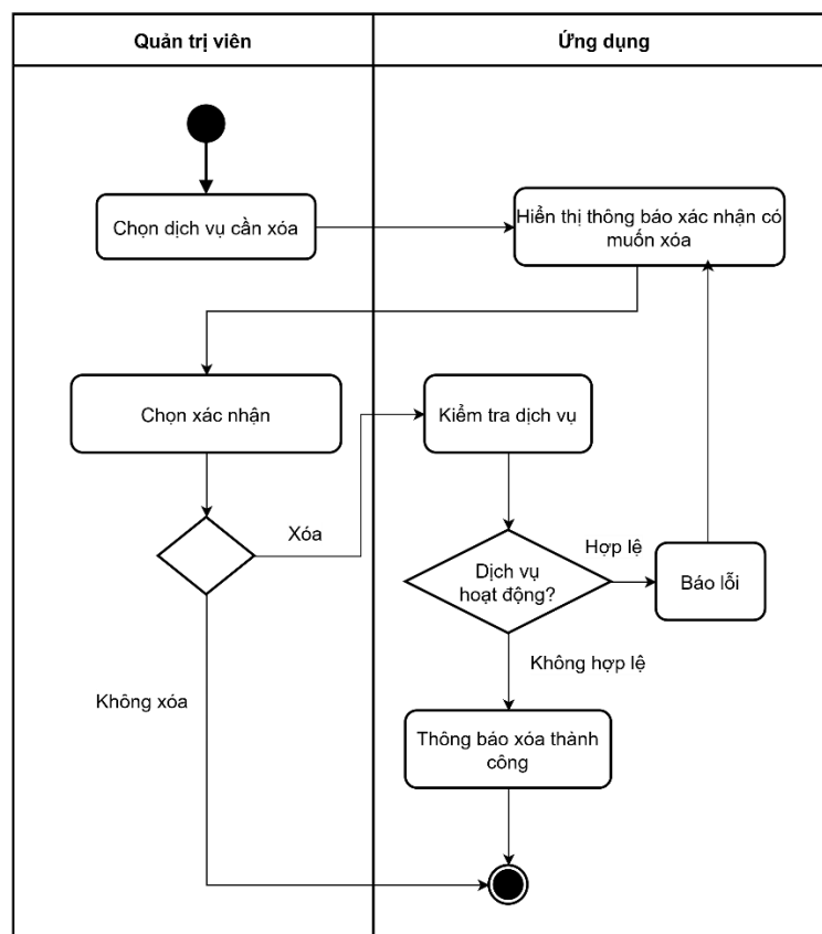
Hình 3-145: Sơ đồ hoạt động xóa dịch vụ
