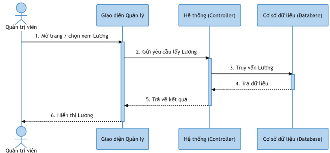
Hình 3-72: Sơ đồ tuần tự xem bảng lương
