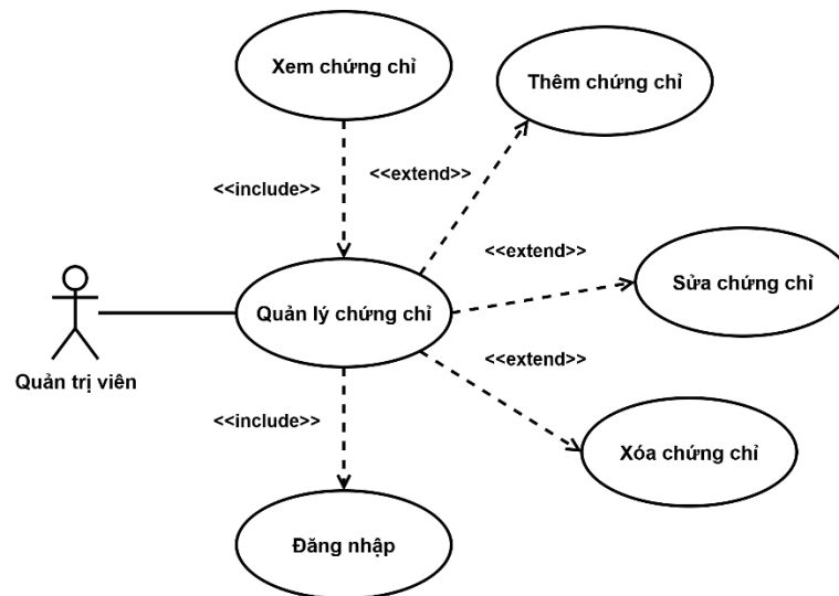
Hình 3-12: Sơ đồ use case chi tiết quản lý chứng chỉ của quản trị viên
