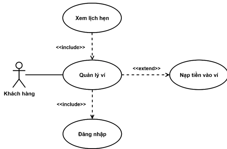
Hình 3-37: Sơ đồ use case chi tiết quản lý ví
