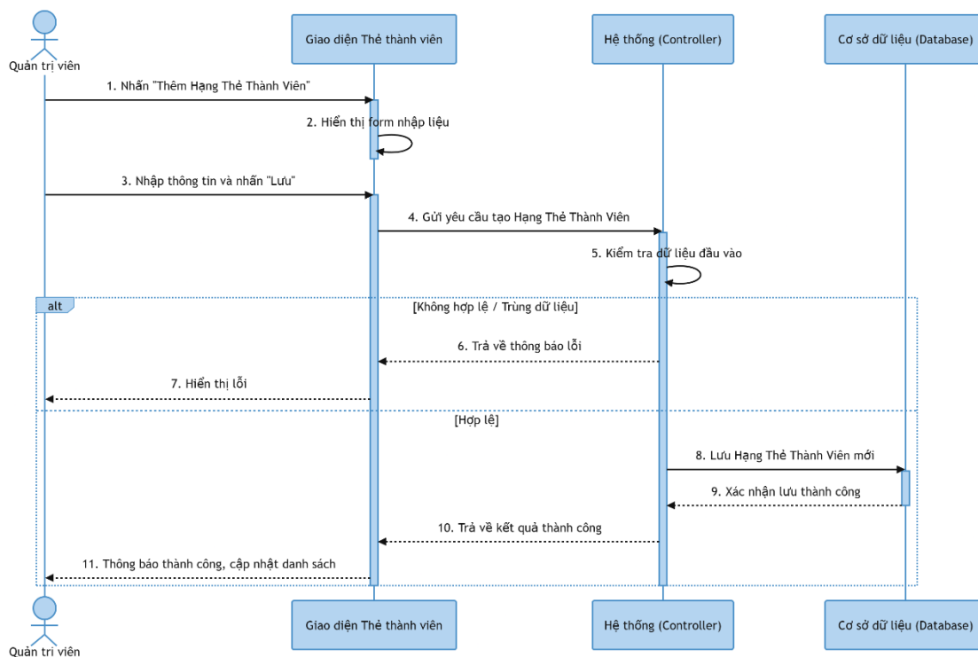
Hình 3-97: Sơ đồ tuần tự thêm hạng thẻ thành viên
