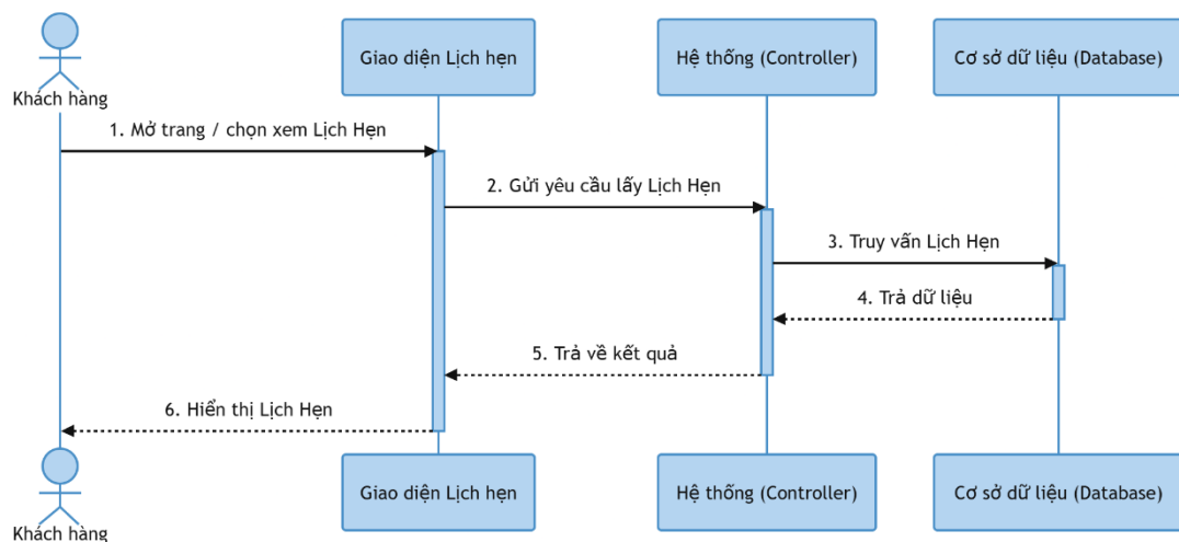
Hình 3-126: Sơ đồ tuần tự xem lịch hẹn
