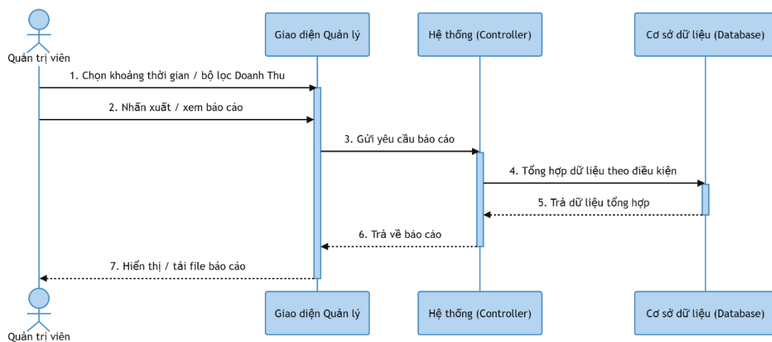
Hình 3-57: Sơ đồ tuần tự xuất báo cáo
