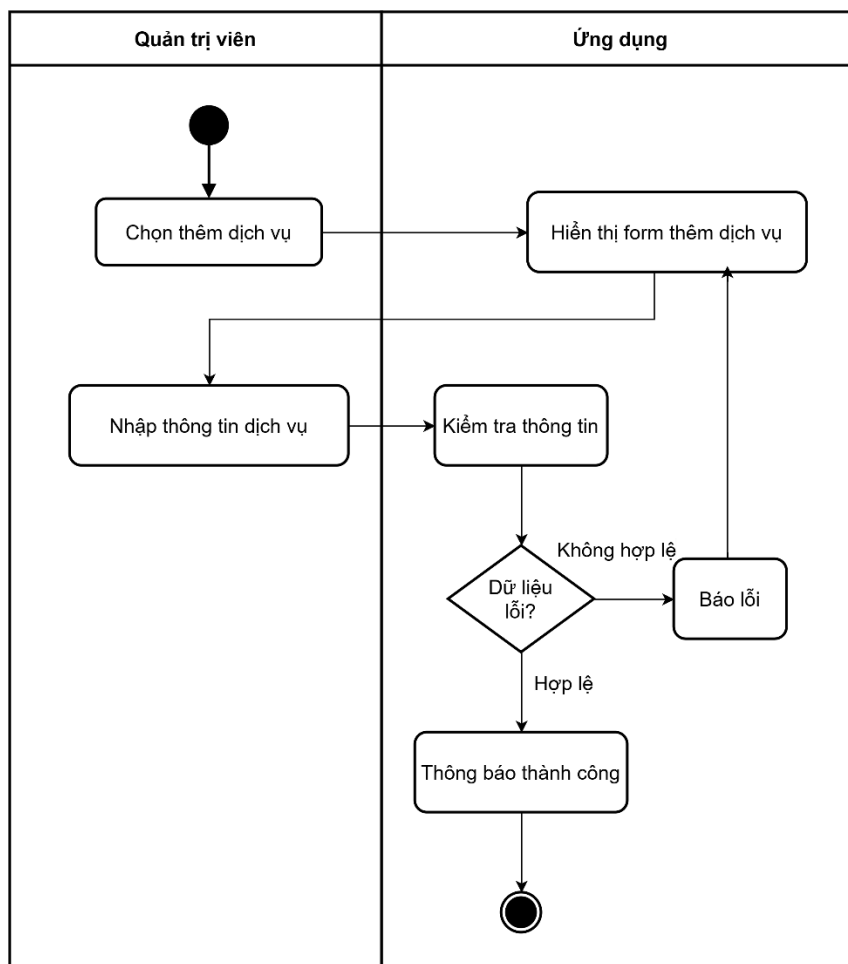
Hình 3-143: Sơ đồ hoạt động thêm dịch vụ
