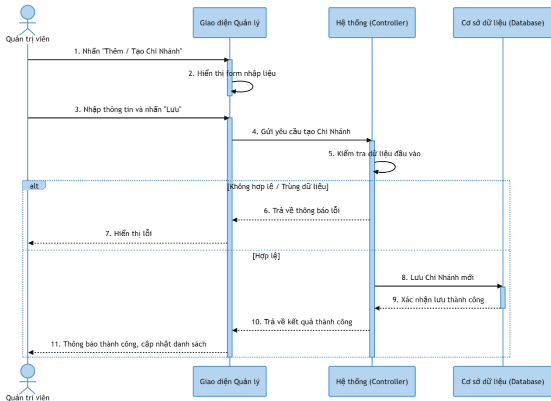
Hình 3-44: Sơ đồ tuần tự tạo chi nhánh
