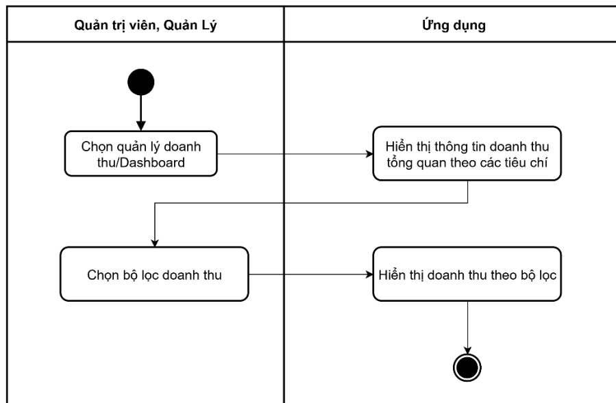
Hình 3-152: Sơ đồ hoạt động xem doanh thu
