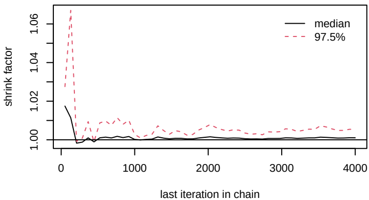
alpha0[7]
