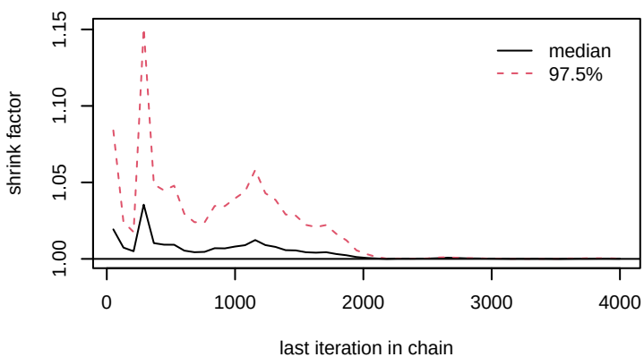
lambda0[9]
