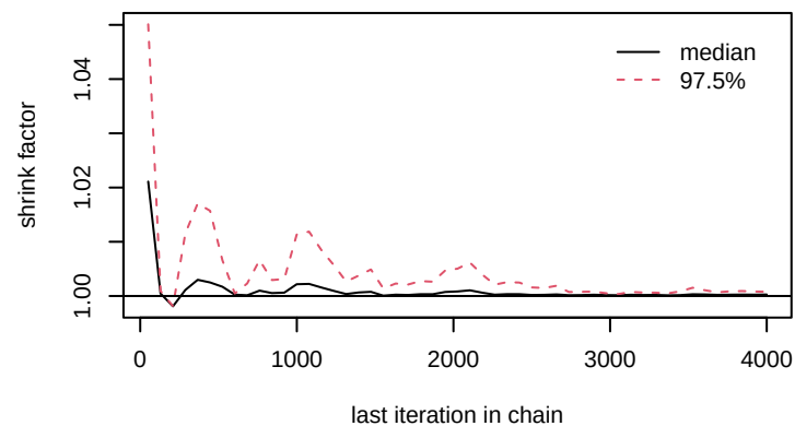
gamma[1,7]
