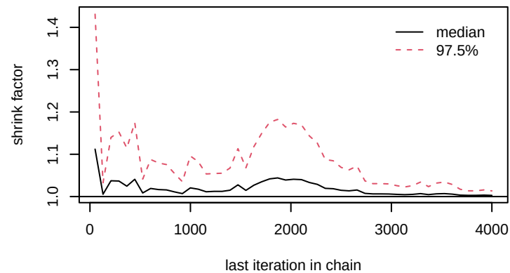
beta_long[7]
