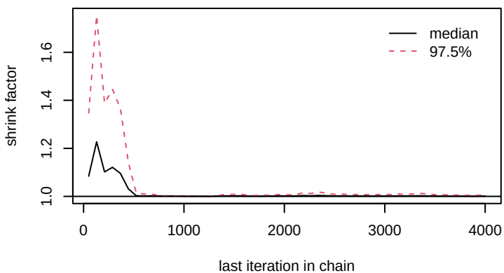
alpha0[4]
