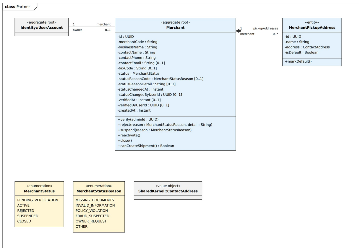
Hình 4.28. Sơ đồ lớp – Partner
