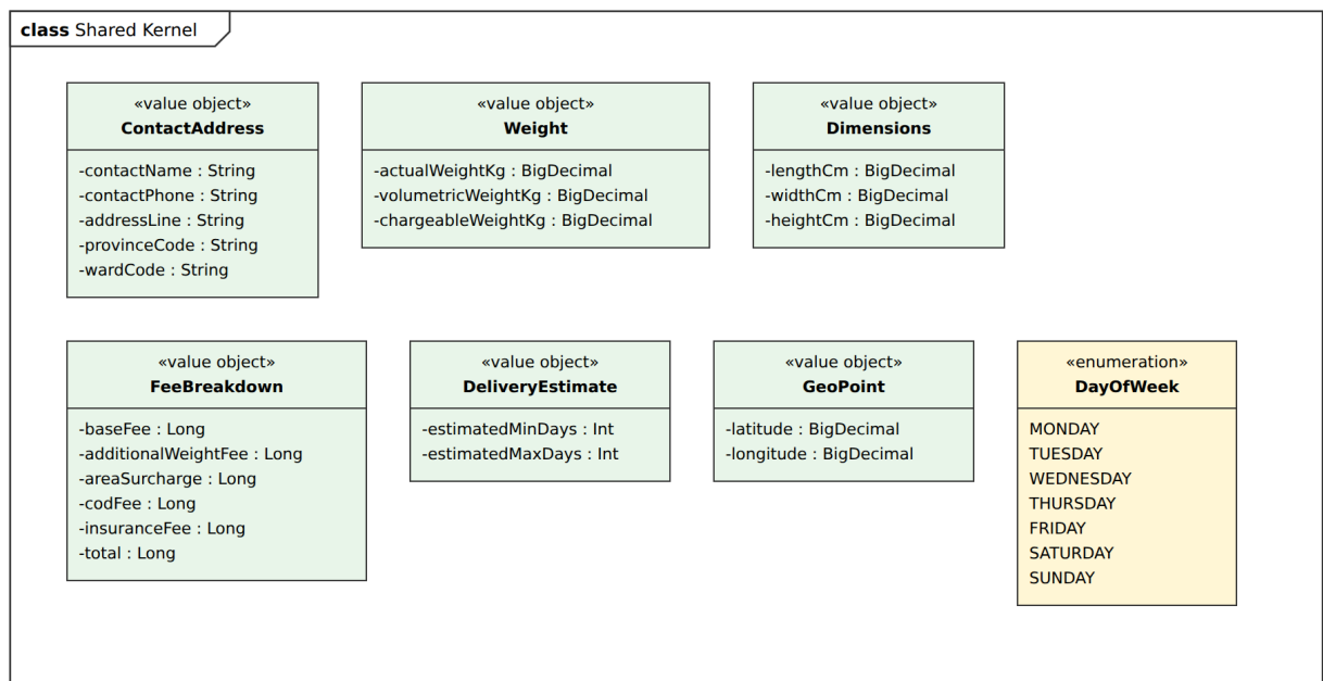
Hình 4.35. Sơ đồ lớp – Shared Kernel
