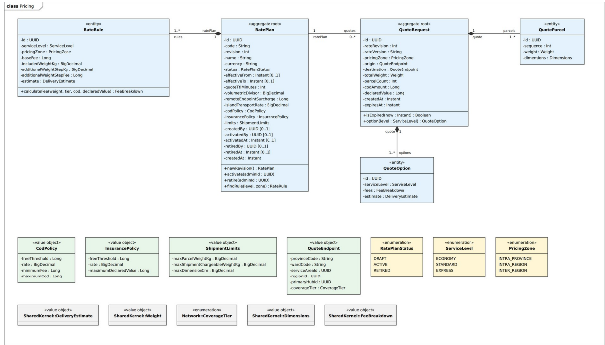
Hình 4.31. Sơ đồ lớp – Pricing
