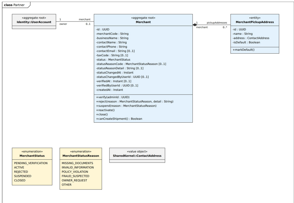
Hình 4.29. Sơ đồ lớp – Partner
