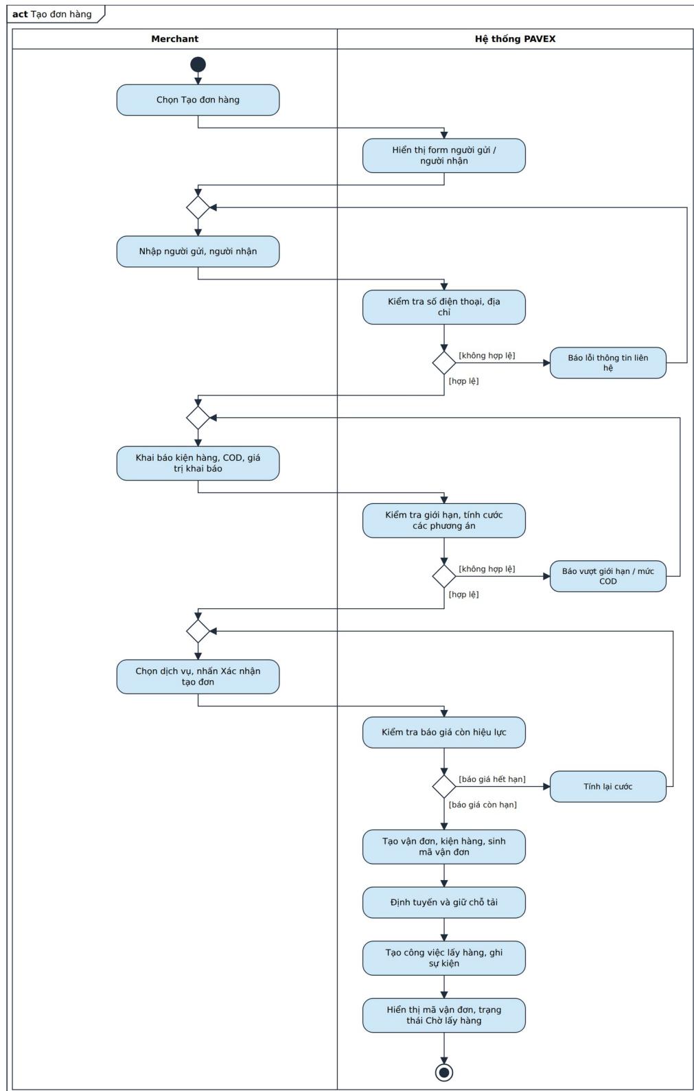
Hình 4.8. Sơ đồ hoạt động – Tạo đơn hàng
