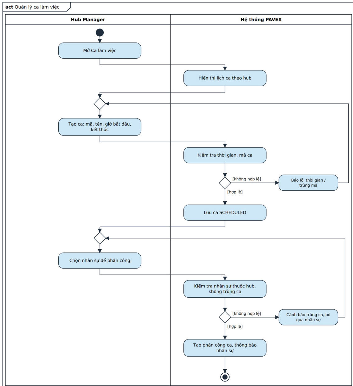
Hình 4.18. Sơ đồ hoạt động – Quản lý ca làm việc
