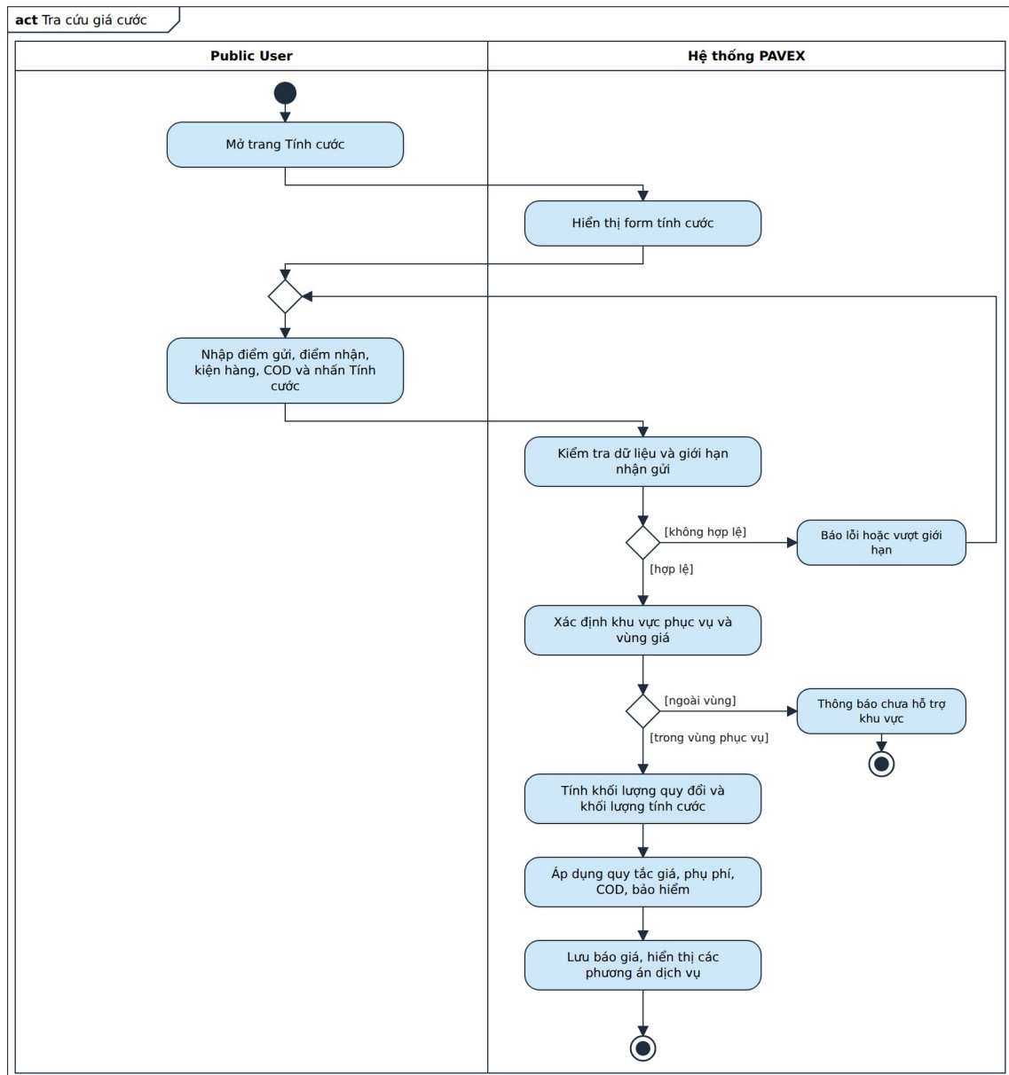
Hình 4.6. Sơ đồ hoạt động – Tra cứu giá cước
