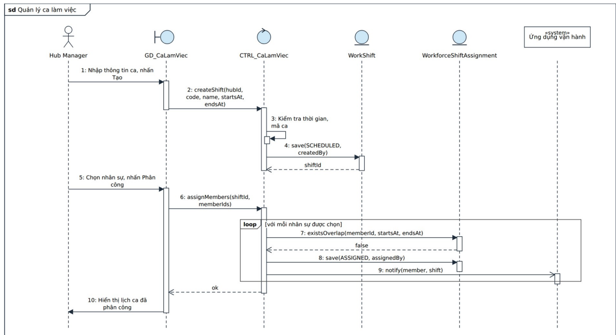
Hình 4.19. Sơ đồ tuần tự – Quản lý ca làm việc
