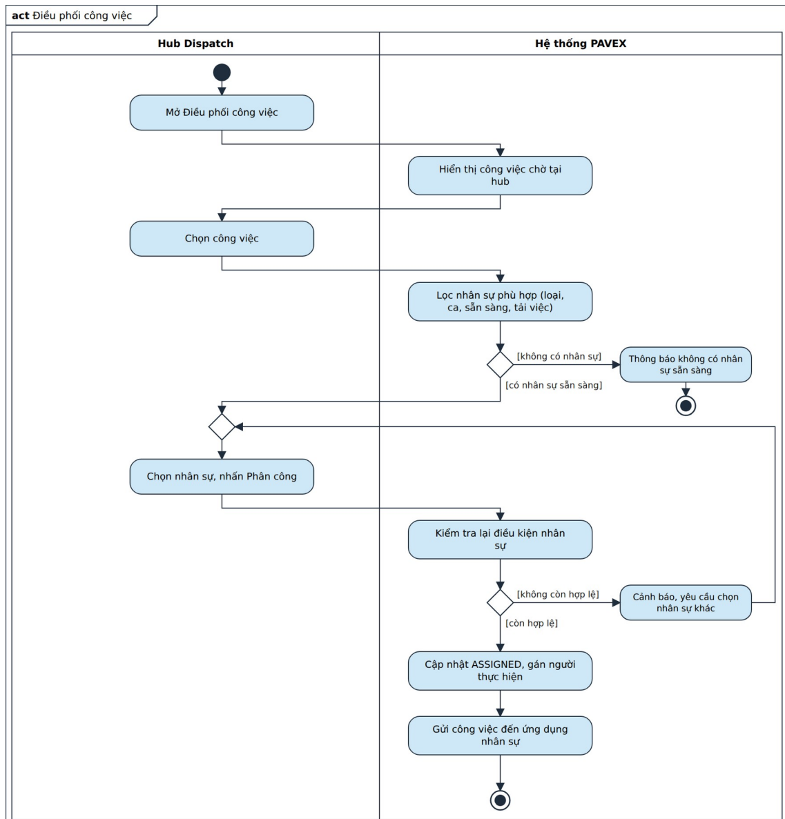
Hình 4.14. Sơ đồ hoạt động – Điều phối công việc
