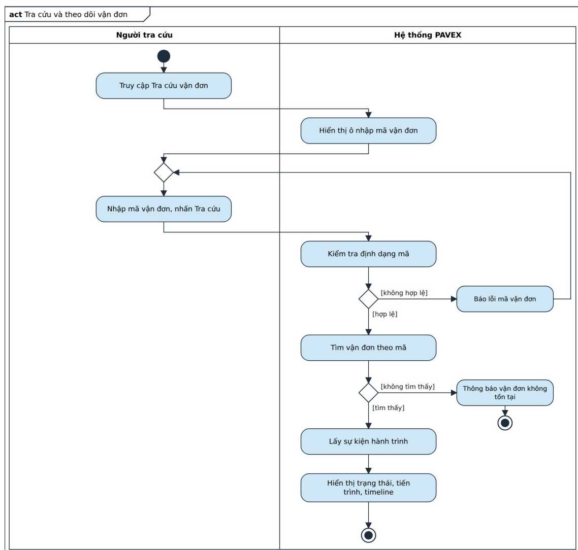
Hình 4.10. Sơ đồ hoạt động – Tra cứu và theo dõi vận đơn
