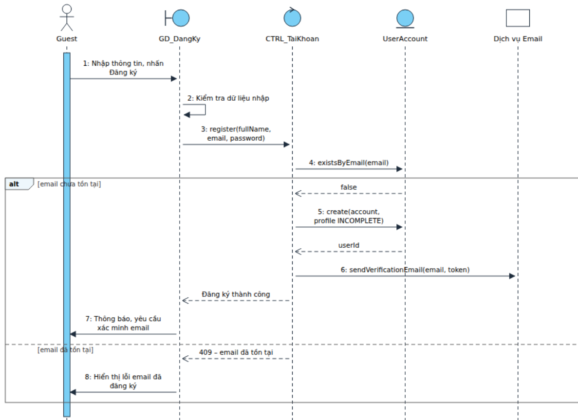
Hình 4.5. Sơ đồ tuần tự – Đăng ký tài khoản
