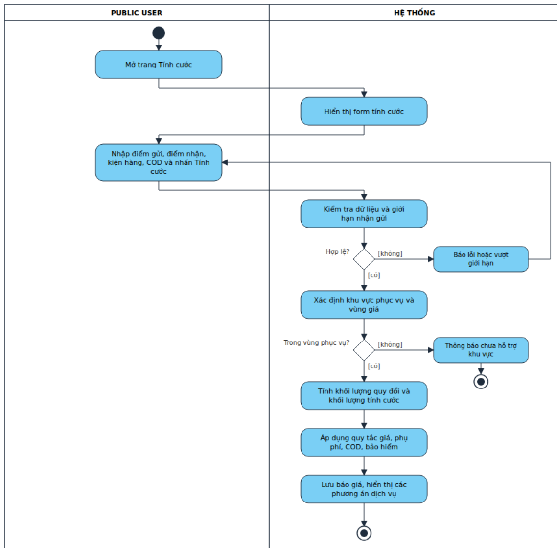
Hình 4.6. Sơ đồ hoạt động – Tra cứu giá cước
