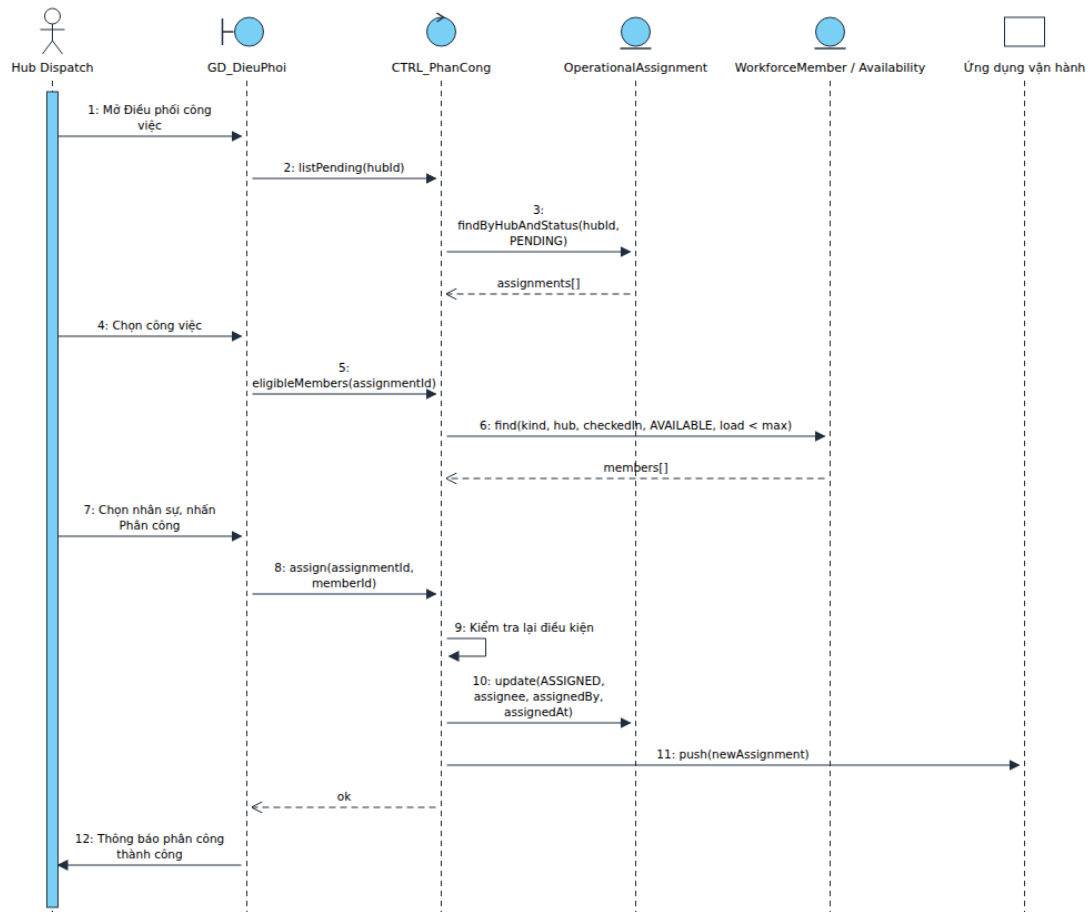
Hình 4.15. Sơ đồ tuần tự – Điều phối công việc
