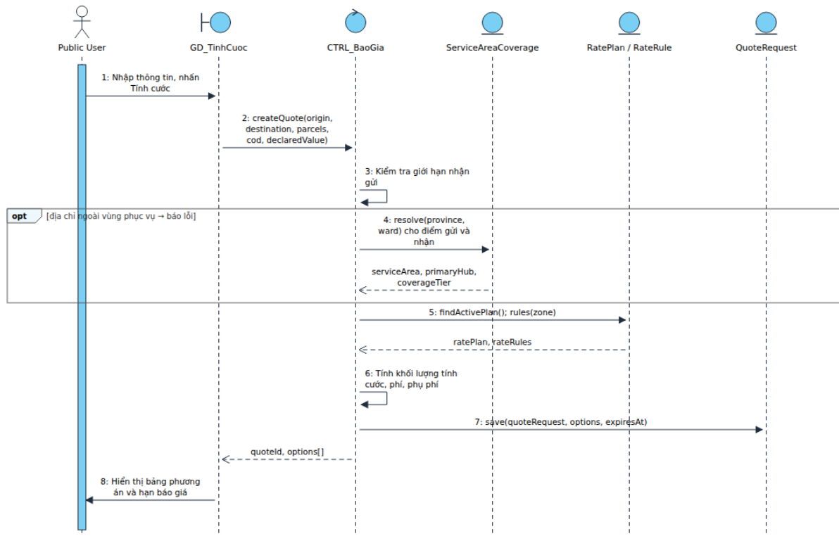
Hình 4.7. Sơ đồ tuần tự – Tra cứu giá cước
