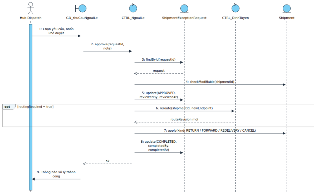
Hình 4.17. Sơ đồ tuần tự – Xử lý yêu cầu ngoại lệ
