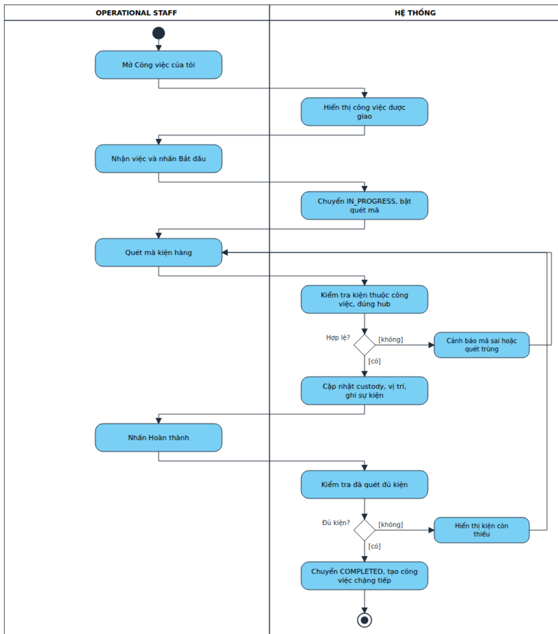
Hình 4.22. Sơ đồ hoạt động – Thực hiện công việc và quét kiện hàng
