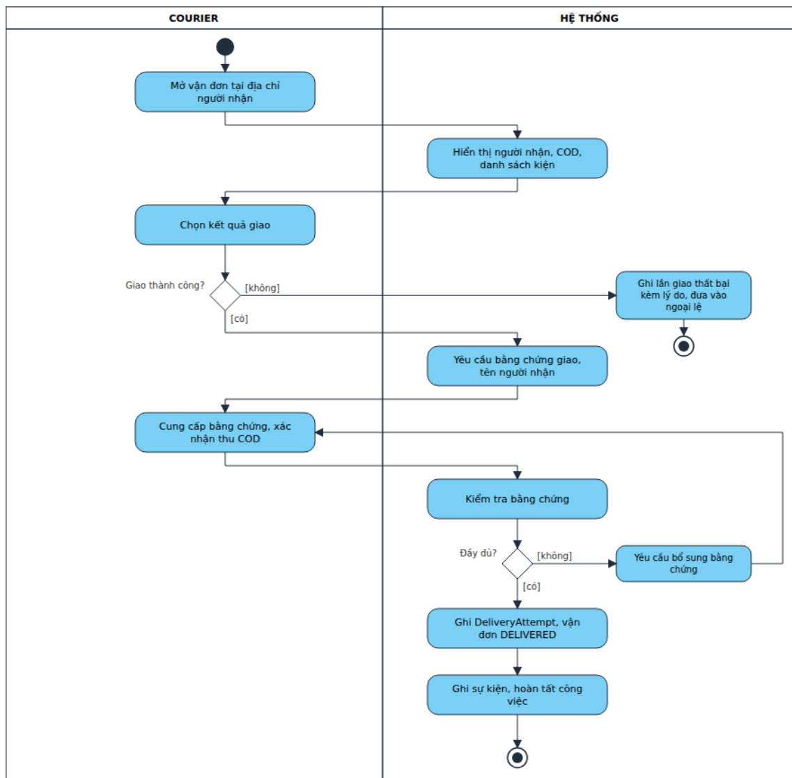
Hình 4.24. Sơ đồ hoạt động – Ghi nhận kết quả giao hàng
