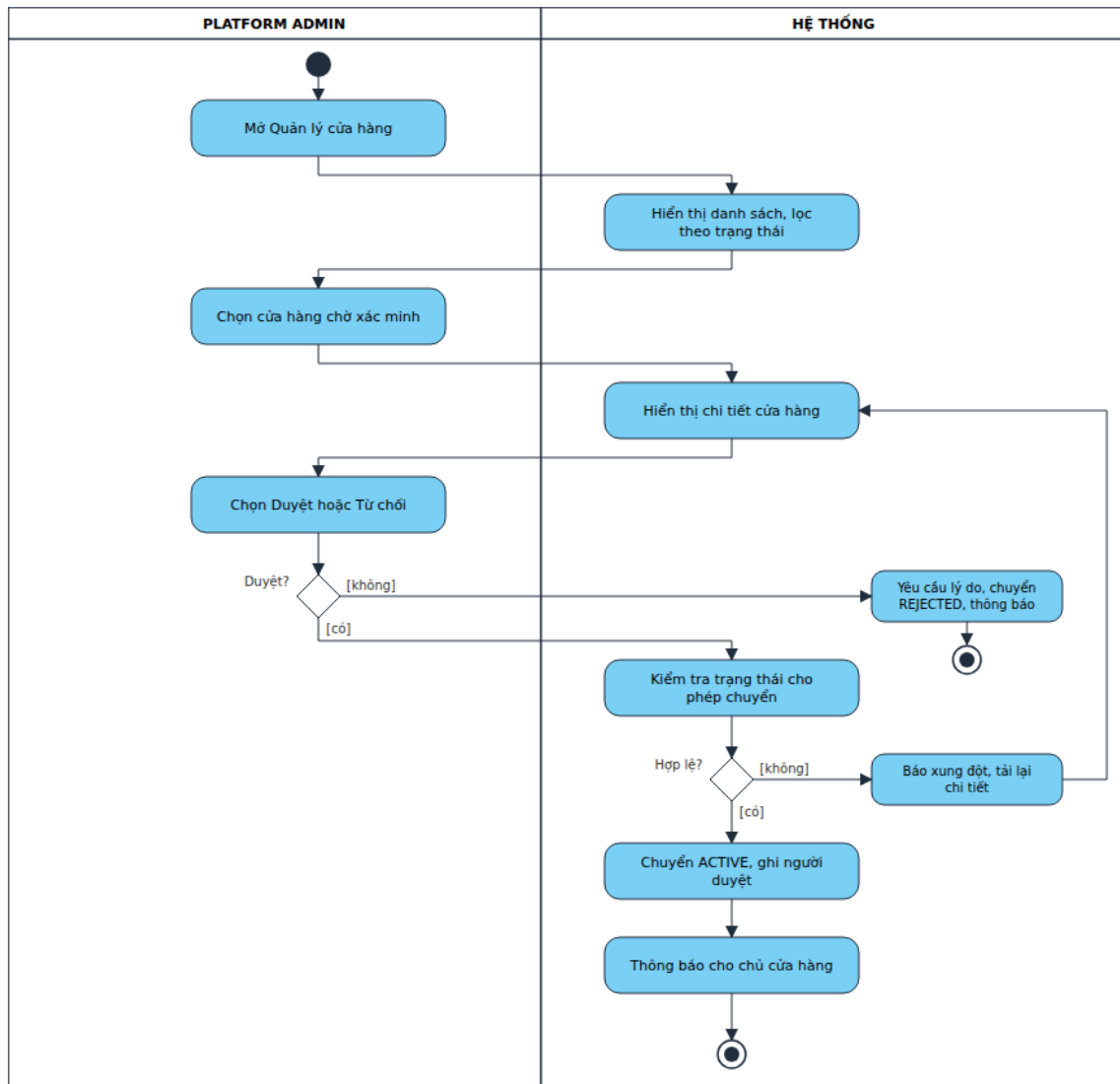
Hình 4.12. Sơ đồ hoạt động – Duyệt và quản lý cửa hàng
