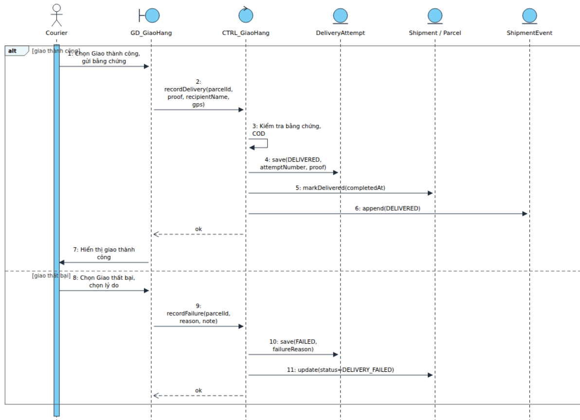
Hình 4.25. Sơ đồ tuần tự – Ghi nhận kết quả giao hàng
