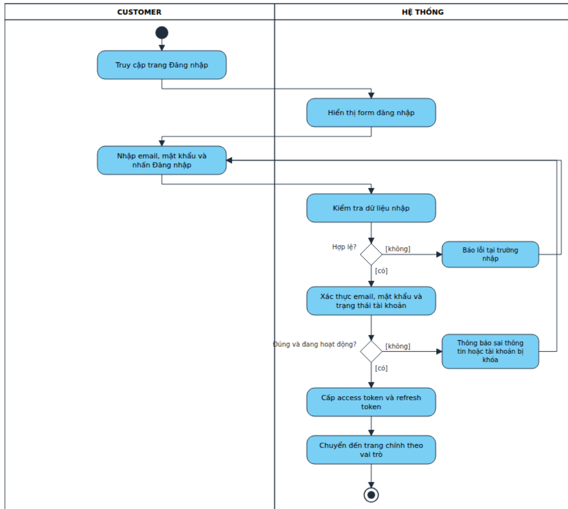
Hình 4.2. Sơ đồ hoạt động – Đăng nhập
