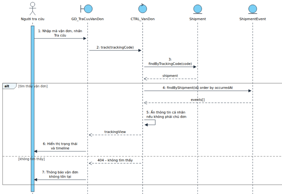
Hình 4.11. Sơ đồ tuần tự – Tra cứu và theo dõi vận đơn
