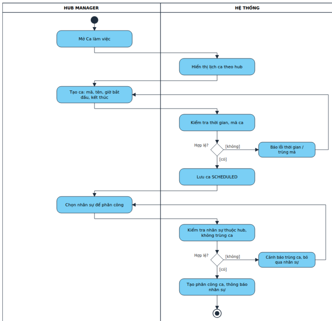
Hình 4.18. Sơ đồ hoạt động – Quản lý ca làm việc
