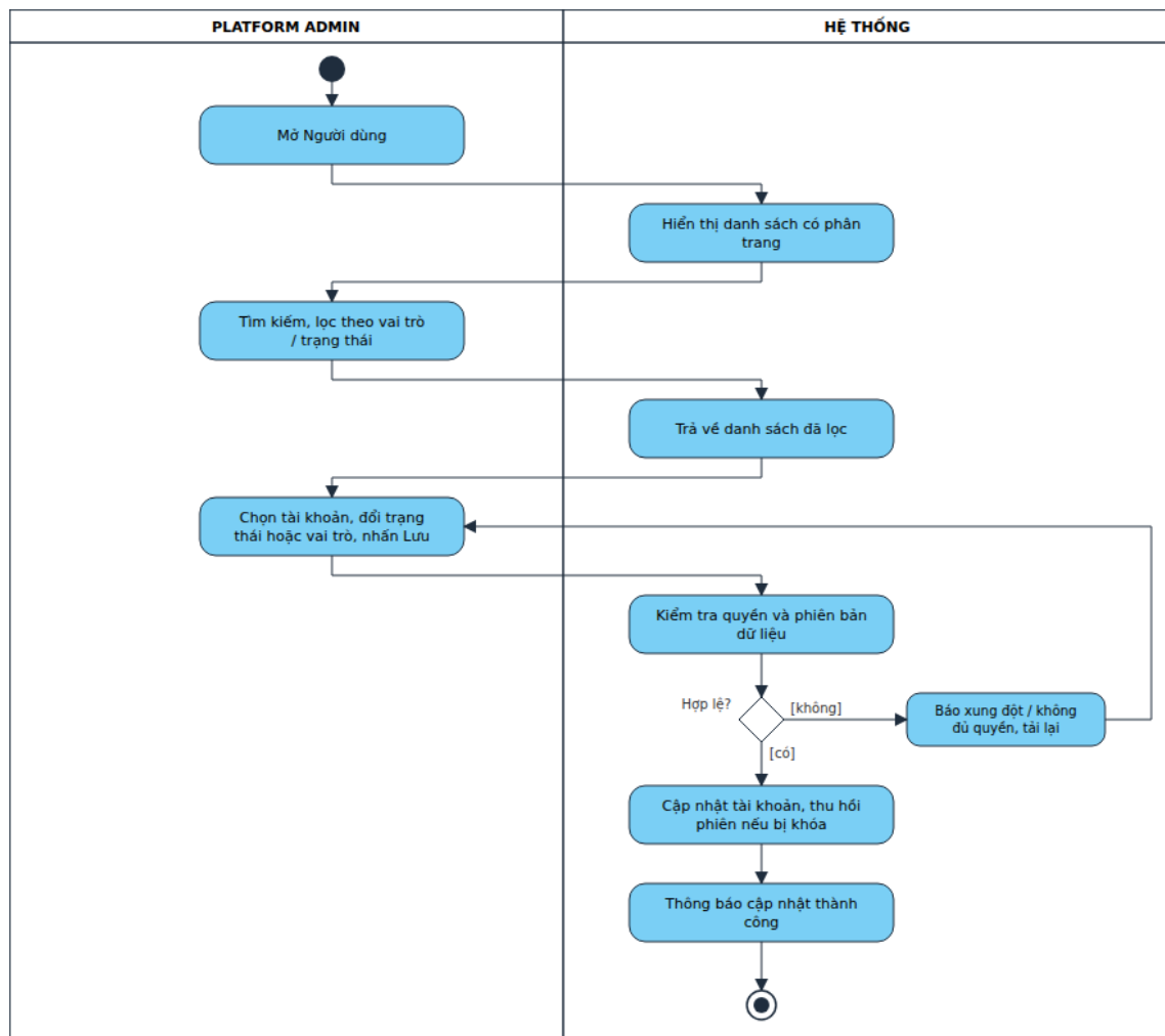
Hình 4.20. Sơ đồ hoạt động – Quản lý người dùng và phân quyền
