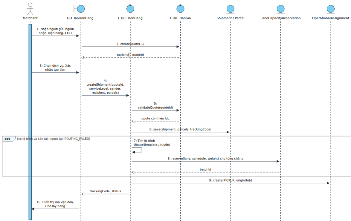
Hình 4.9. Sơ đồ tuần tự – Tạo đơn hàng
