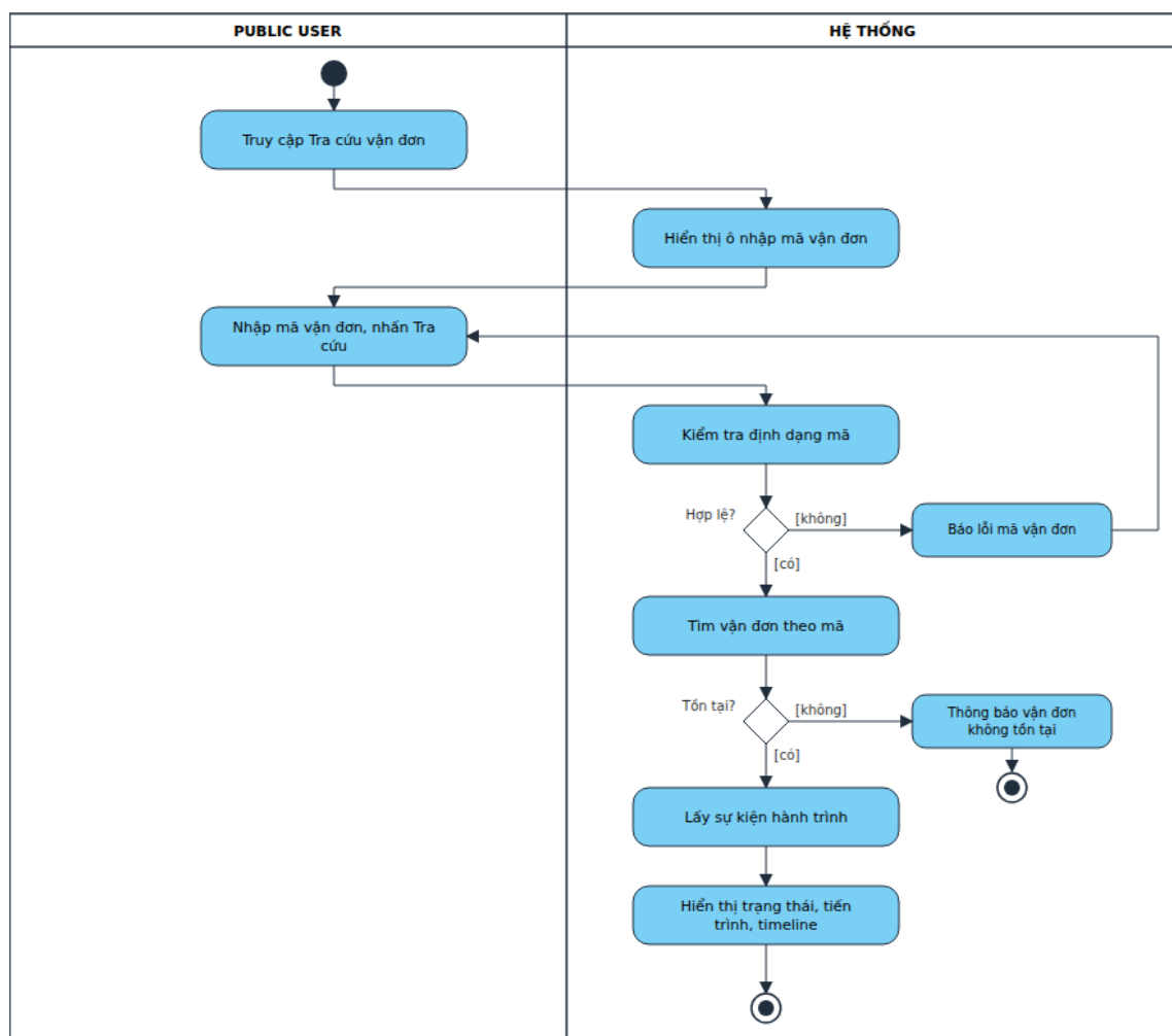
Hình 4.10. Sơ đồ hoạt động – Tra cứu và theo dõi vận đơn
