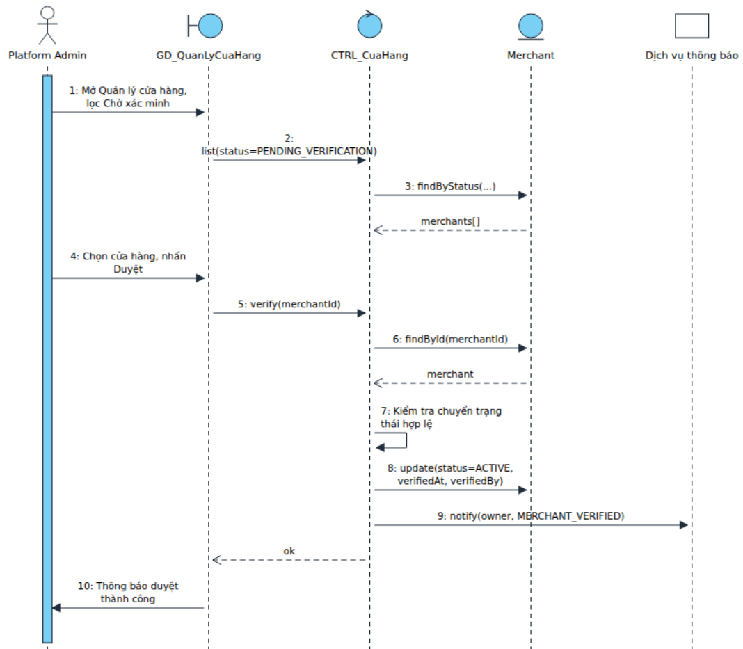
Hình 4.13. Sơ đồ tuần tự – Duyệt và quản lý cửa hàng
