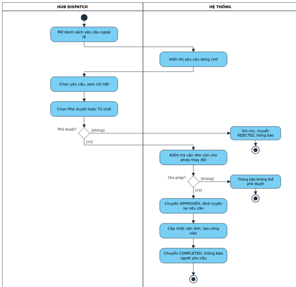
Hình 4.16. Sơ đồ hoạt động – Xử lý yêu cầu ngoại lệ
