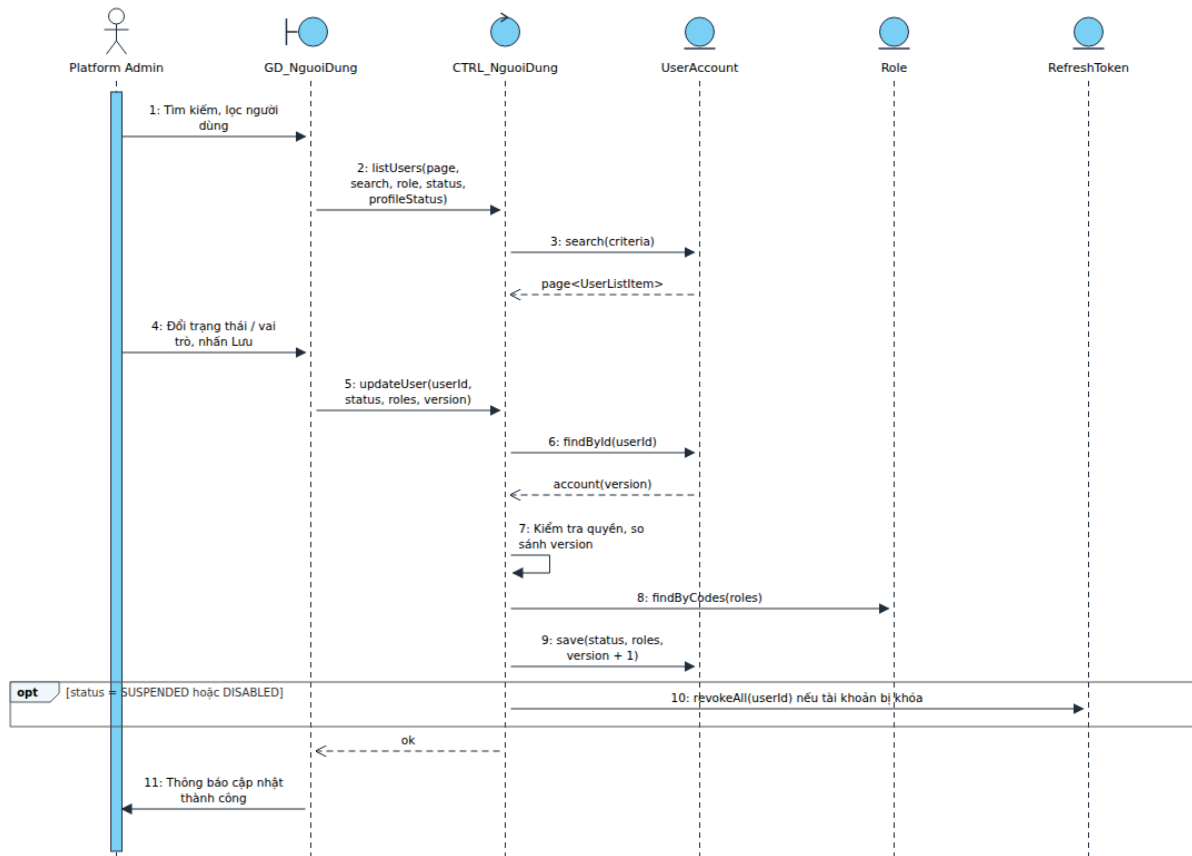
Hình 4.21. Sơ đồ tuần tự – Quản lý người dùng và phân quyền
