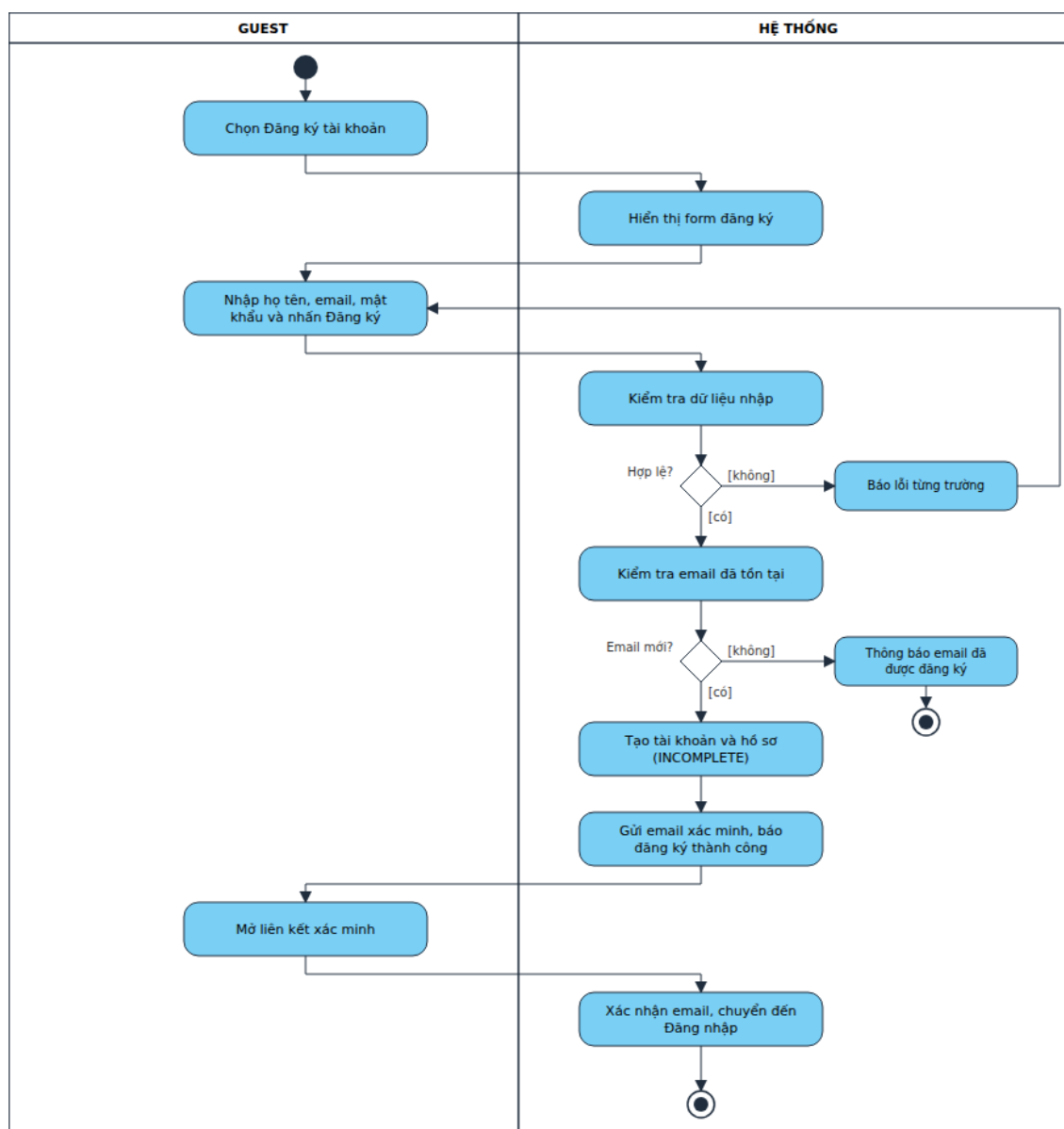
Hình 4.4. Sơ đồ hoạt động – Đăng ký tài khoản
