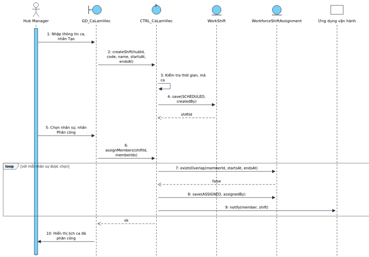
Hình 4.19. Sơ đồ tuần tự – Quản lý ca làm việc
