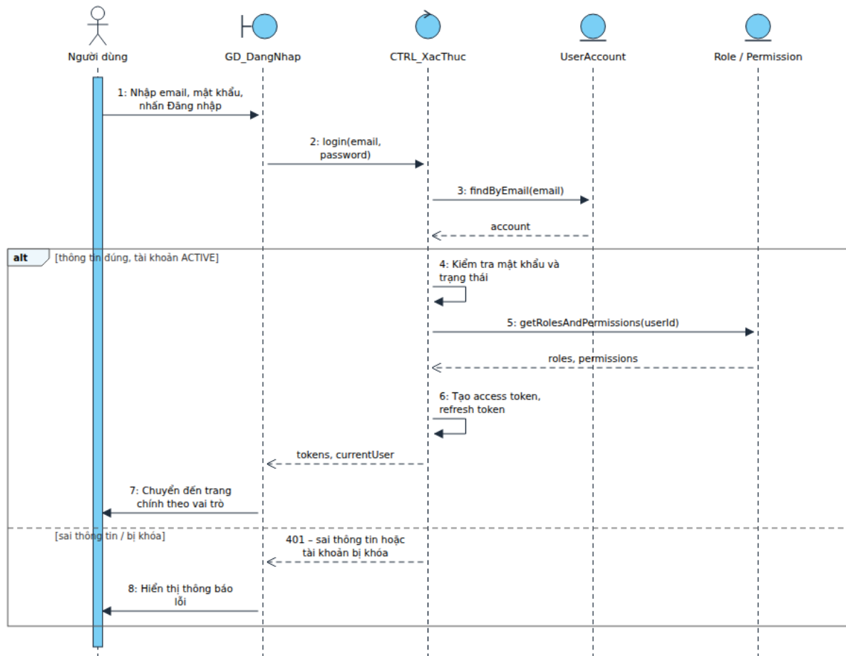
Hình 4.3. Sơ đồ tuần tự – Đăng nhập
