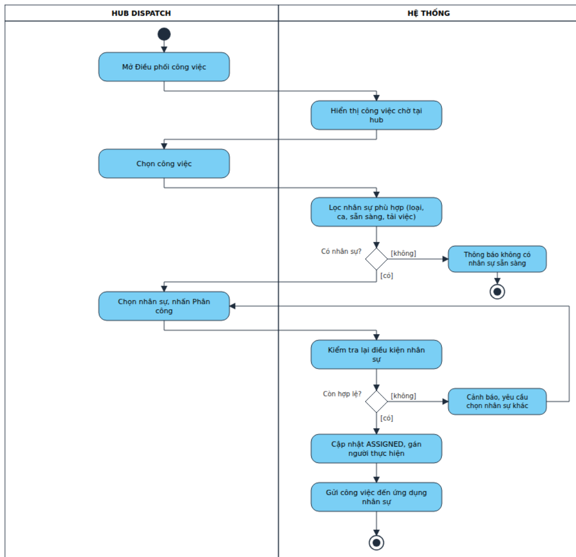
Hình 4.14. Sơ đồ hoạt động – Điều phối công việc
