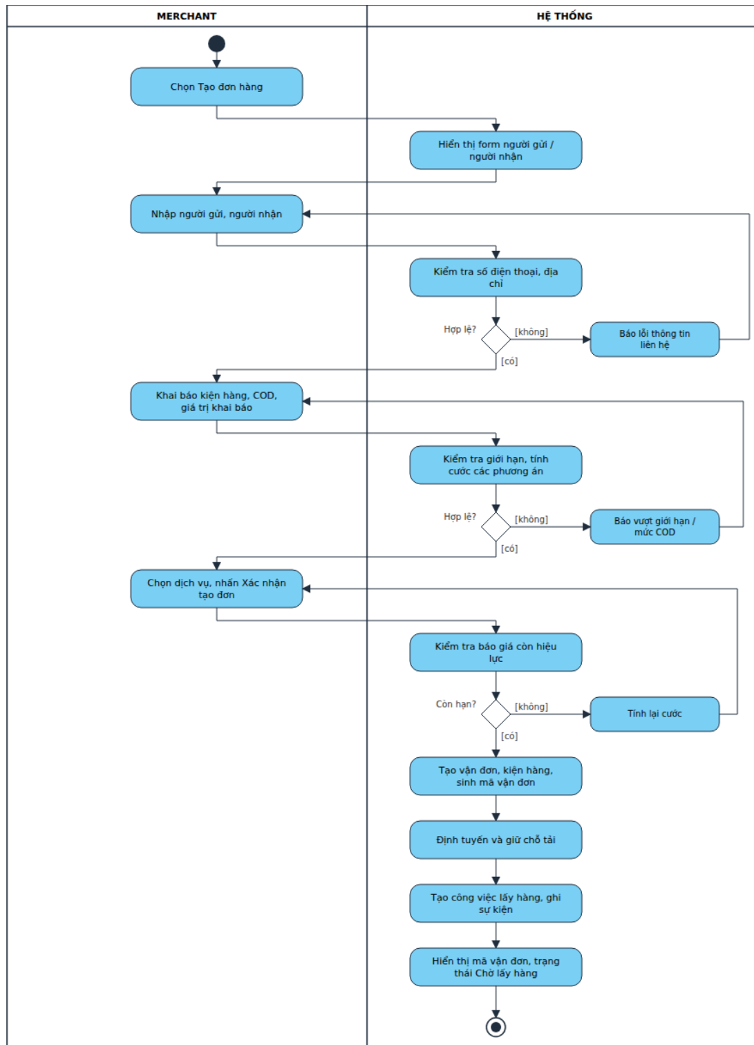
Hình 4.8. Sơ đồ hoạt động – Tạo đơn hàng
