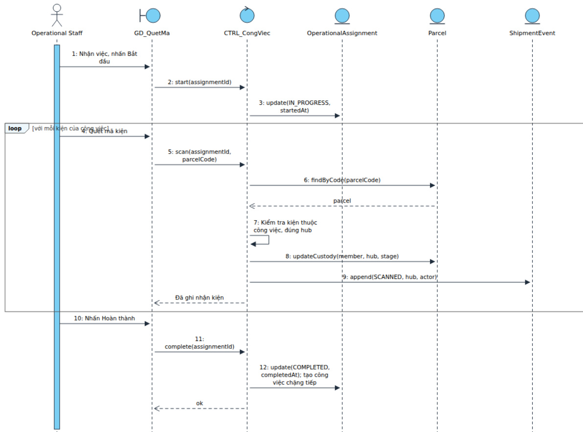
Hình 4.23. Sơ đồ tuần tự – Thực hiện công việc và quét kiện hàng
