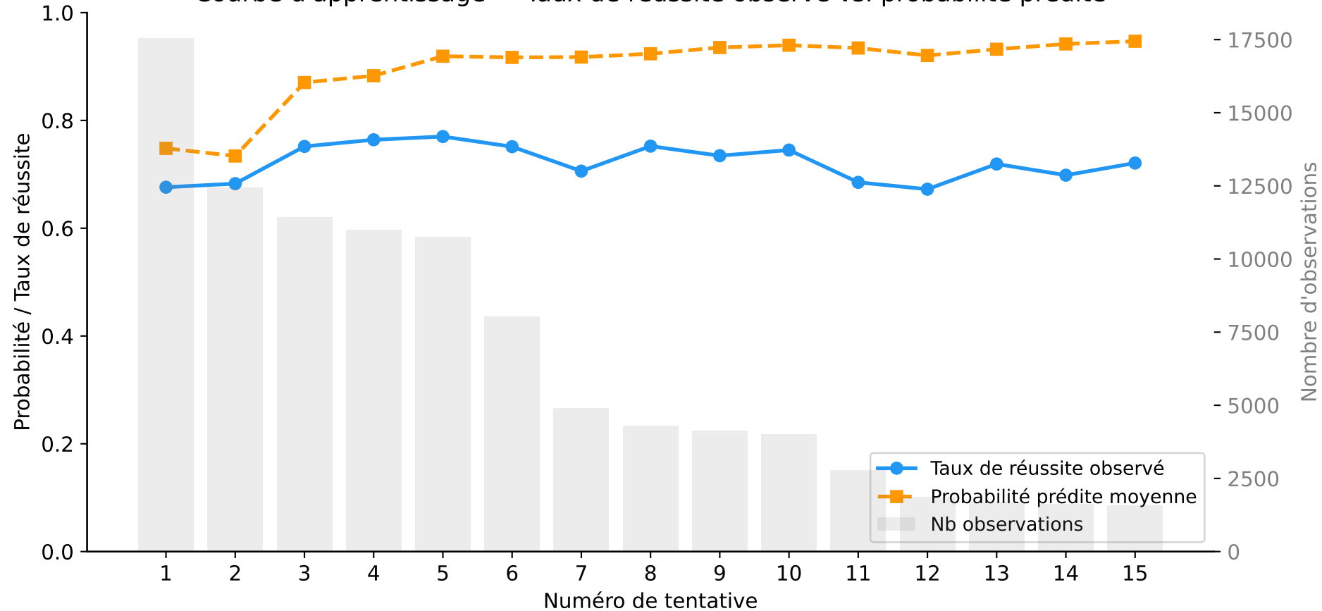
Courbe d'apprentissage — Taux de réussite observé vs. probabilité prédite
