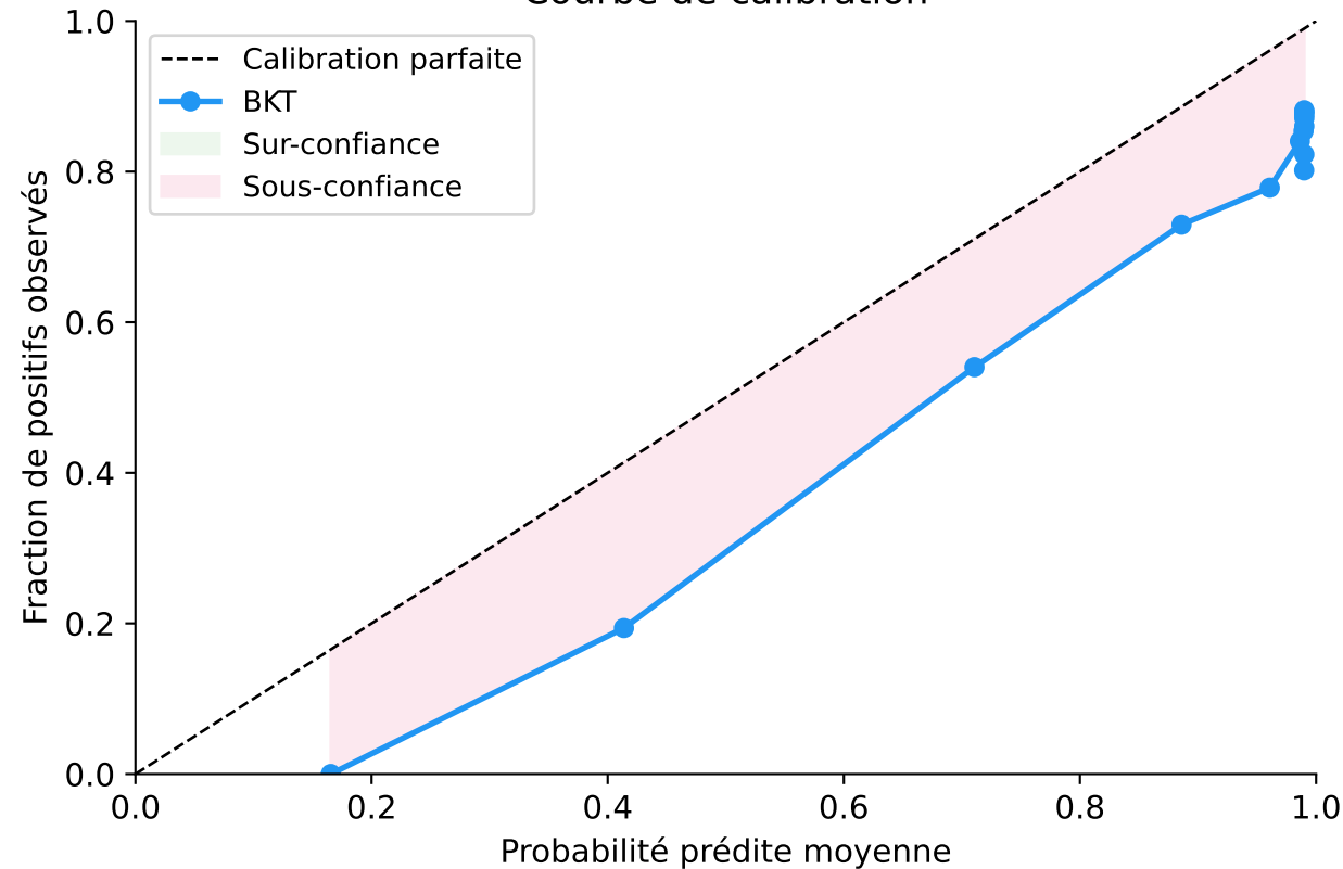
Courbe de calibration
