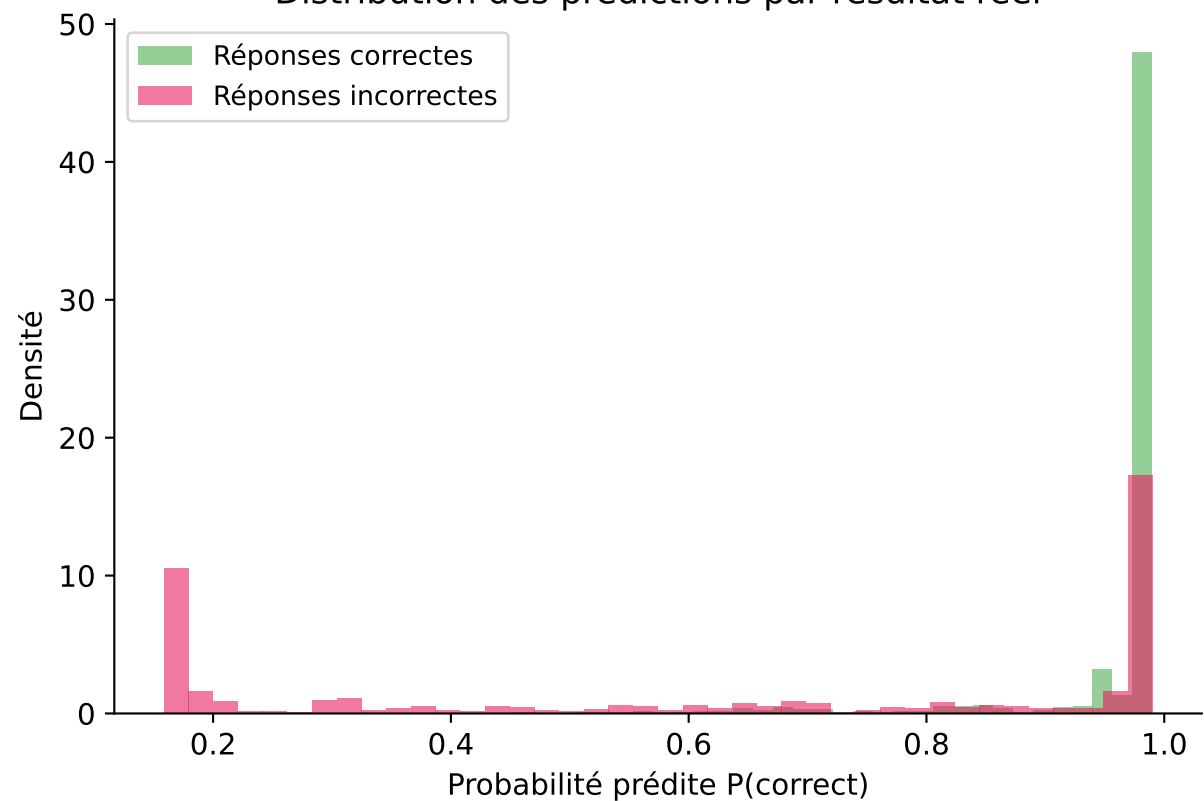
Distribution des prédictions par résultat réel
