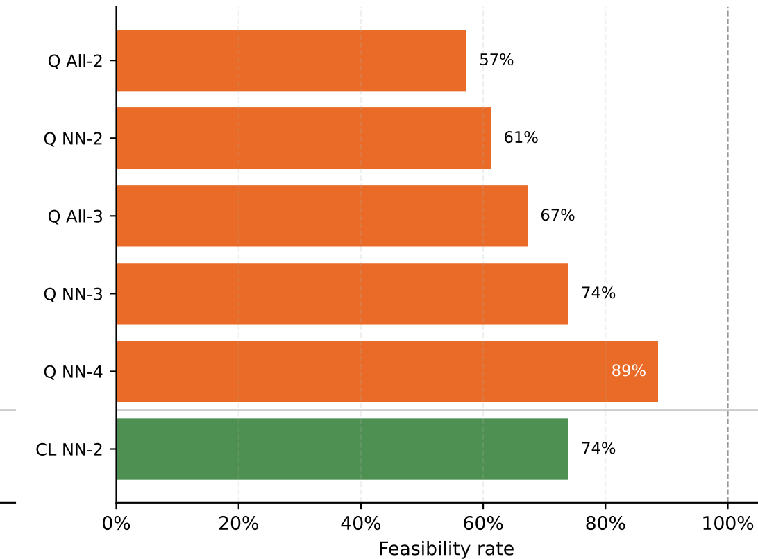
15-bus
