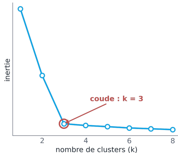
Methode du coude
