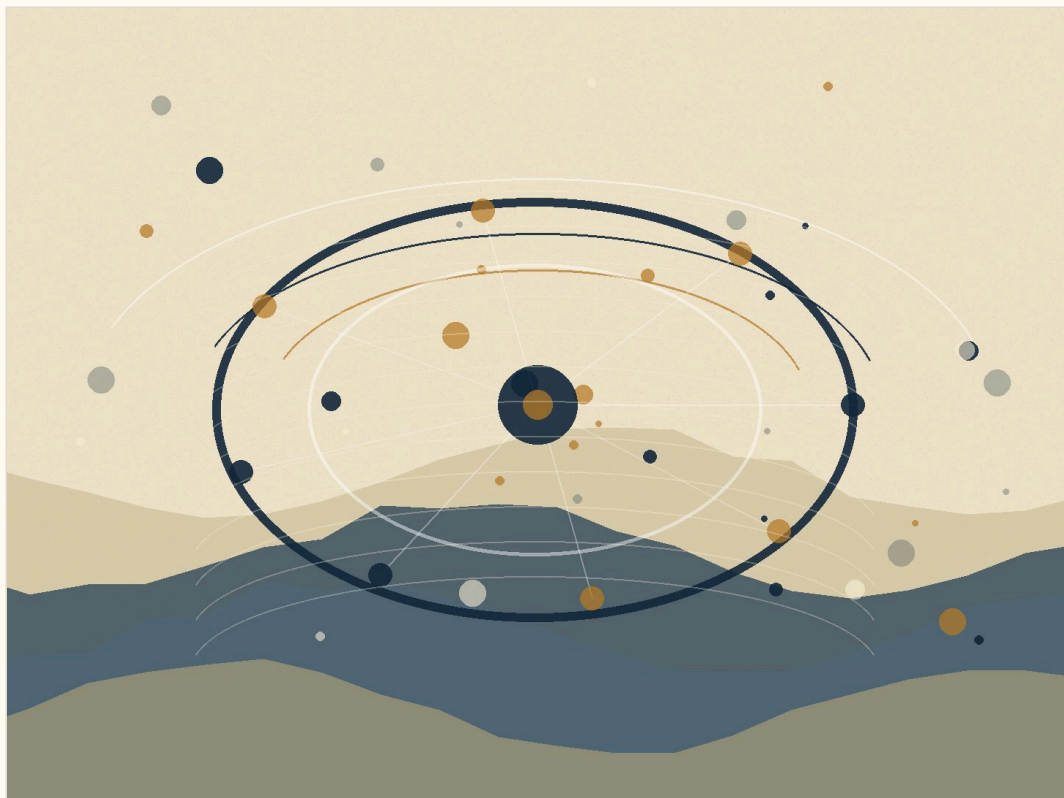
תיאור תמונה: אנרגיה, חלקיקים ואופקים כבדיקה של גבולות הצורה.
