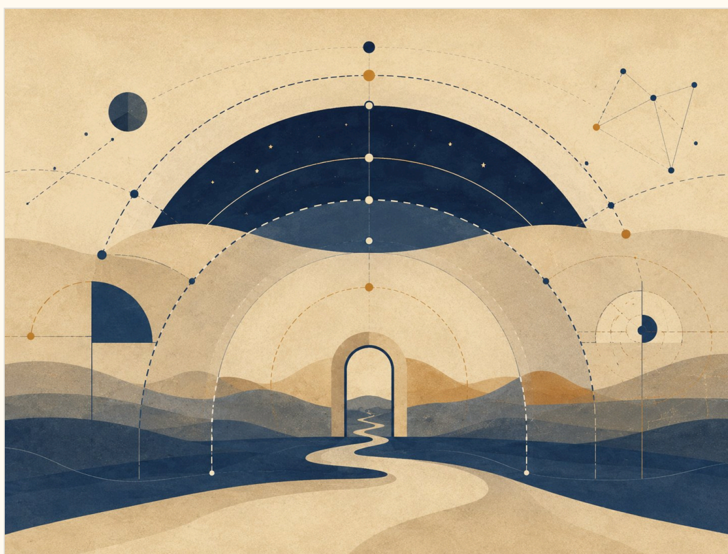
תיאור תמונה: גבול שאינו קיר בלבד, אלא אופק שמכוון את היחס בין אפשרות לצורה.
