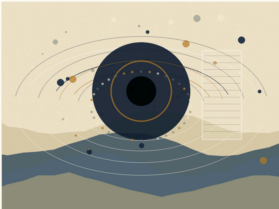
תיאור תמונה: אופק, מידע וסוף שבו מה שנעלם עדיין משאיר עקבה מבנית.
