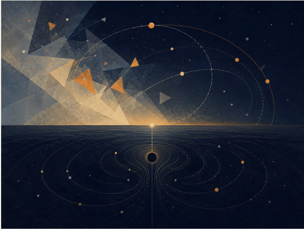
איור ו: המדומה, הווירטואלי והאופק במודל הלוגי.
