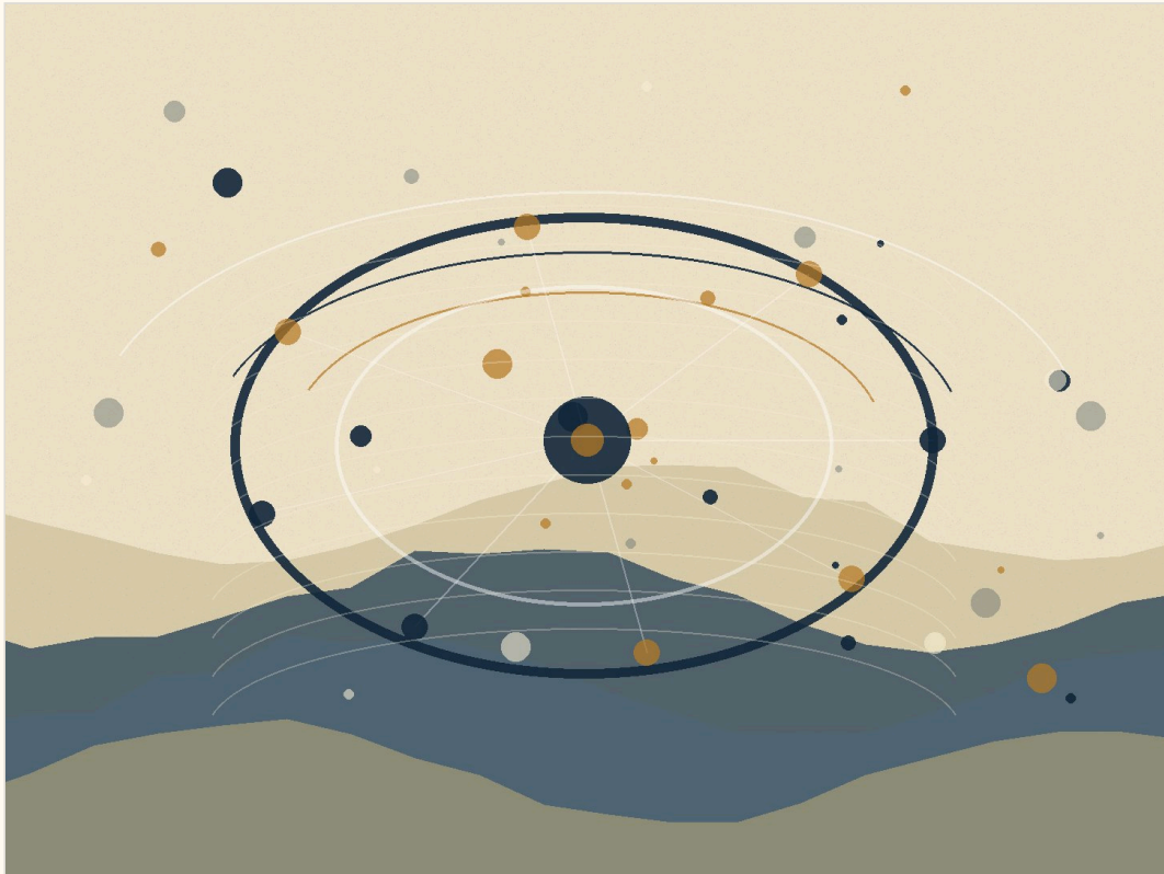
תיאור תמונה: אנרגיה, חלקיקים ואופקים כבידוק של גבולות הצורה.
