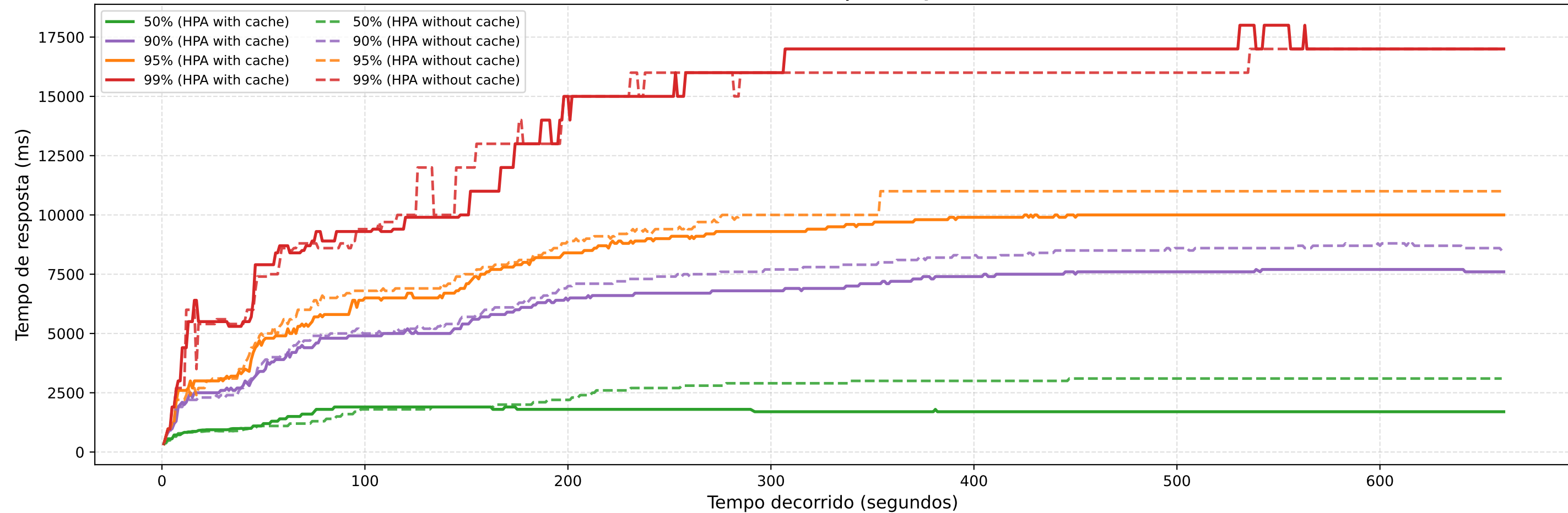
Latência (Sólido = HPA with cache | Tracejado = HPA without cache)
