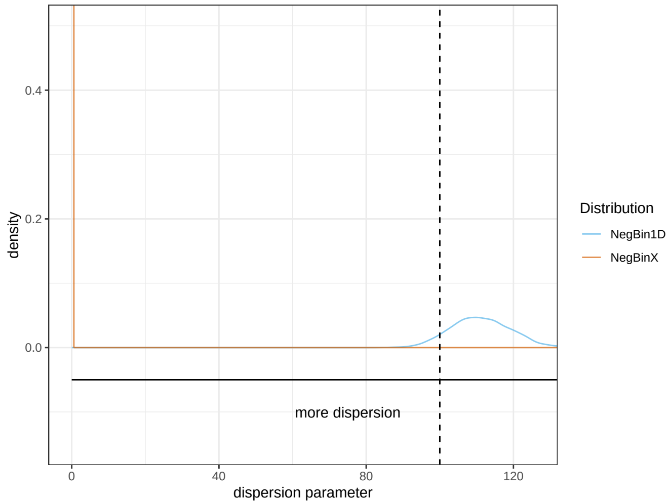
Dispersion parameter asymptotic distribution
