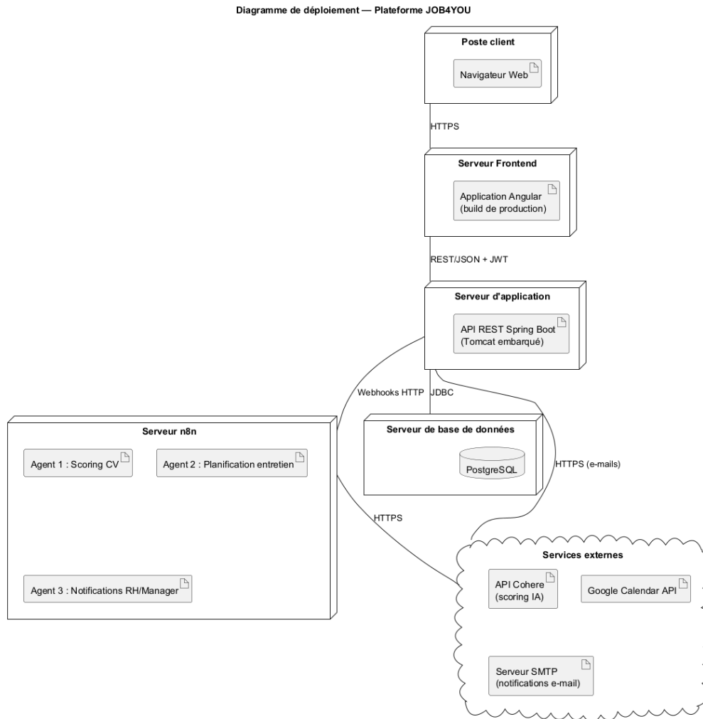
Figure 3.7 : Diagramme de déploiement de la plateforme JOB4YOU
