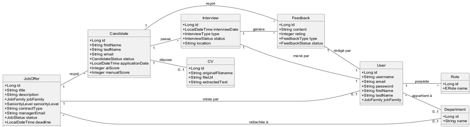
Figure 3.2 : Diagramme de classes global
