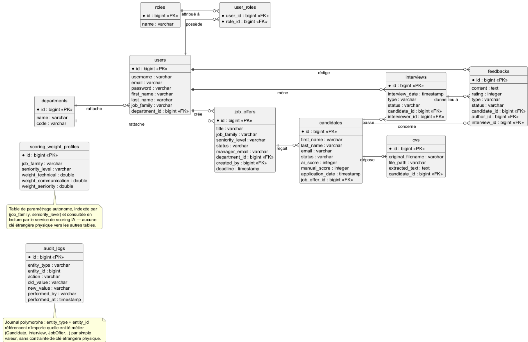
Figure 3.6 : Schéma relationnel de la base de données PostgreSQL
