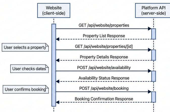
Figure 4.11: Ροή επικοινωνίας Website API.
