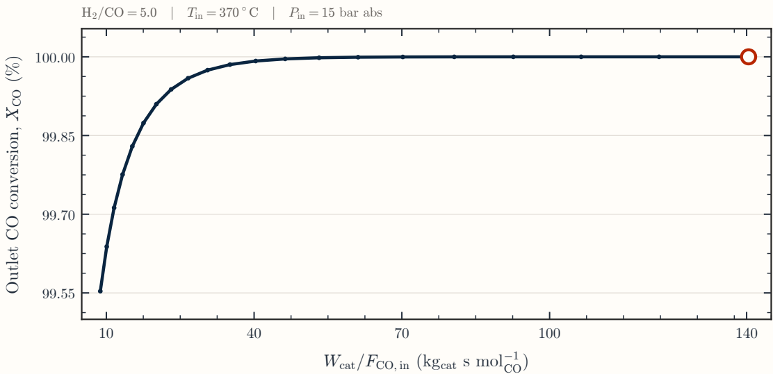
(d) Catalyst space time
