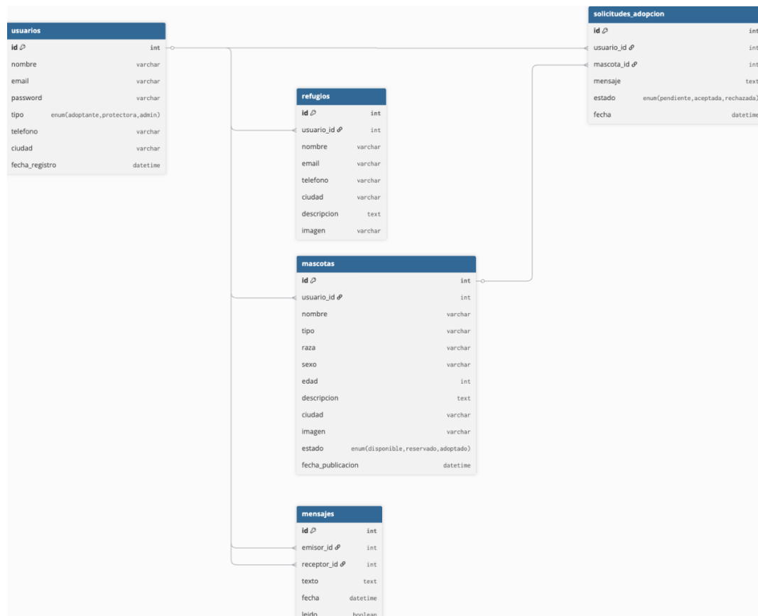
Diagrama entidad-relación
