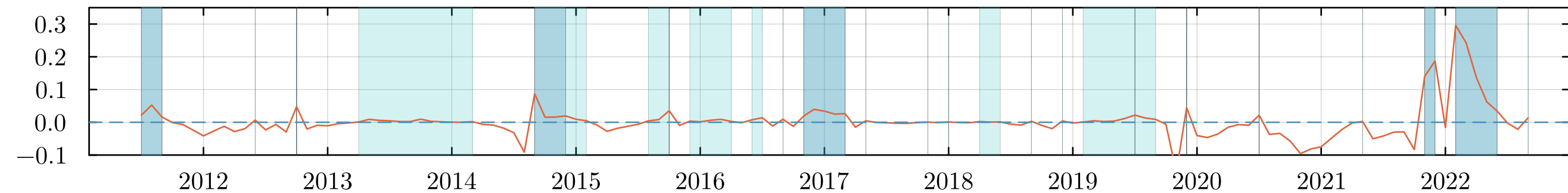
TV-EWD vs. RW
