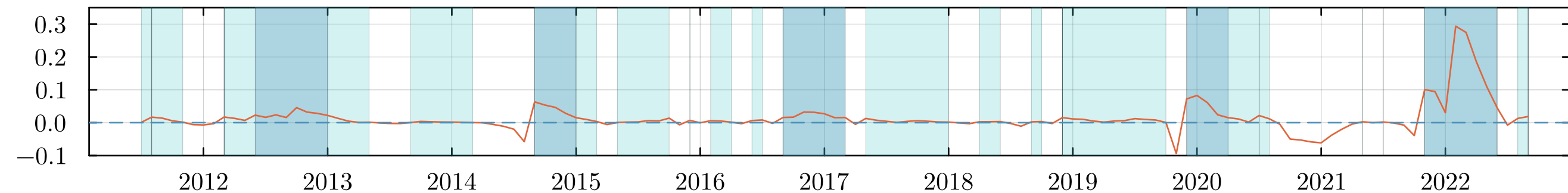
TV-AR vs. AR
