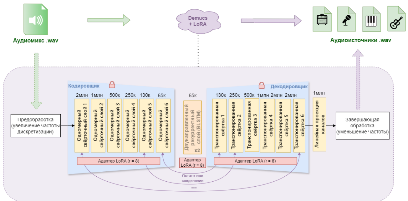
Рисунок 2.8 – Архитектурные изменения в Demucs. Авторский материал
