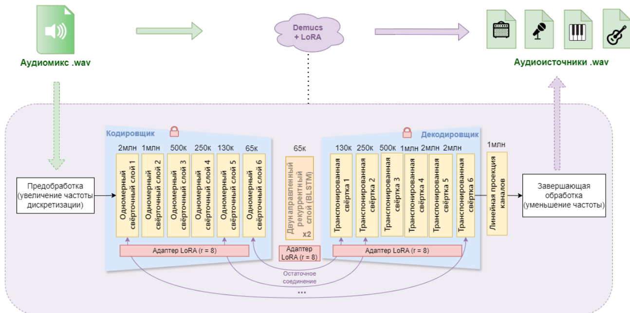
Рисунок 2.7 – Архитектурные изменения в Demucs
