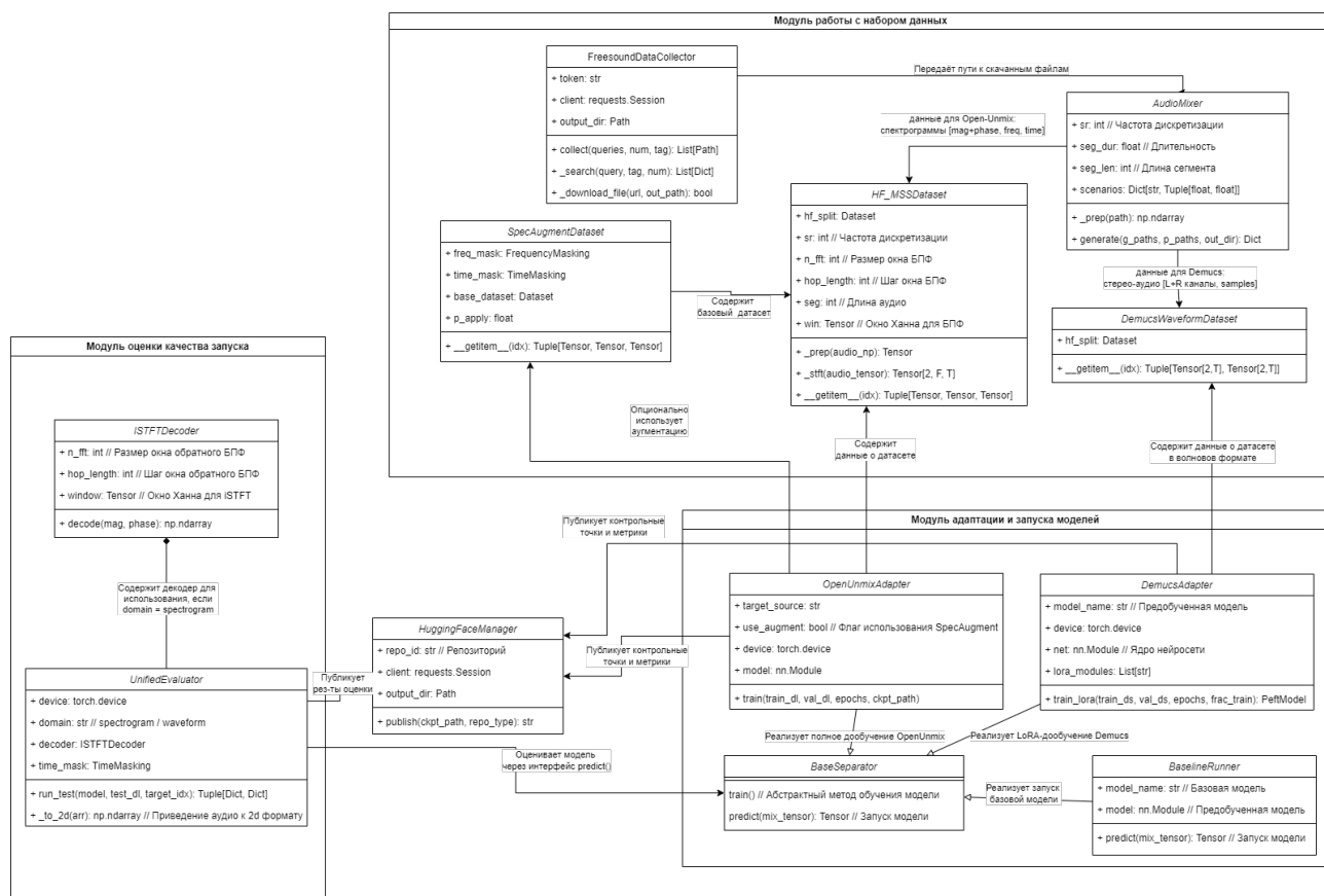
Рисунок 2.2 – Диаграмма классов
