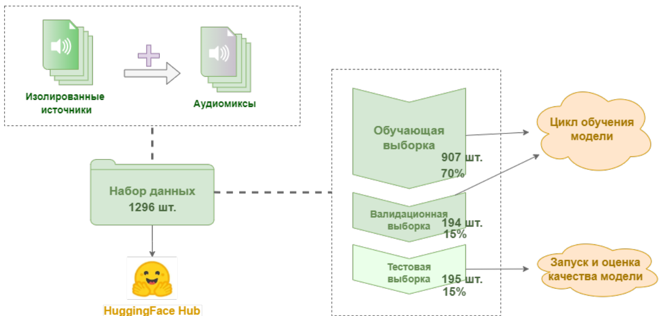
Рисунок 2.4 – Состав выборок
