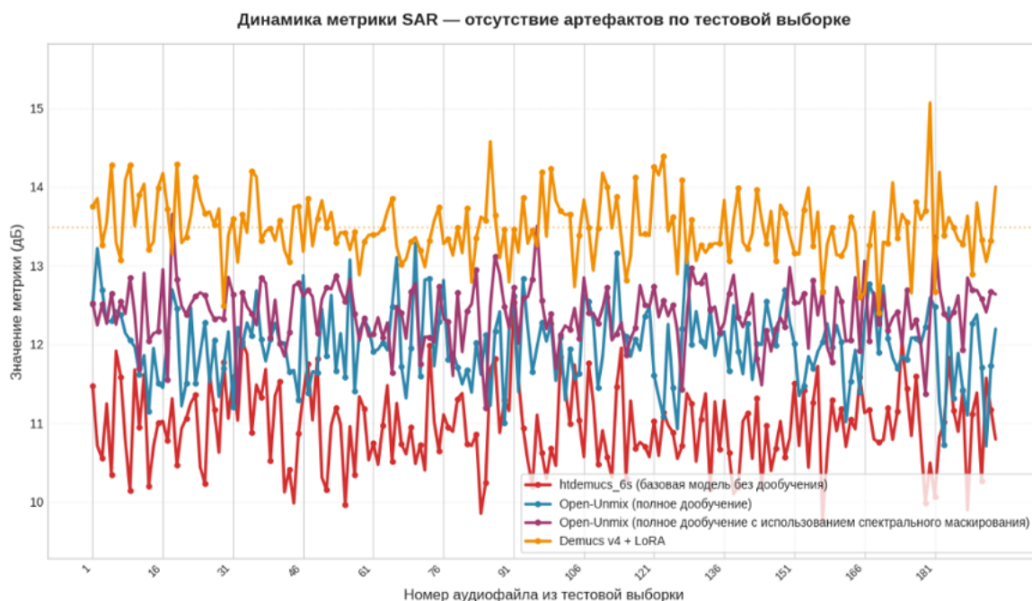
Рисунок 3.4 – Динамика метрики SAR по аудиофайлам тестовой выборки для четырёх моделей
