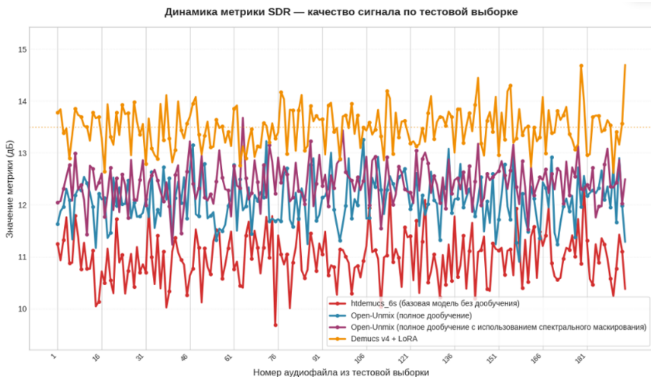
Рисунок 3.2 – Динамика метрики SDR по аудиофайлам тестовой выборки для четырёх моделей
