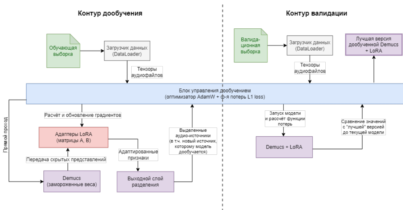
Рисунок 2.8 – Контуры дообучения модели Demucs. Авторский материал
