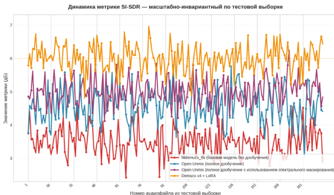
Рисунок 3.5 – Динамика метрики SI-SDR по аудиофайлам тестовой выборки для четырёх моделей
