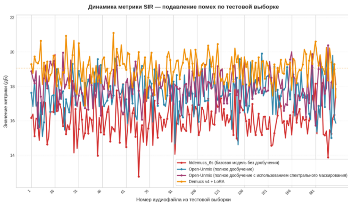
Рисунок 3.3 – Динамика метрики SIR по аудиофайлам тестовой выборки для четырёх моделей
